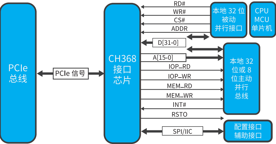
应用框图 \ Block Diagram
