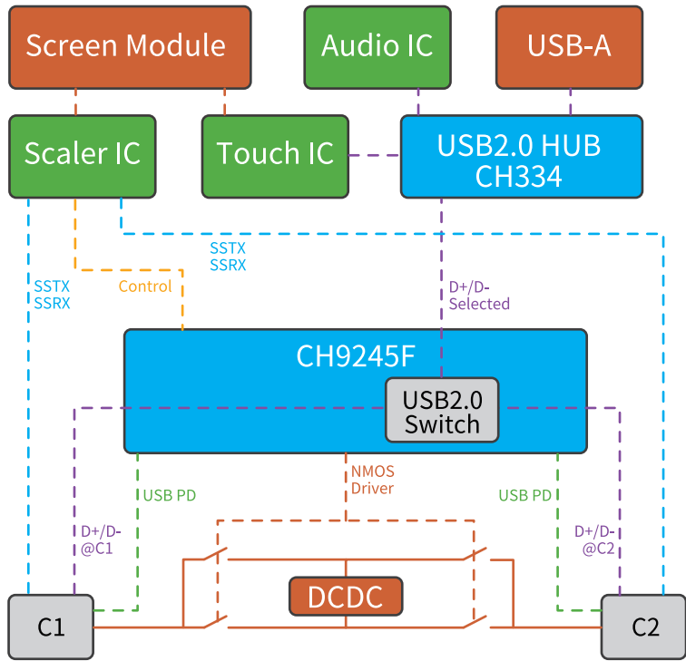
应用框图 \ Block Diagram
