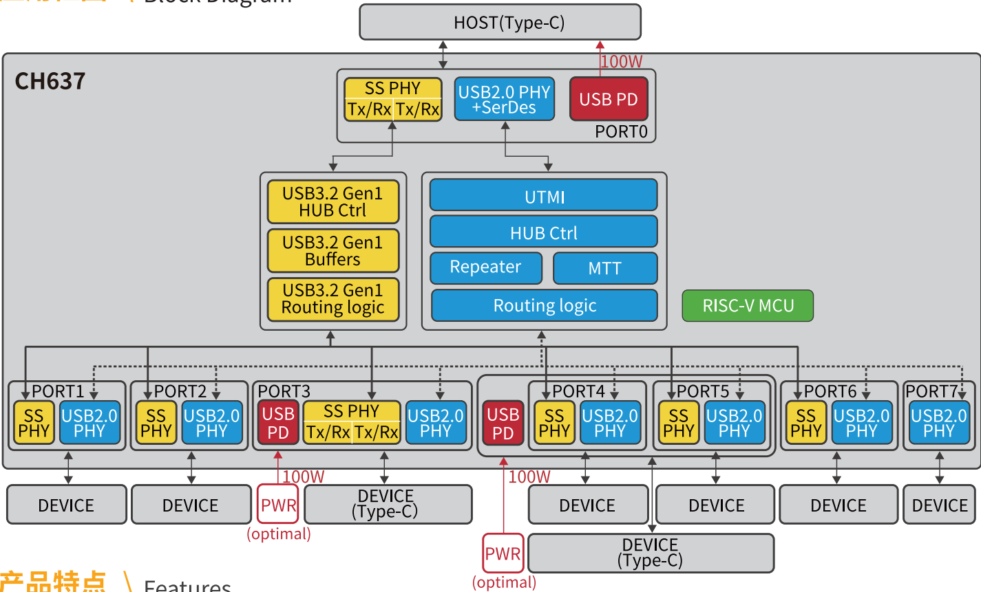
应用框图 \ Block Diagram
