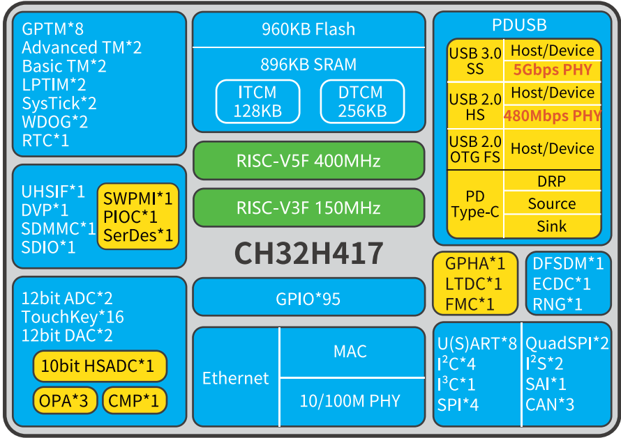
应用框图 \ Block Diagram
