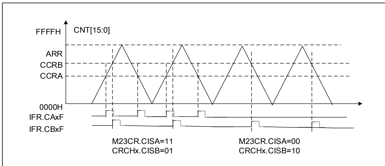
图 14-46 中断示意图
