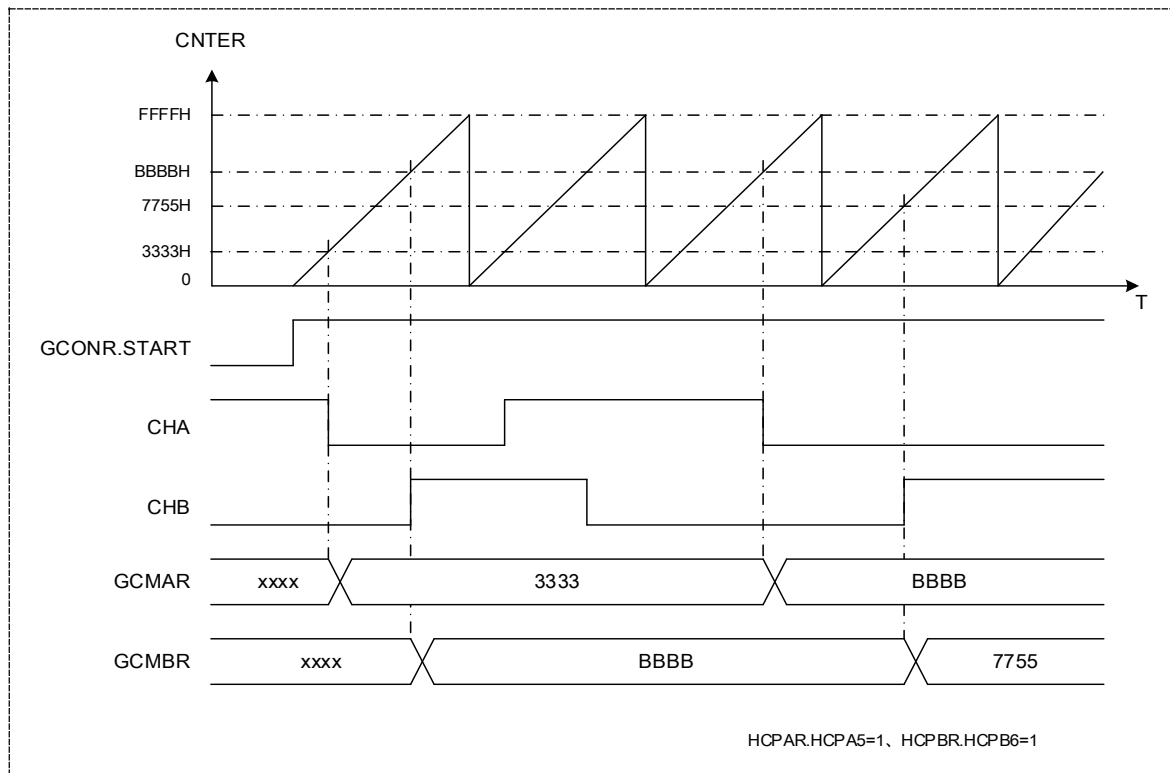
图 17-5 捕获输入动作
