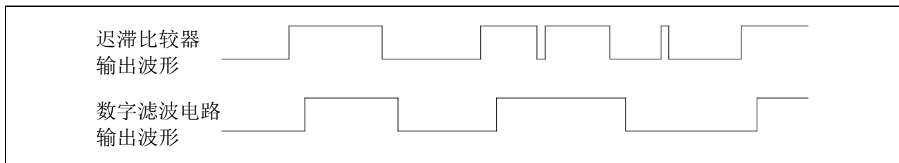
图 29-3 LVD 滤波输出
