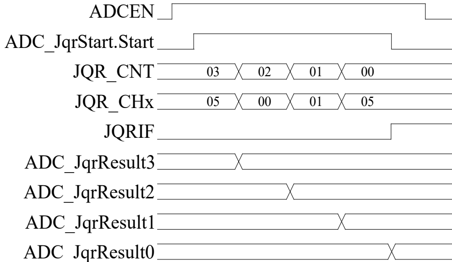
图 27-4 ADC 插队扫描转换过程示例
