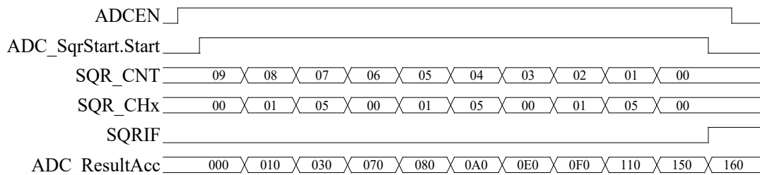
图 27-6 ADC 连续转换累加过程示例
