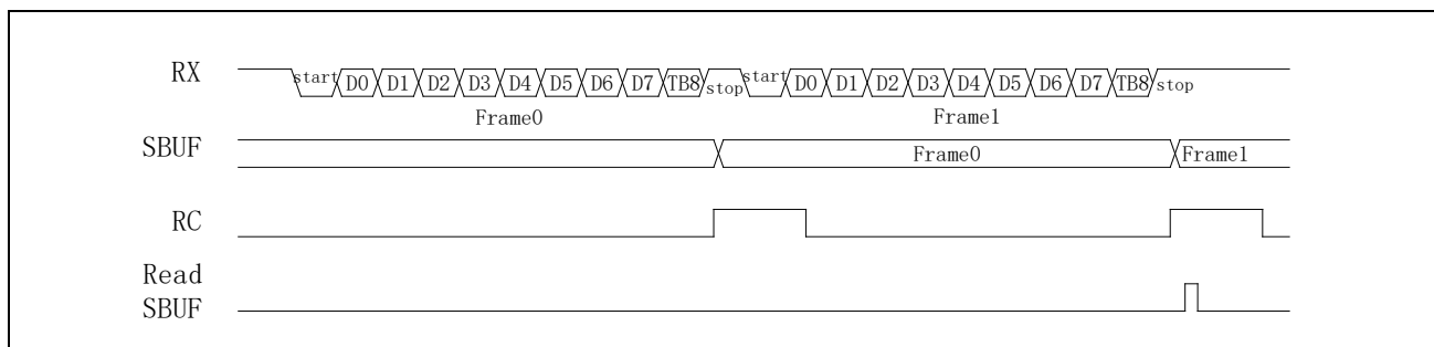
图 22-13 接收缓存
