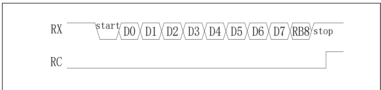
图 21-9 Mode3 接收数据
