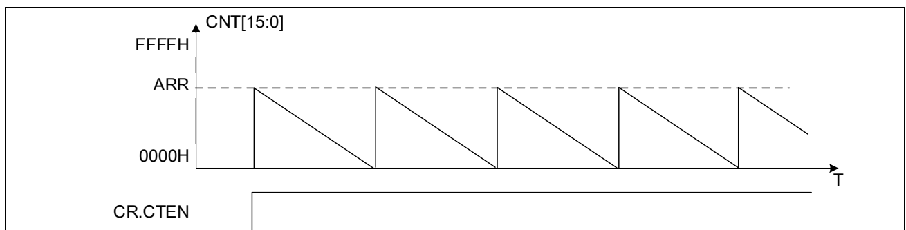
图 14-20 边沿对齐计数器波形( DIR =1)
