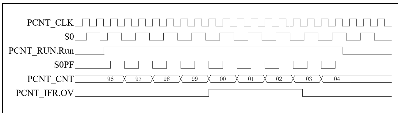
图 20-2 单通道脉冲计数模式加计数波形
