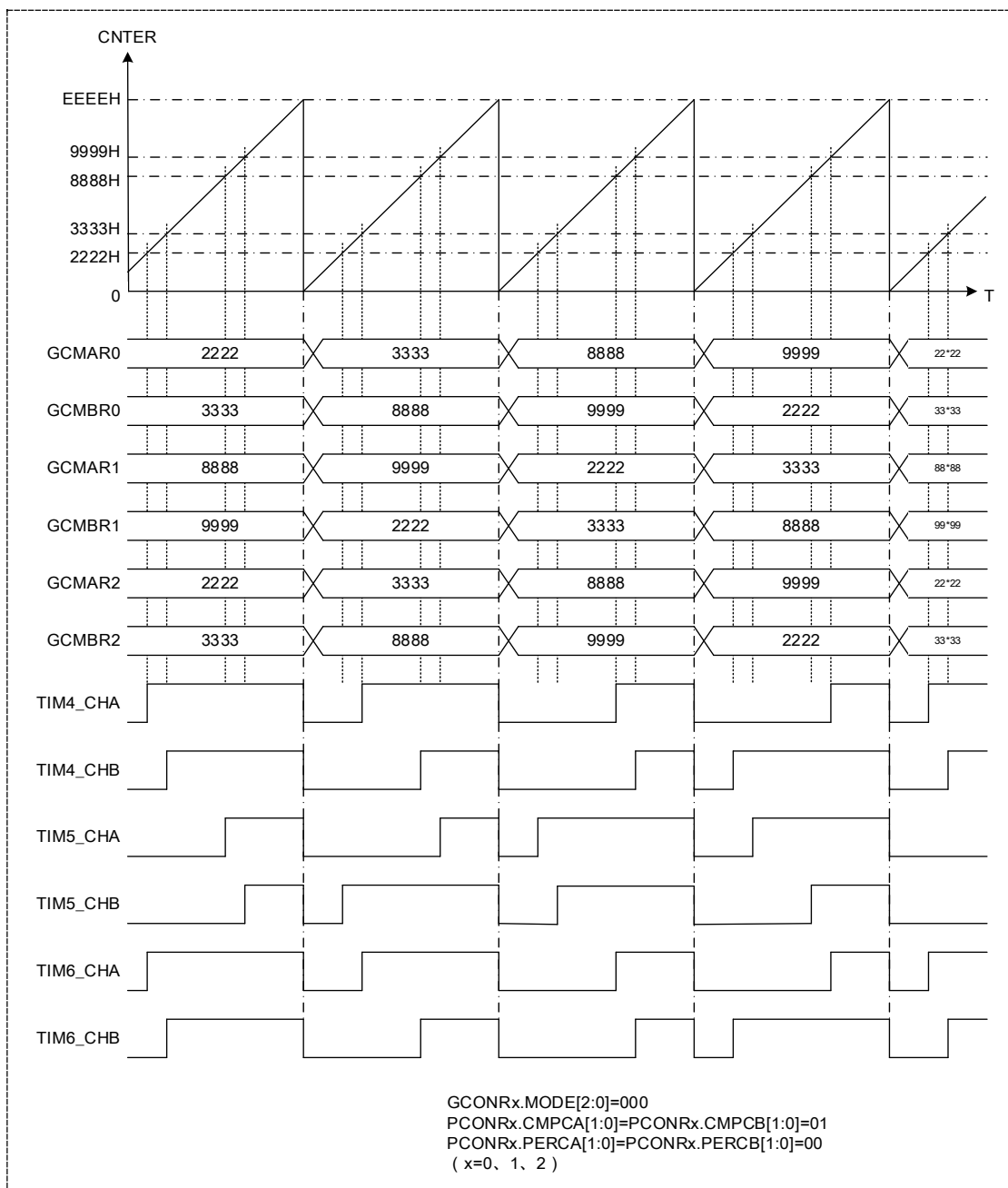
图 17-14 6 相 PWM 波
