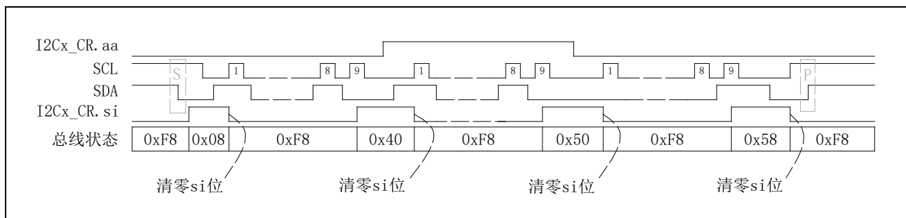
图 7-9 主接收模式数据同步图
