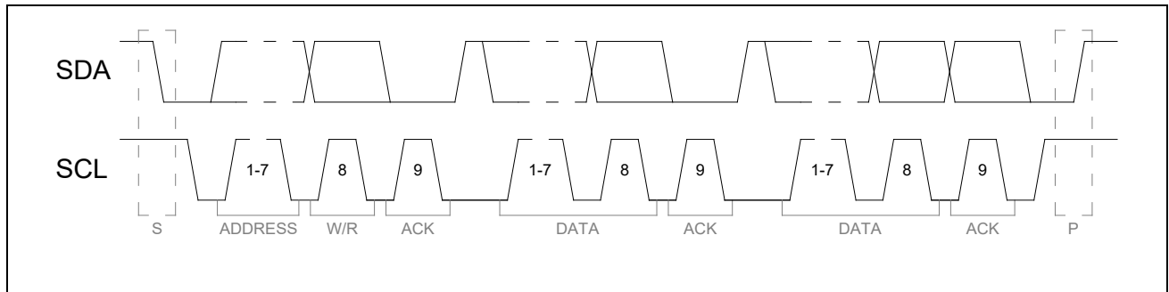
图 7-1 I2C 传输协议
