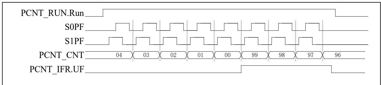
图 20-7 双通道正交脉冲计数模式减计数波形
