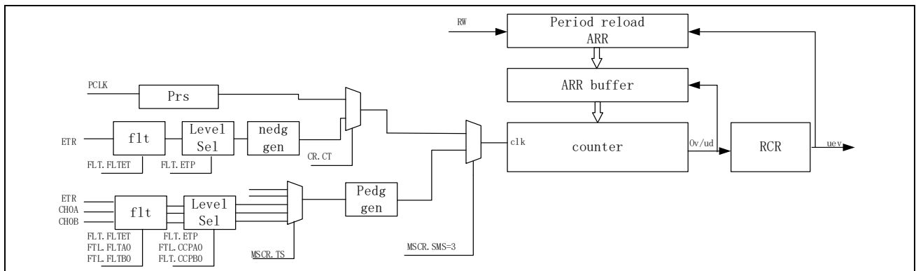
图 14-14 计数器框图
