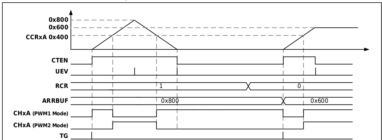
图 14-43 三角波模式单脉冲计数
