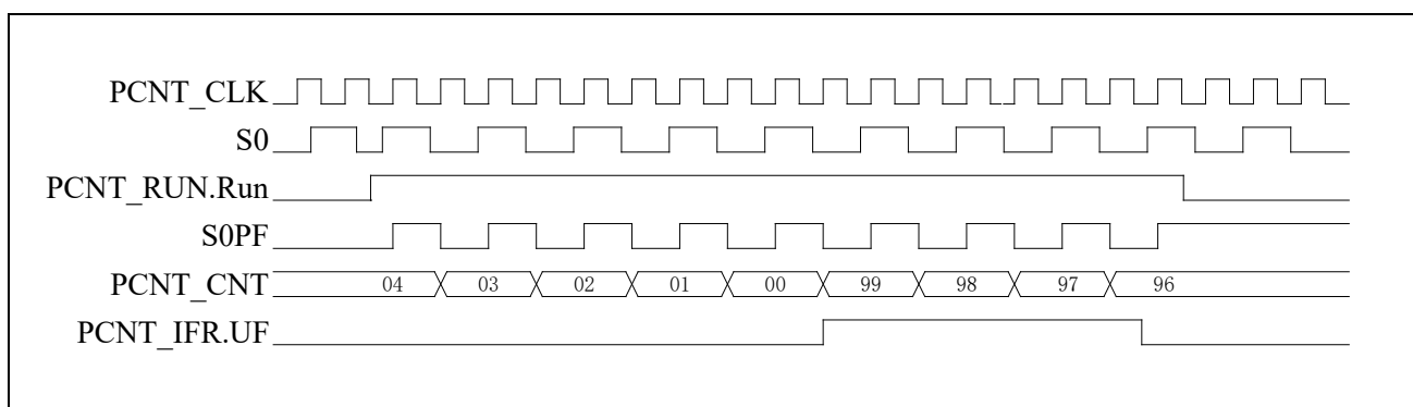
图 20-3 单通道脉冲计数模式减计数波形
