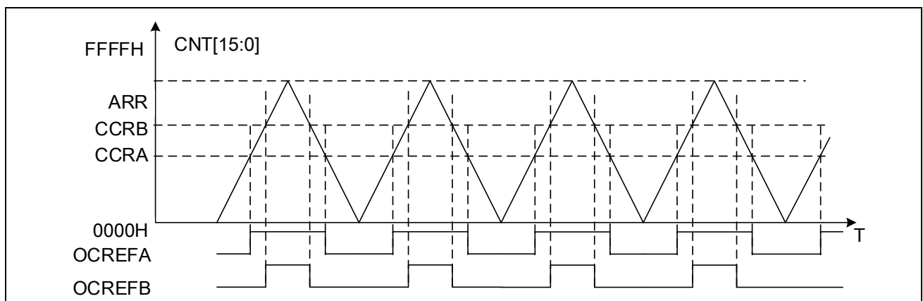
图 14-33 三角波计数单点比较 OREF 输出波形 (OCMx=111)
