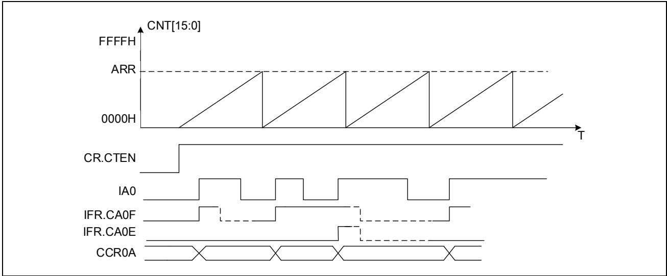
图 14-48 捕获时序图
