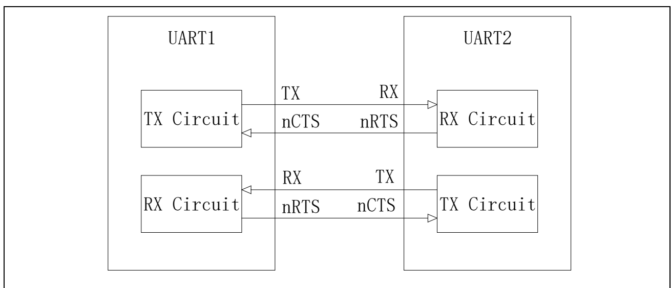
图 21-10 UART 硬件流控
