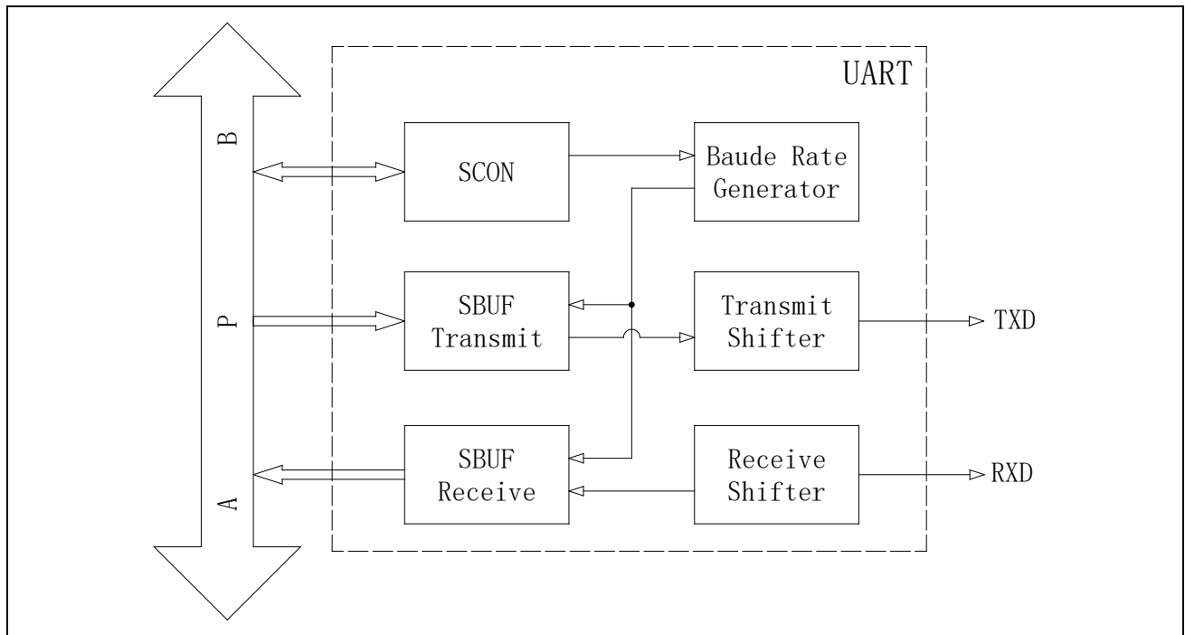
图 21-1 结构框图
