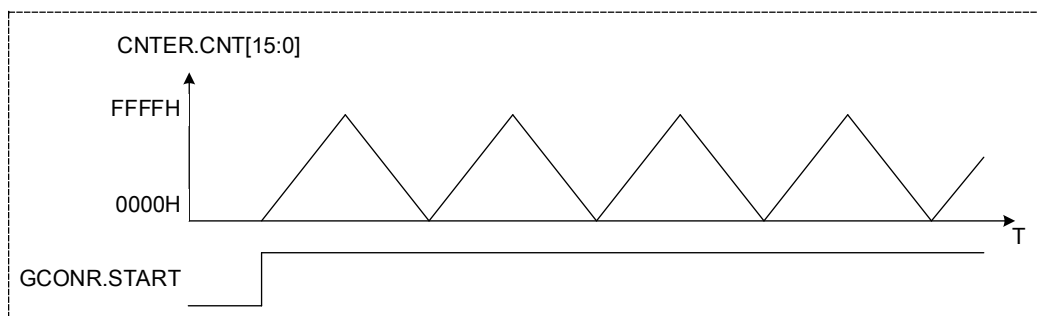
图 17-3 三角波波形
