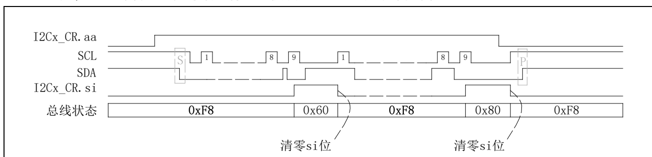
图 7-11 从接收模式数据同步图
