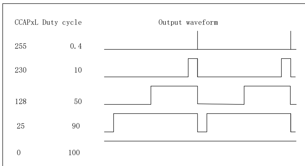
图 16-8 PCA PWM 输出波形
