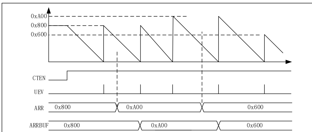
图 14-28 锯齿波模式下计数缓存使能
