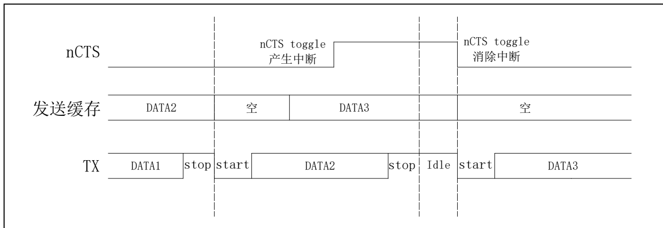
图 22-12 nCTS 硬件流控信号
