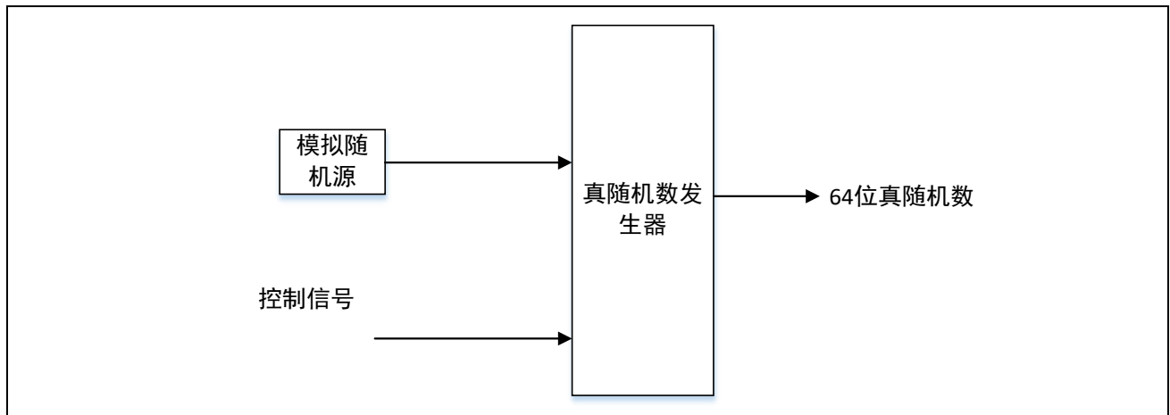
图 24-1 TRNG 数据流
