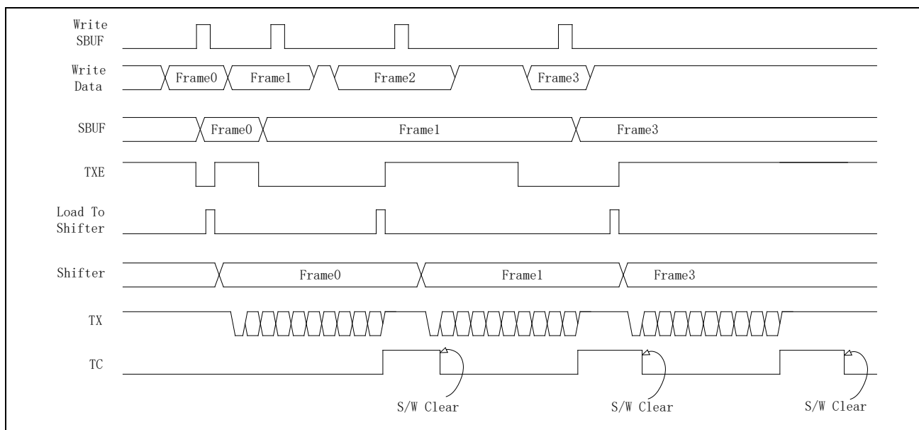
图 21-14 发送缓存
