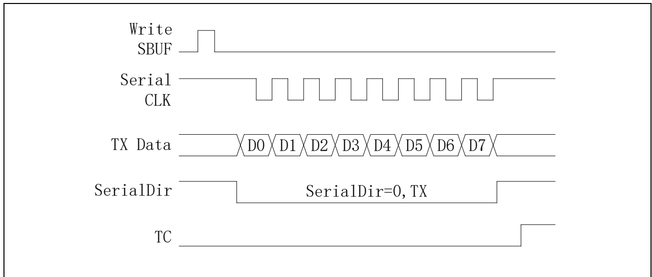
图 22-2 Mode0 发送数据
