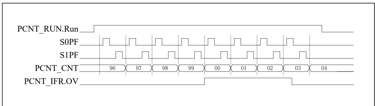
图 20-4 双通道非交脉冲计数模式加计数波形
