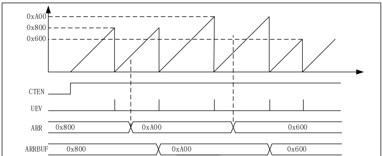
图 14-26 锯齿波模式下上计数缓存使能
