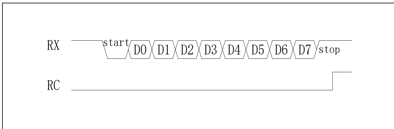
图 21-5 Mode1 接收数据
