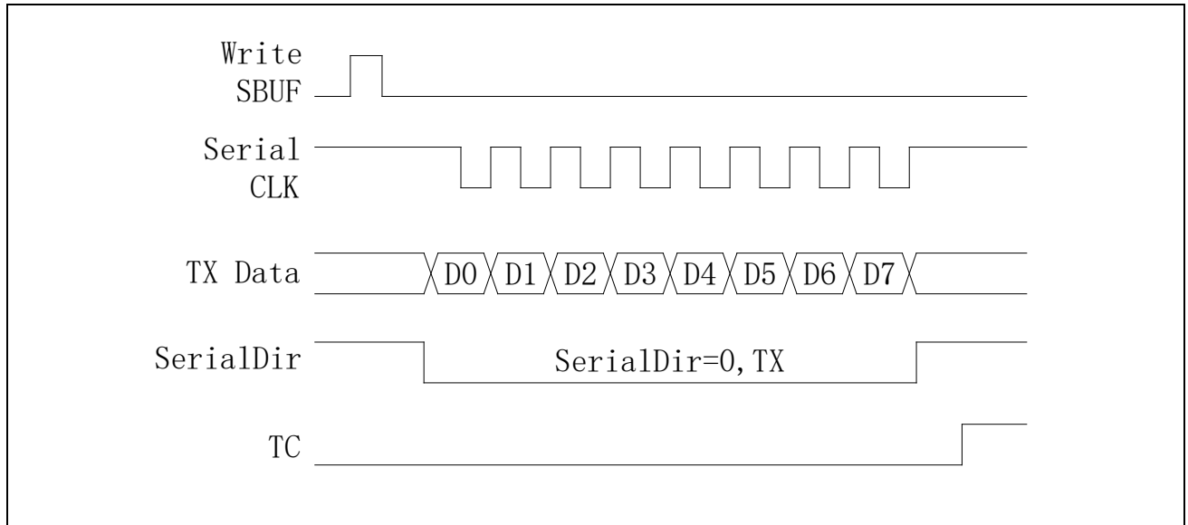
图 21-2 Mode0 发送数据
