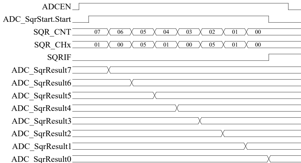
图 27-3 ADC 顺序扫描转换过程示例
