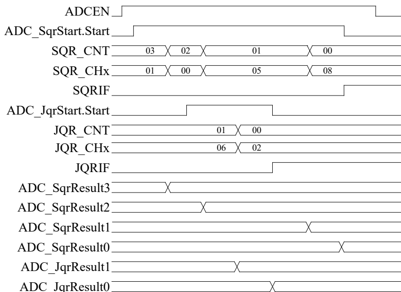
图 27-5 ADC 顺序扫描过程中进行插队扫描示例
