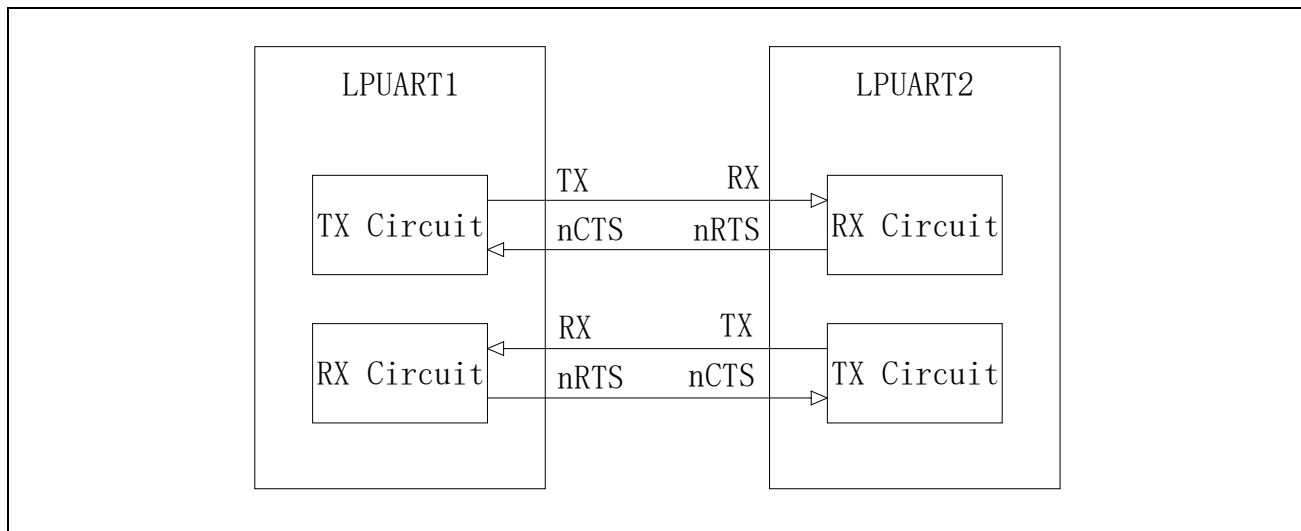
图 22-10 LPUART 硬件流控
