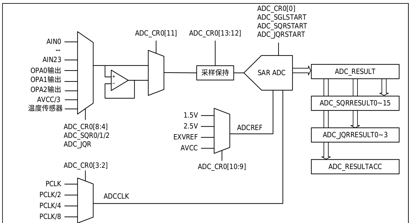
图 27-1 ADC 示意图
