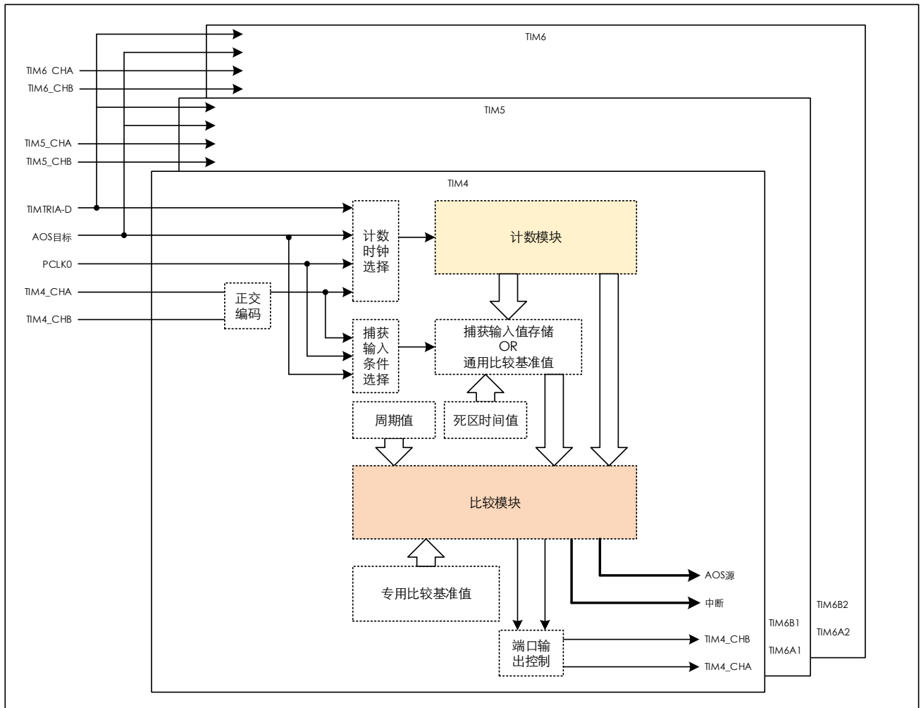
图 17-1 Advanced Timer 框图
