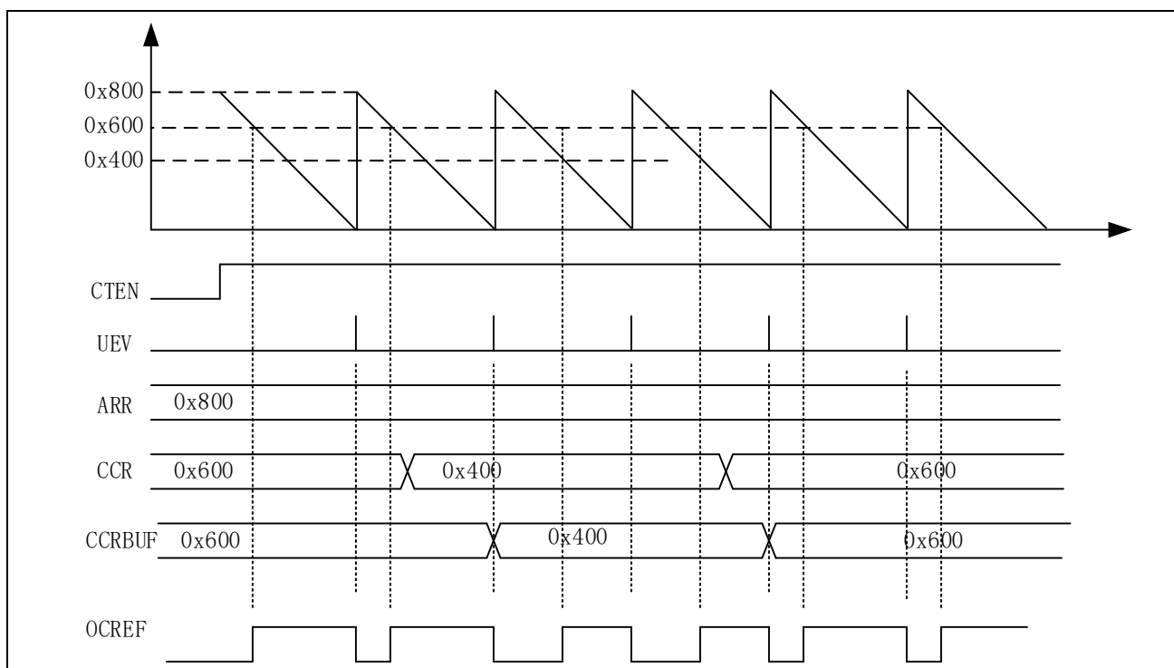
图 14-30 锯齿波模式下计数比较缓存使能
