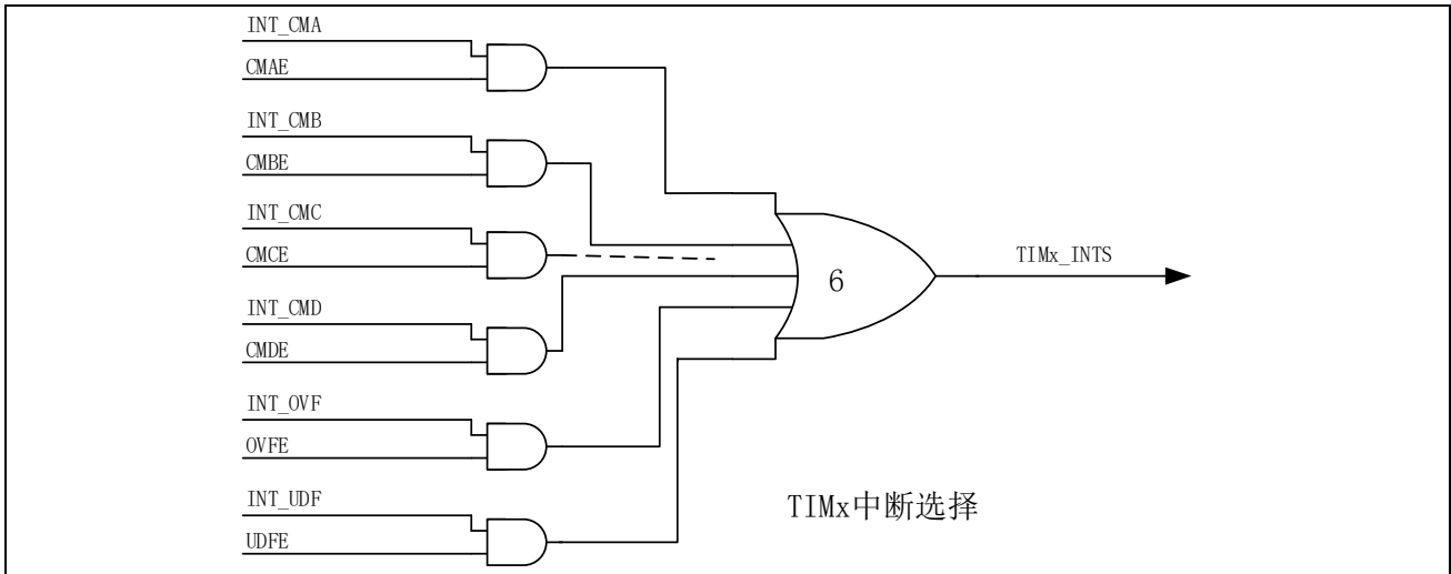
图 17-30 Timer4/5/6 中断选择
