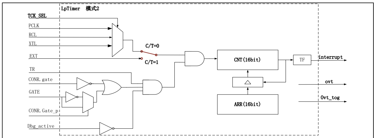
图 15-3 LPTimer 模式 2
