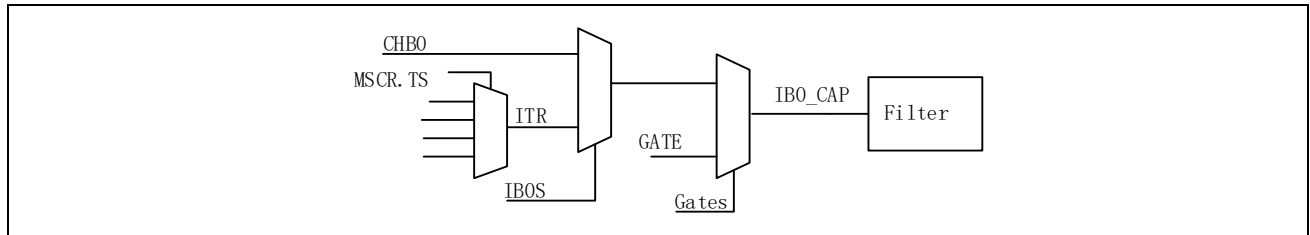
图 14-50 CHB 端口选择
