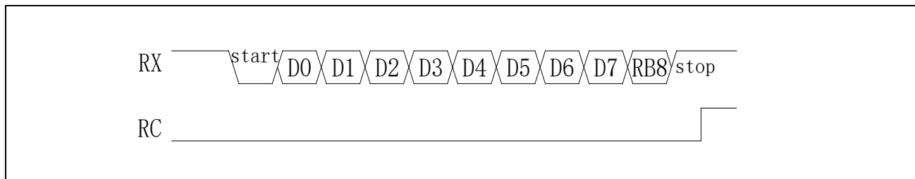
图 22-9 Mode3 接收数据
