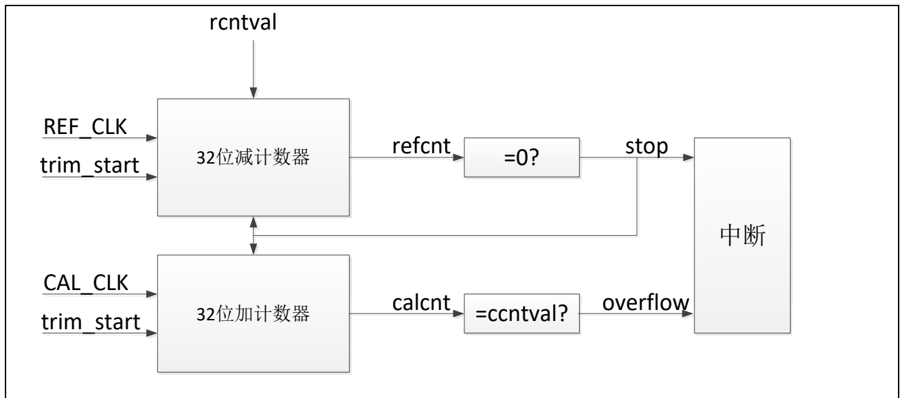
图 9-2 时钟校准模块硬件示意图
