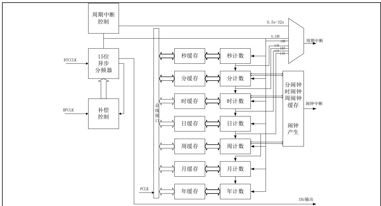
图 18-1 RTC 框图
