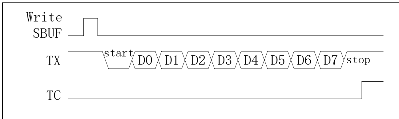
图 21-4 Mode1 发送数据
