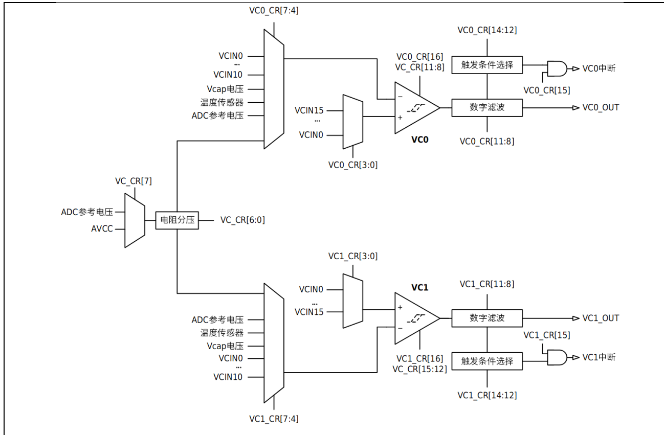
图 28-1 VC 框架图
