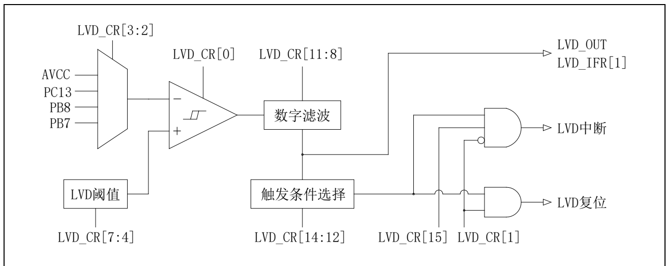
图 29-1 LVD 框图
