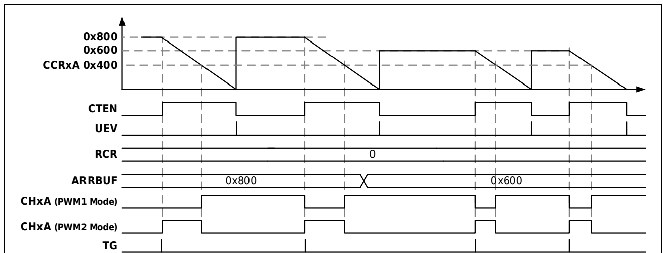
图 14-45 锯齿波下计数单脉冲模式
