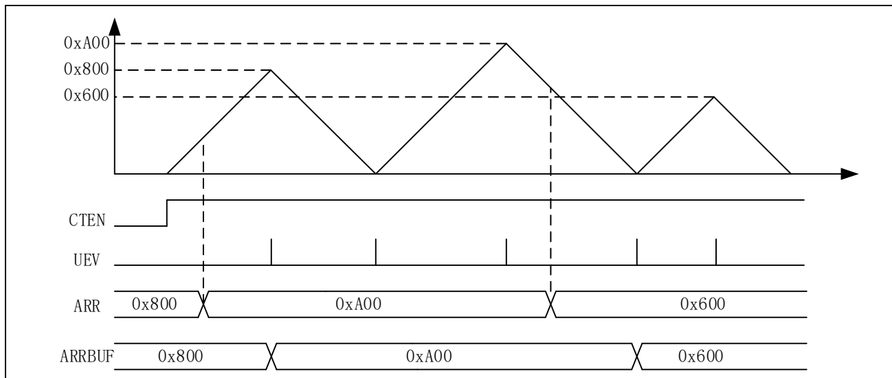
图 14-24 三角波模式下缓存使能
