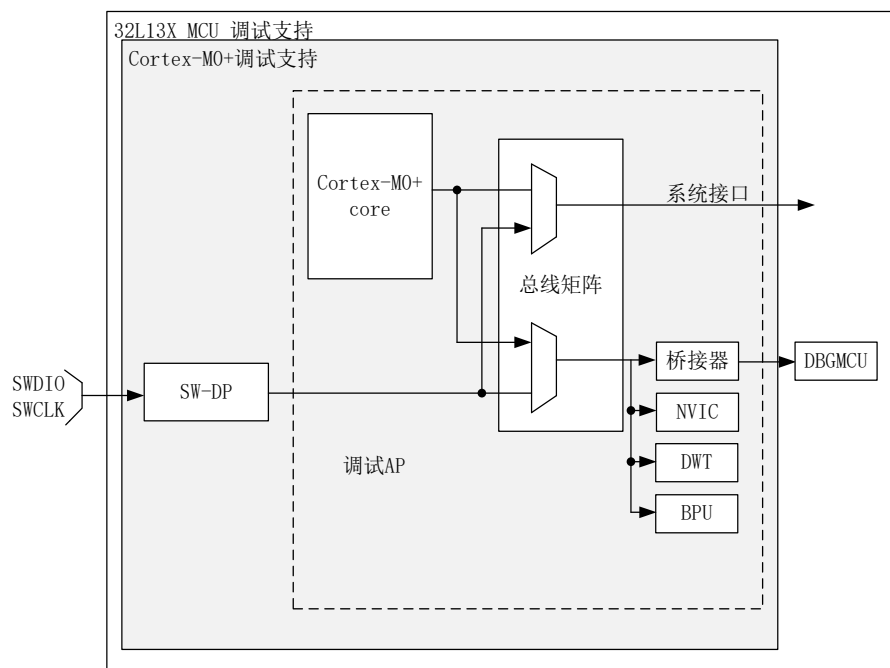
图 32-1 调试支持框图
