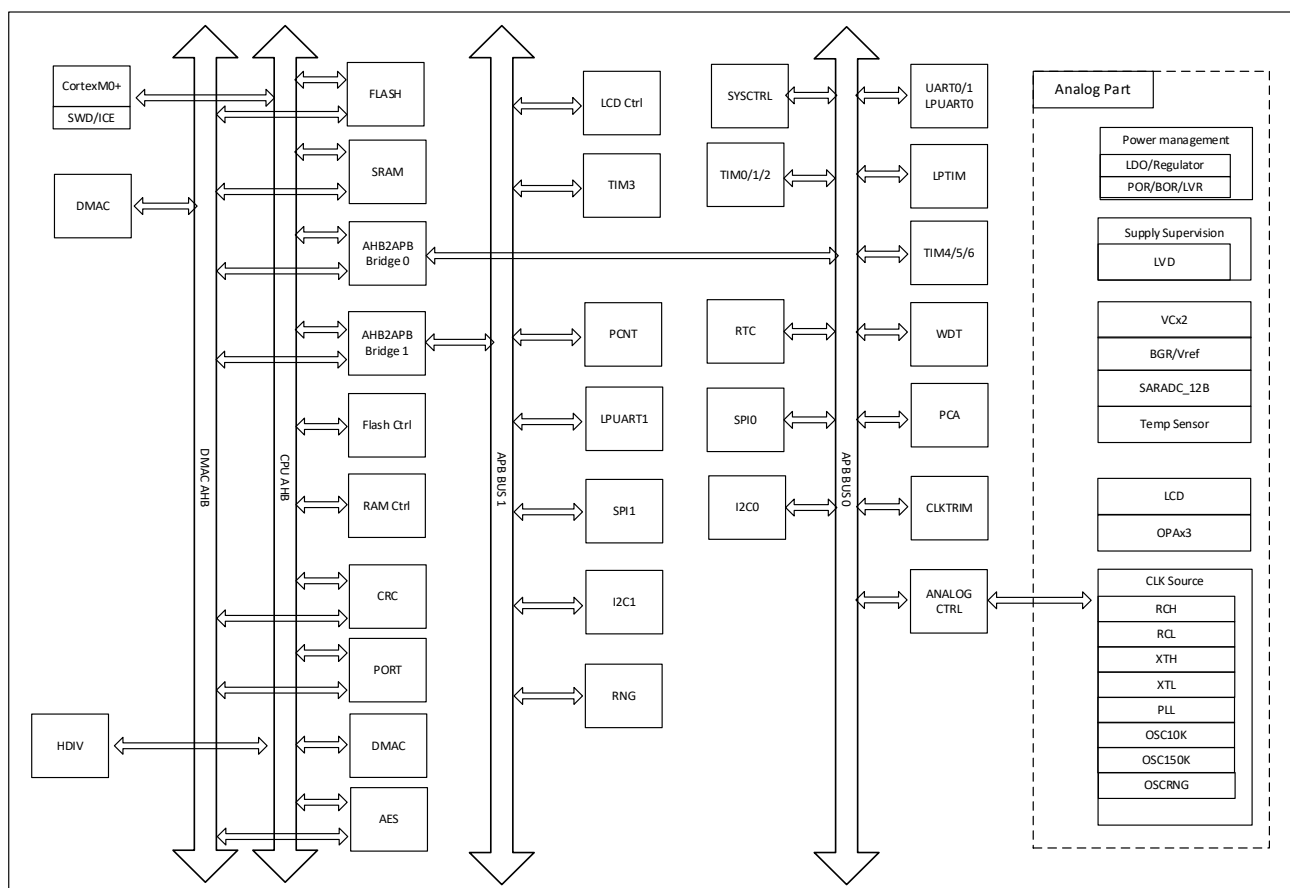
图 1-1 系统架构示意图
