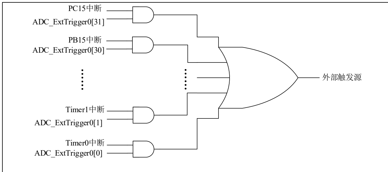
图 27-7 ADC 单次转换或顺序扫描转换外部触发源示意图
