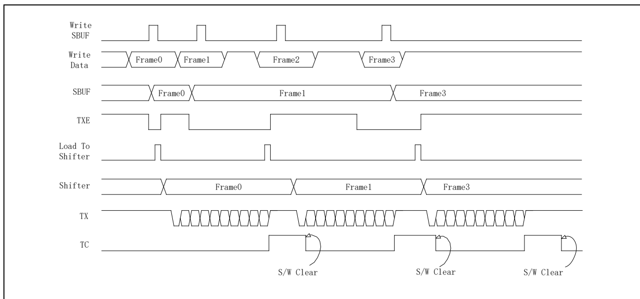
图 22-14 发送缓存
