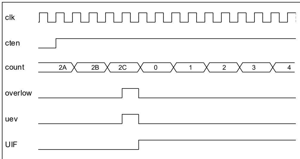
图 14-16 带预分频的上计数
