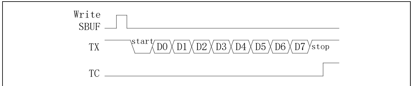
图 22-4 Mode1 发送数据
