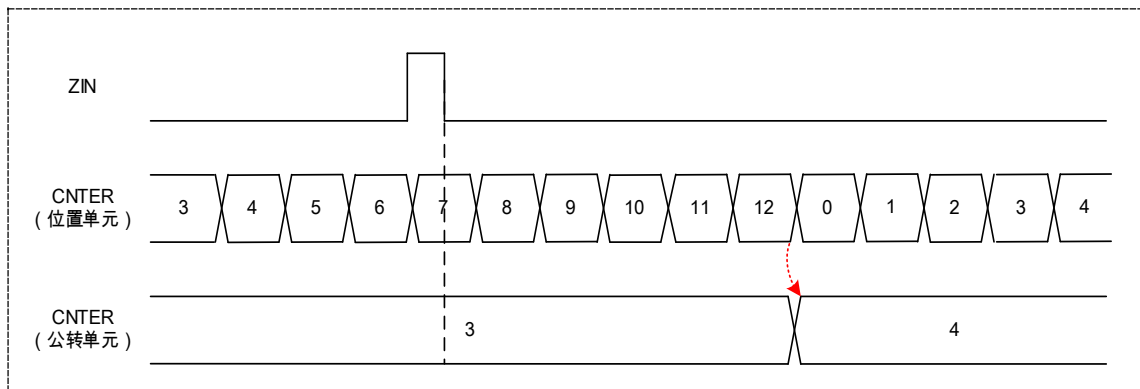
图 17-22 公转模式时位置计数器输出计数动作
