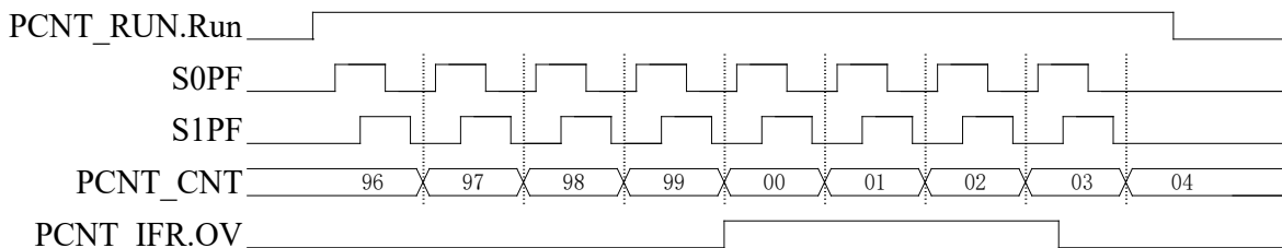
图 20-6 双通道正交脉冲计数模式加计数波形
