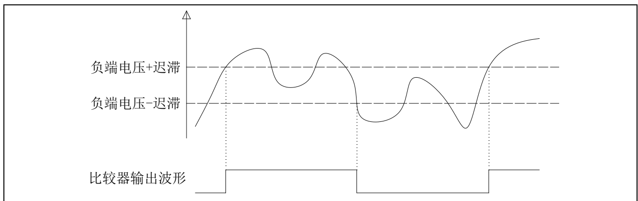
图 28-3 VC 迟滞功能
