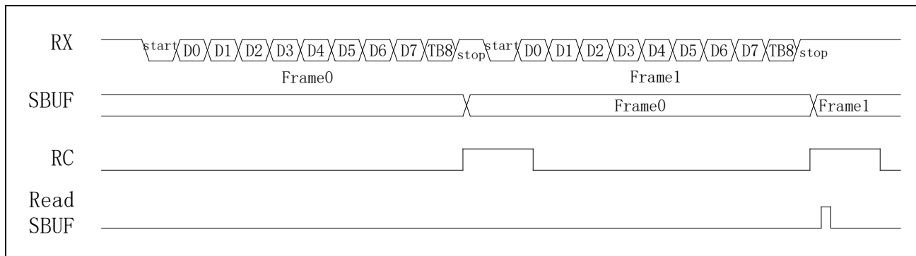
图 21-13 接收缓存
