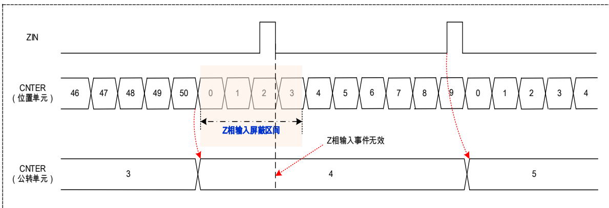
图 17-24 公转计数模式-混合计数 Z 相屏蔽动作例 1
