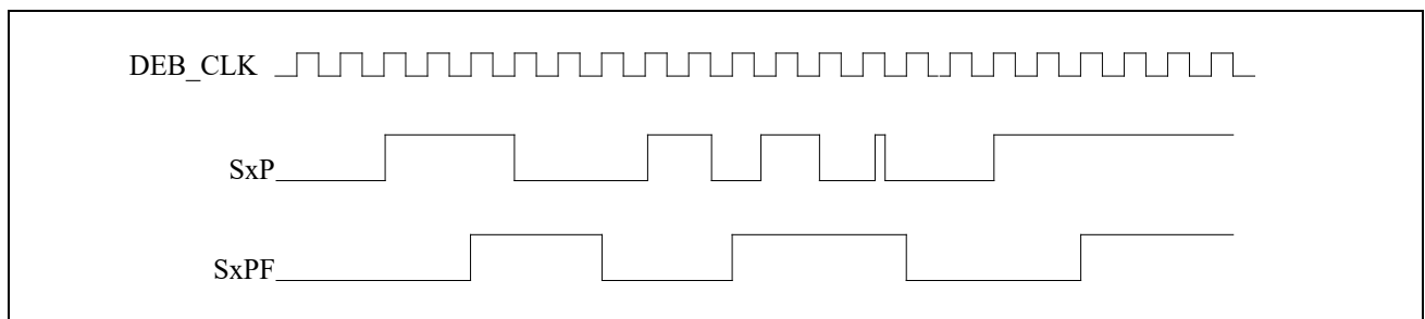
图 20-8 脉冲宽度滤波波形
