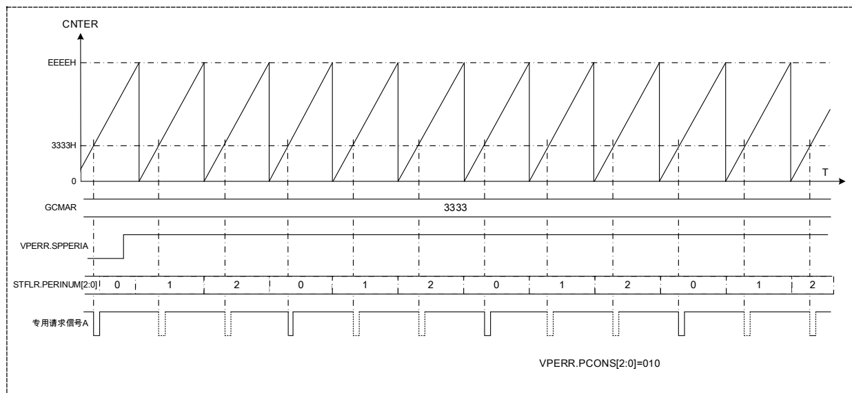
图 17-26 周期间隔有效请求信号动作
