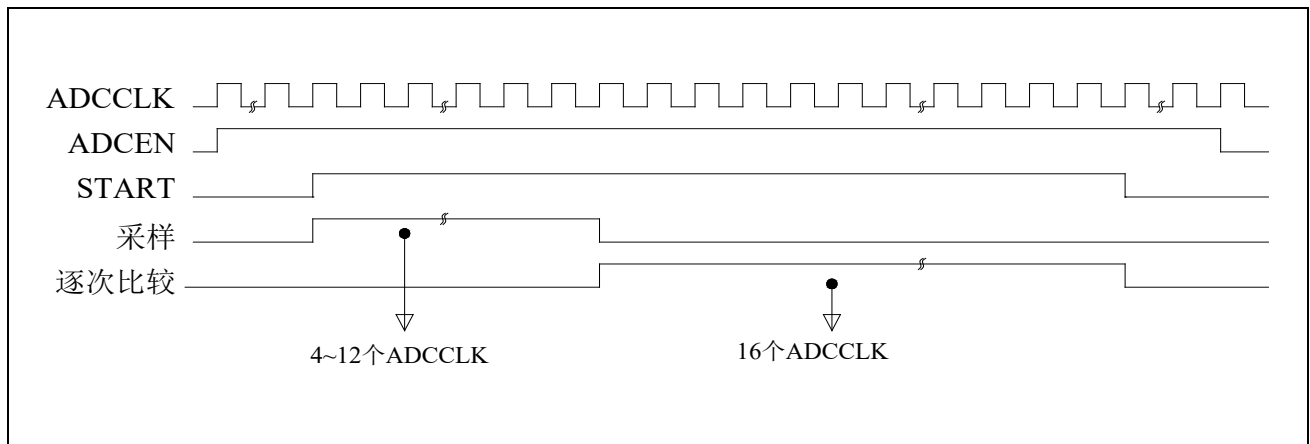
图 27-2 ADC 转换时序图
