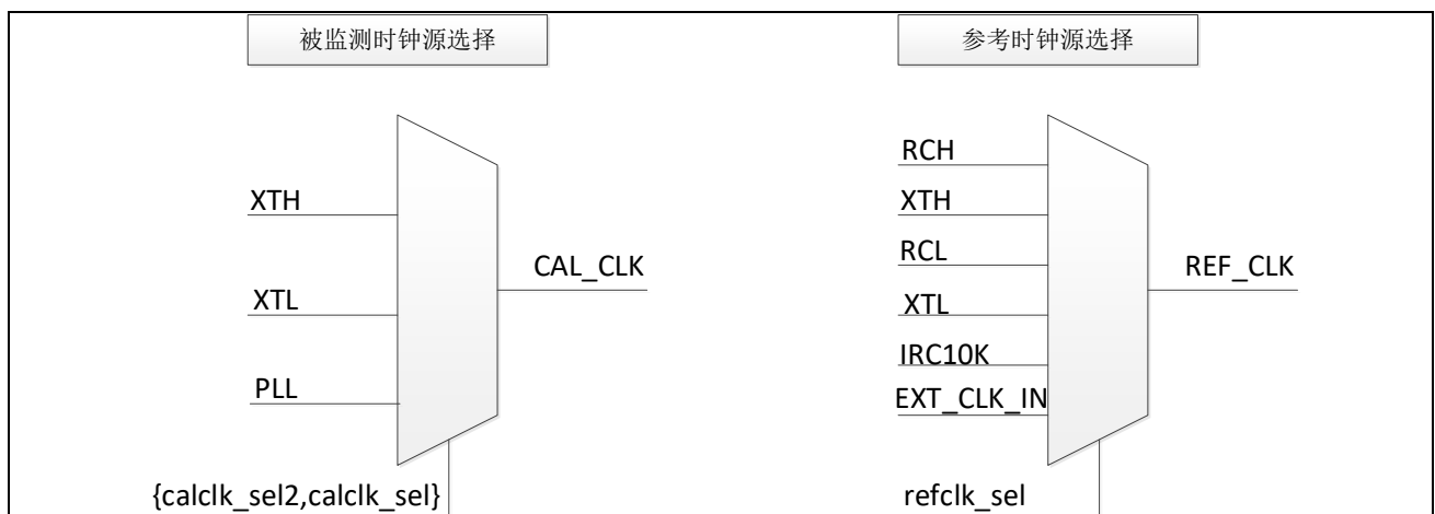
图 9-4 CLKTRIM 时钟选择
