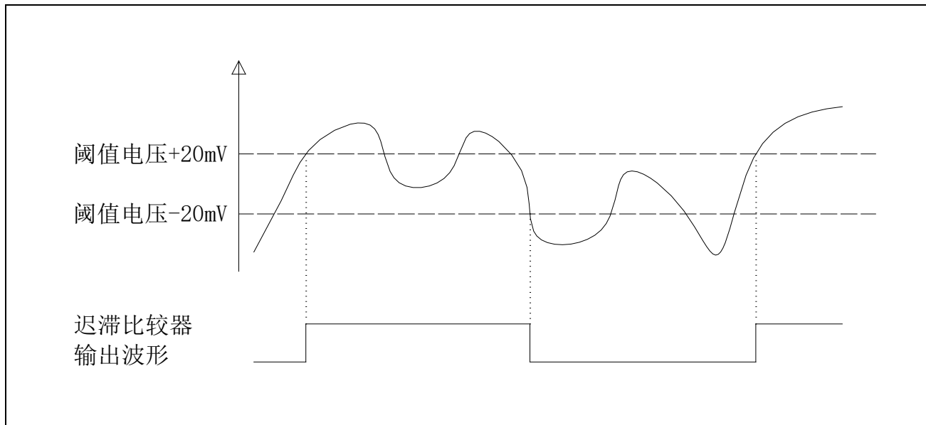
图 29-2 LVD 迟滞响应
