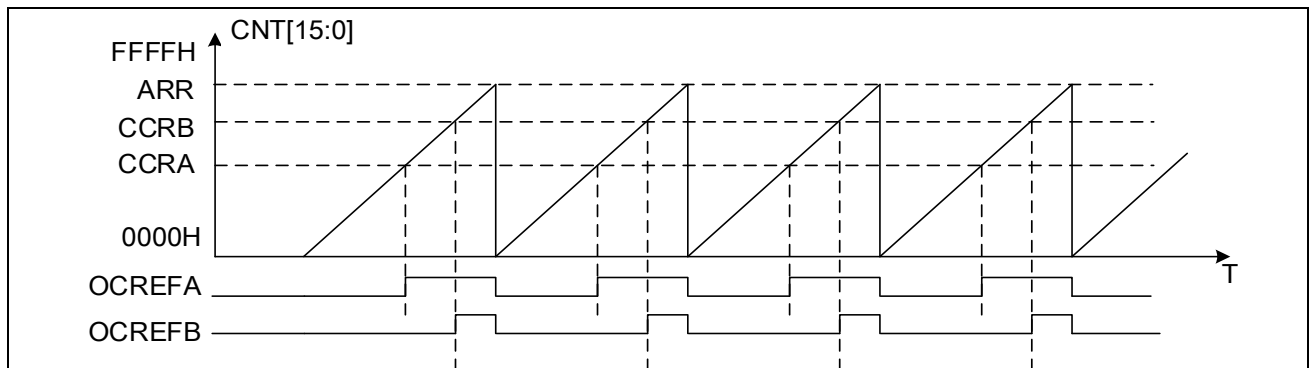
图 14-32 锯齿波计数单点比较 OREF 输出波形 (OCMx=111)
