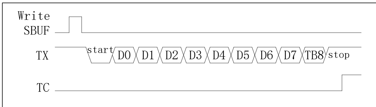
图 21-6 Mode2 发送数据
