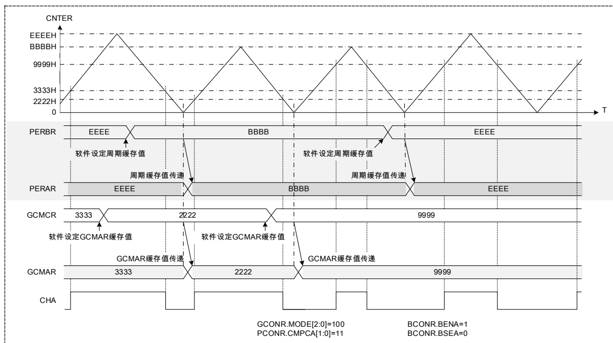
图 17-9 单缓存方式比较输出时序
