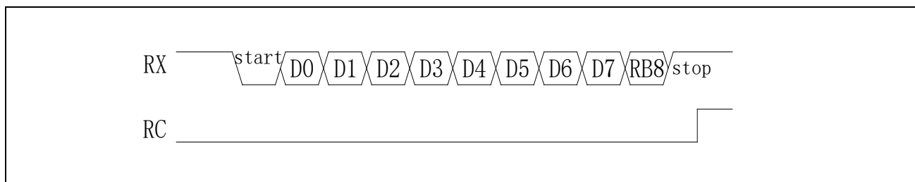
图 22-7 Mode2 接收数据
