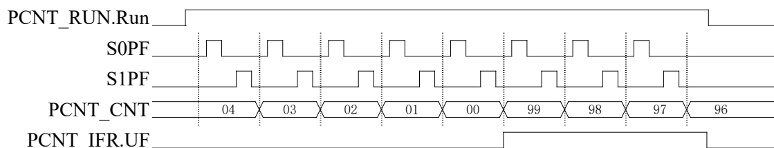
图 20-5 双通道非交脉冲计数模式减计数波形
