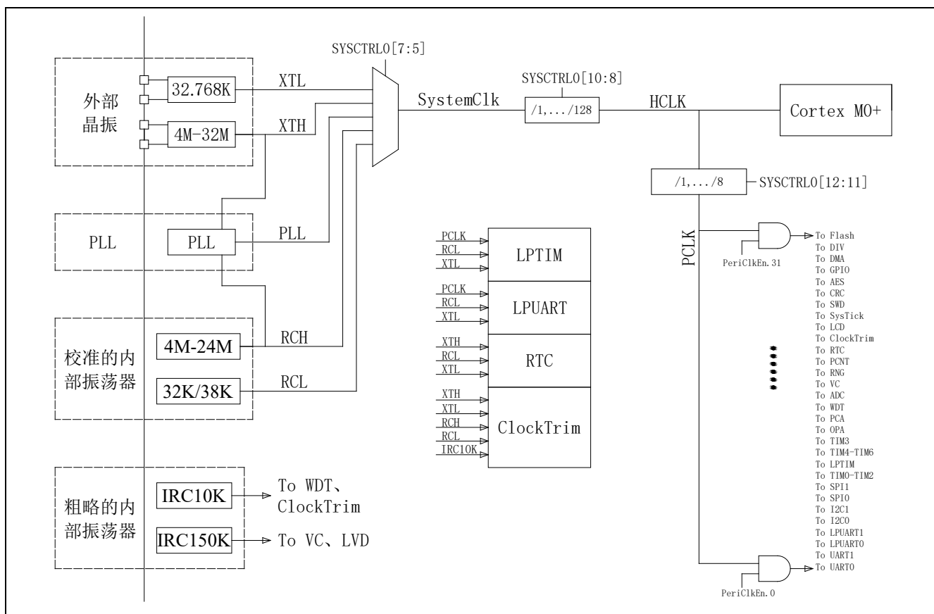
图 3-1 时钟控制模块框图
