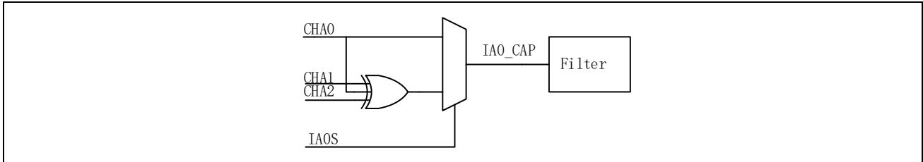
图 14-49 CHA 端口选择
