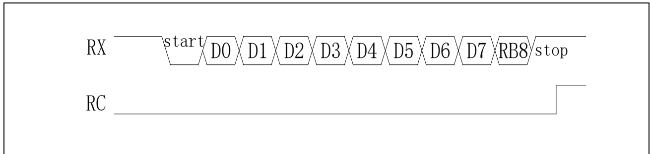
图 21-7 Mode2 接收数据
