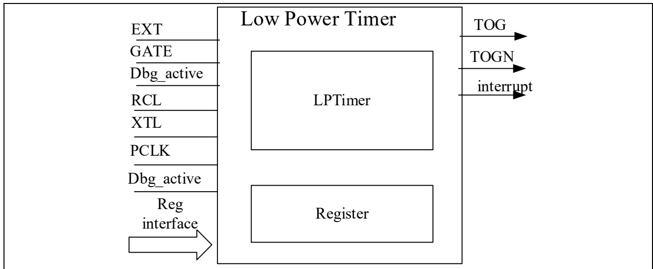
图 15-1 LPTimer 框图
