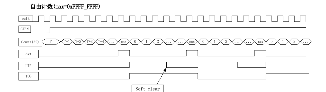
图 14-7 自由计数时序图
