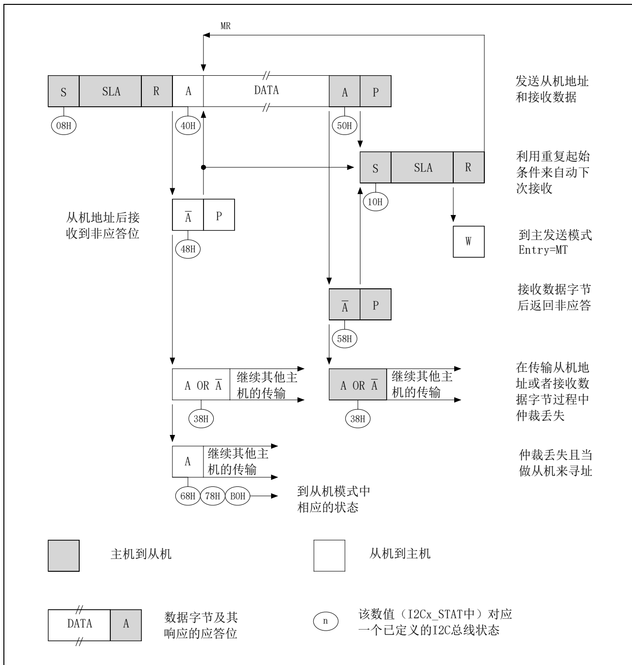
图 7-10 I2C 主机接收状态图
