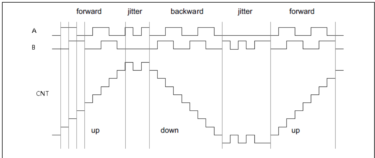
图 14-54 编码计数
