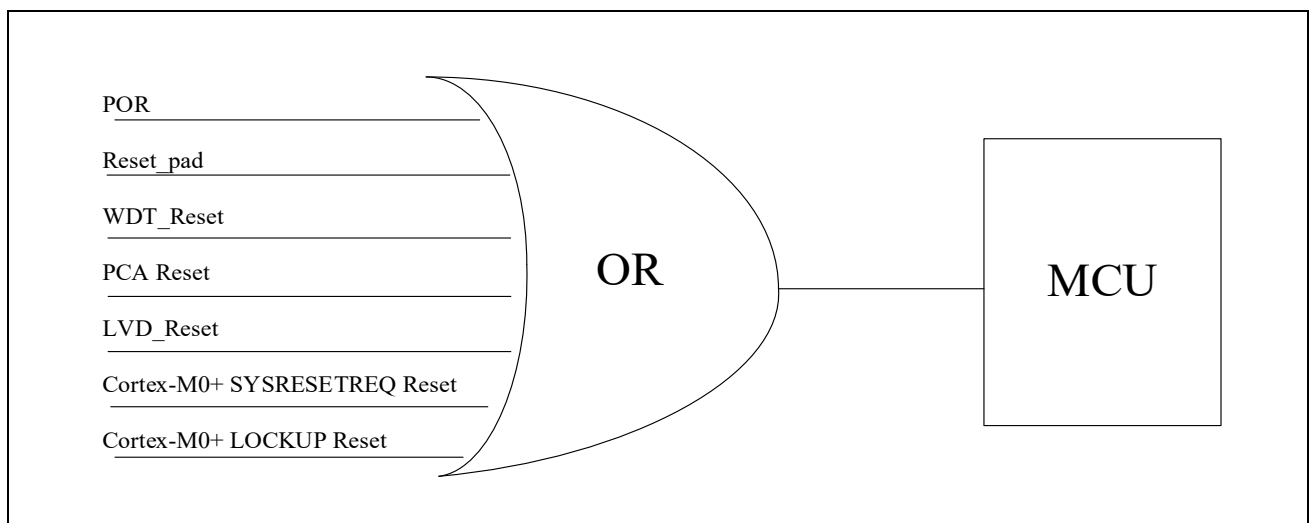
图 4-1 复位来源示意图
