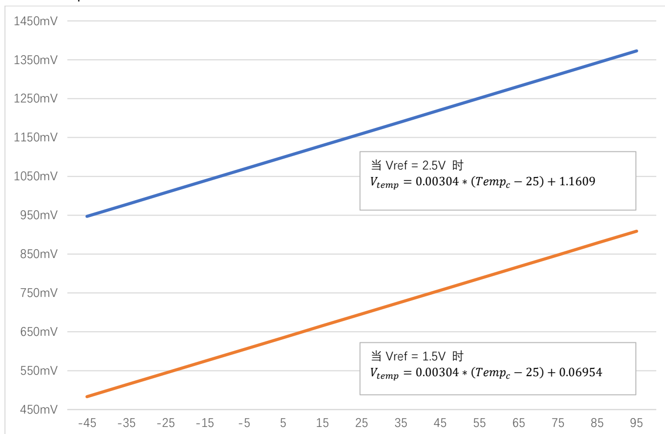
图 27-9 温度电压曲线
