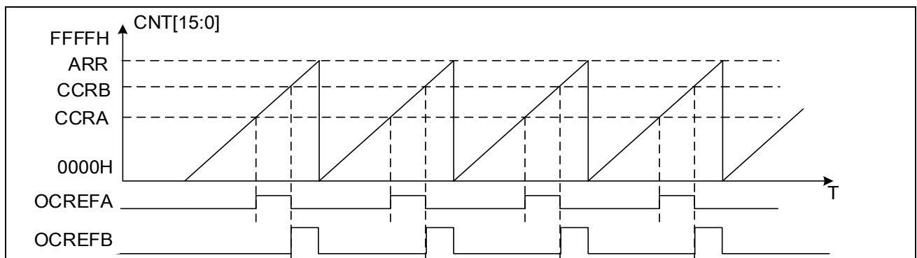
图 14-34 锯齿波计数双点比较 OREF 输出 (OCMx=111)
