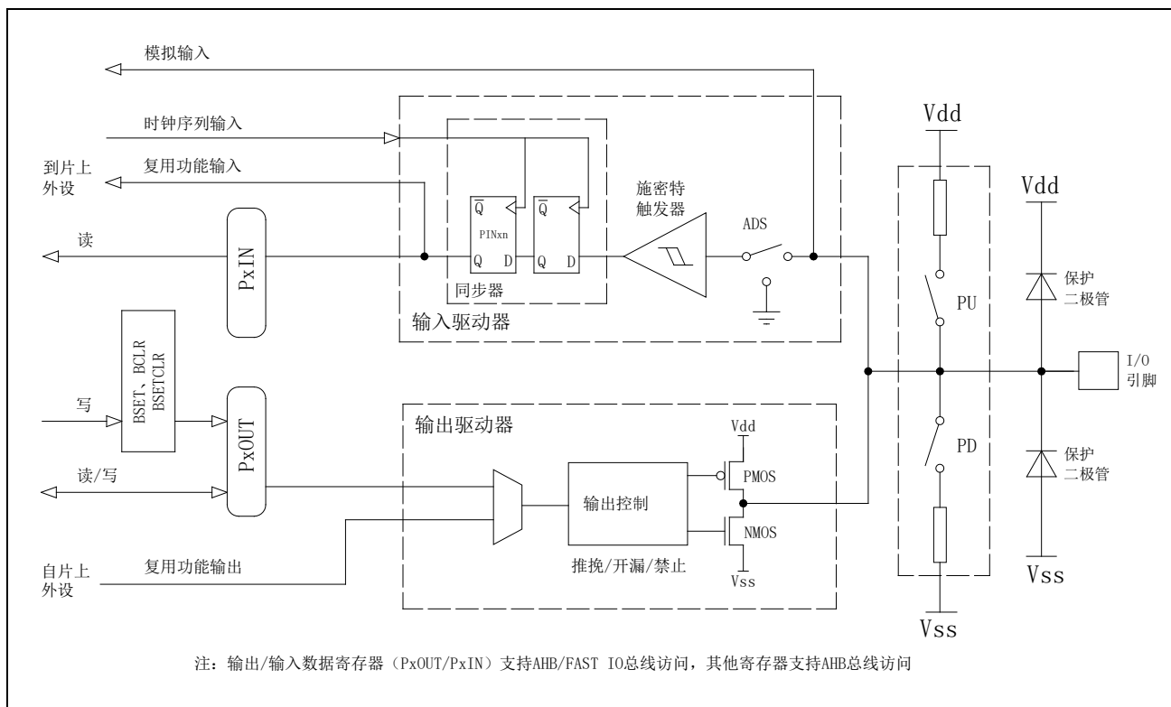
图 6-1 端口电路图
