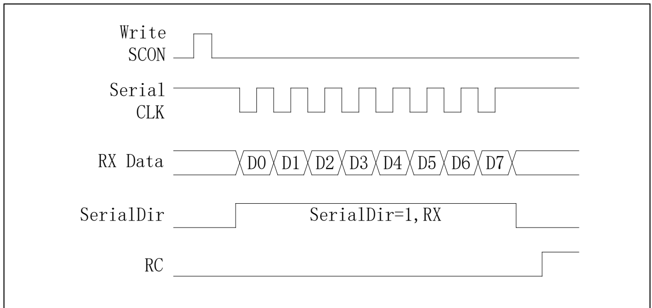
图 21-3 Mode0 接收数据
