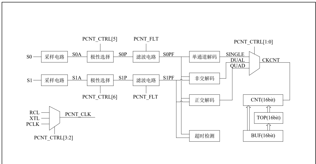
图 20-1 整体框图
