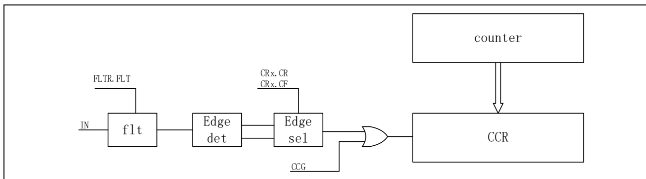
图 14-47 捕获功能框图
