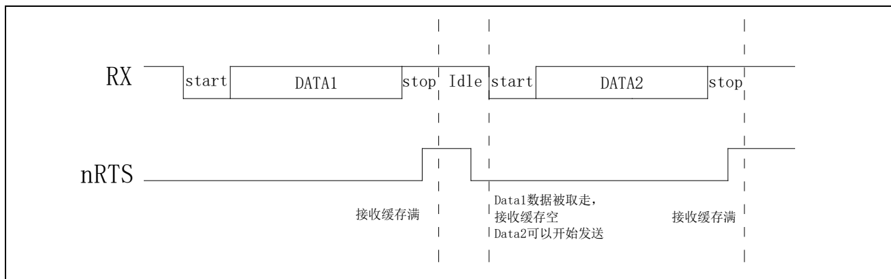
图 22-11 nRTS 硬件流控信号
