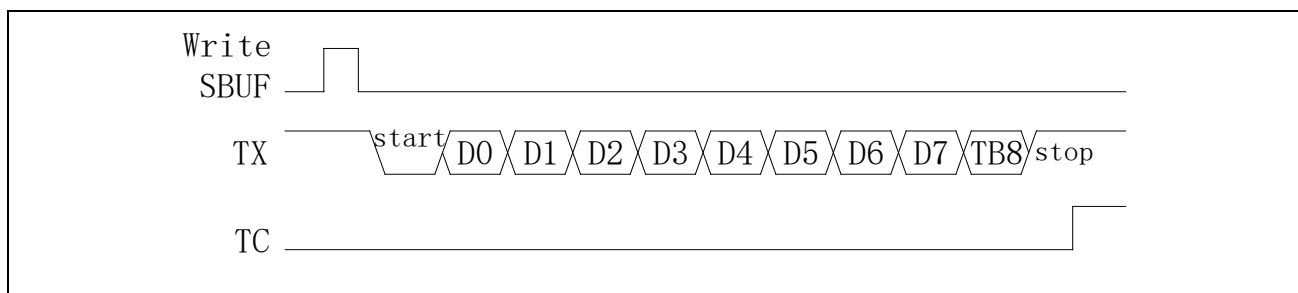
图 22-8 Mode3 发送数据
