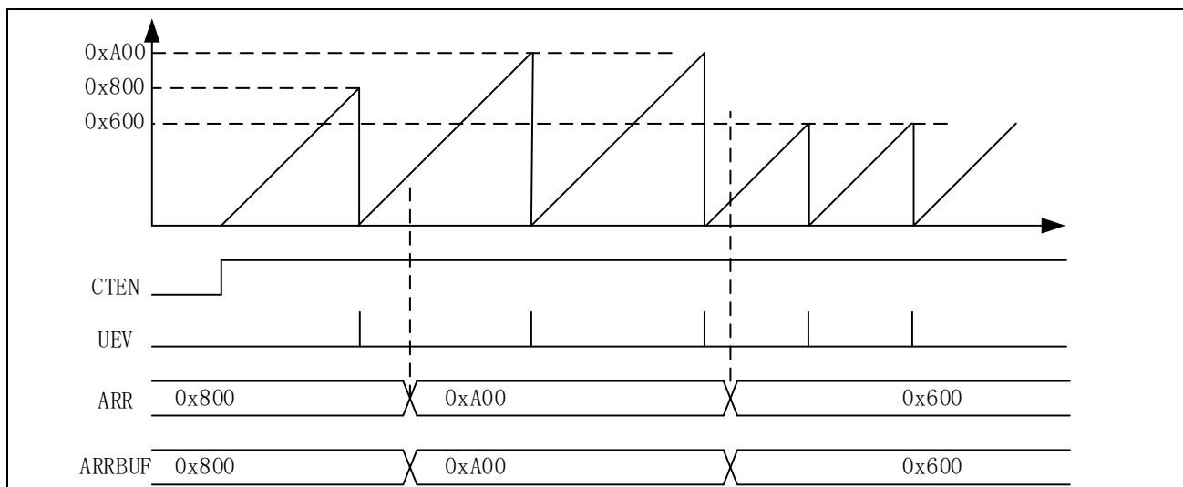
图 14-27 锯齿波模式下上计数缓存无效
