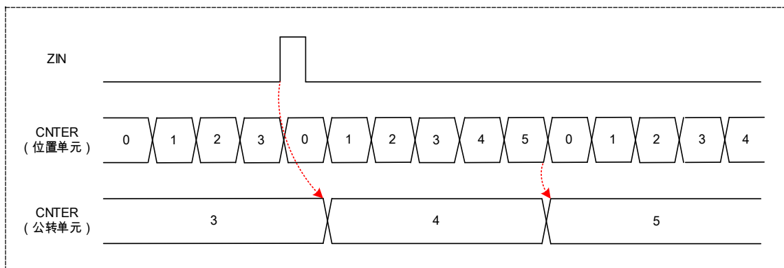
图 17-23 公转模式时 Z 相计数和位置计数器输出混计数动作
