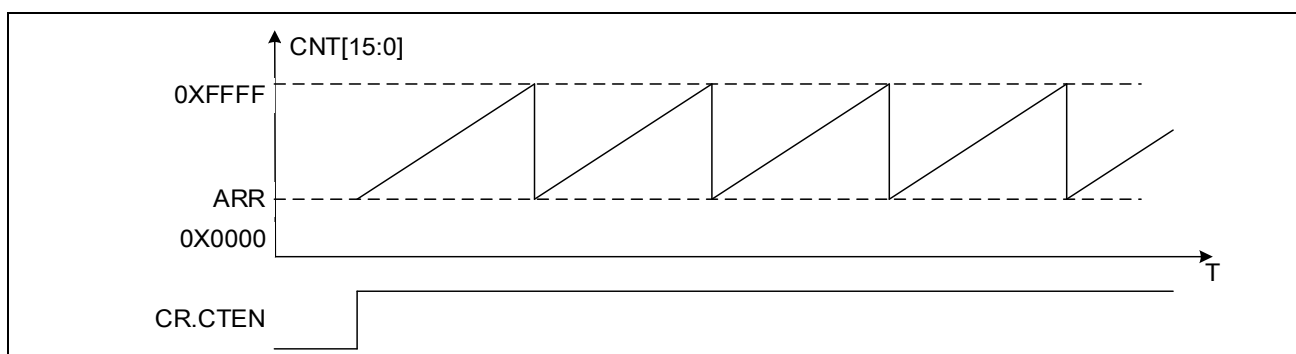
图 14-5 16 位重载计数波形
