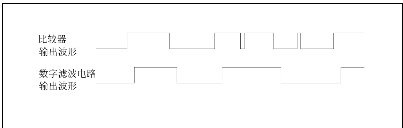
图 28-2 VC 滤波响应时间
