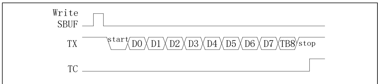
图 22-6 Mode2 发送数据
