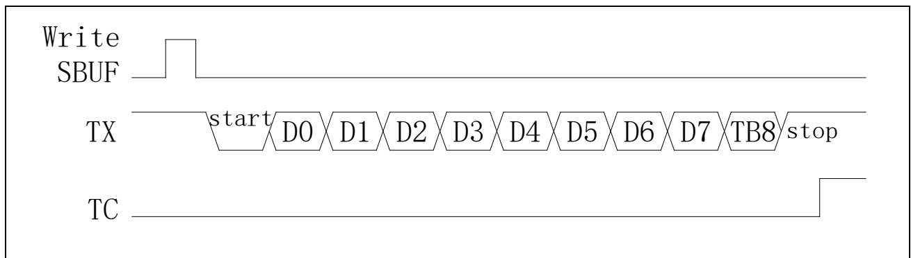
图 21-8 Mode3 发送数据
