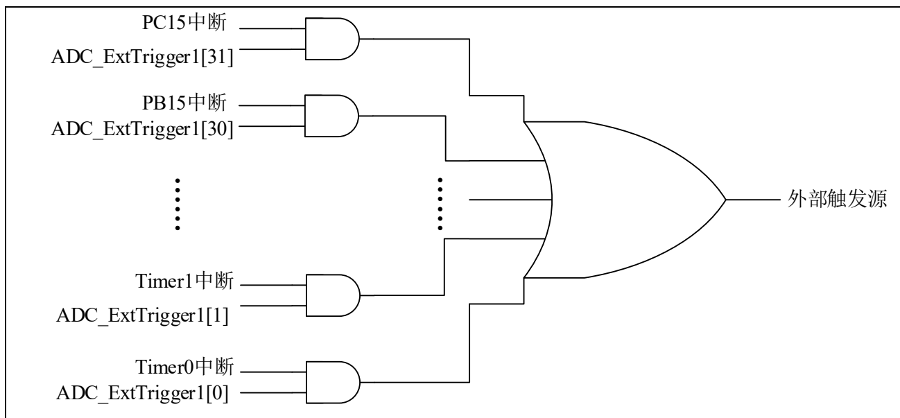
图 27-8 ADC 插队扫描转换外部触发源示意图
