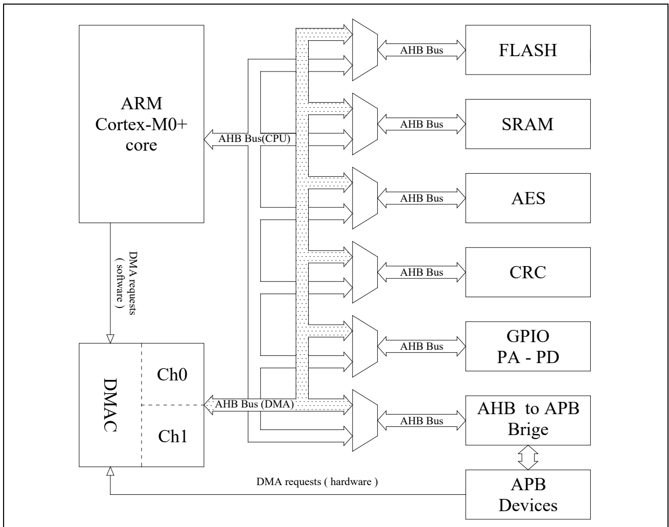
图 13-1 功能框图
