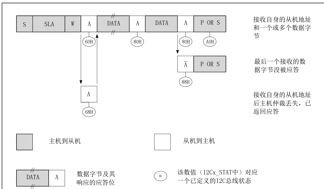
图 7-12 从机接收状态图
