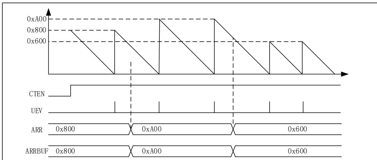
图 14-29 锯齿波模式下计数缓存无效
