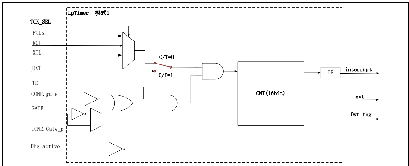
图 15-2 LPTimer 模式 1
