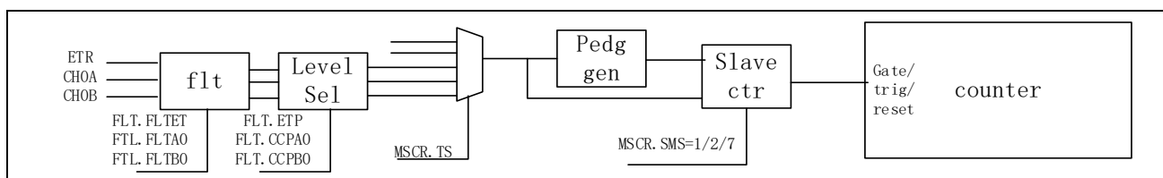
图 14-51 从模式示意图
