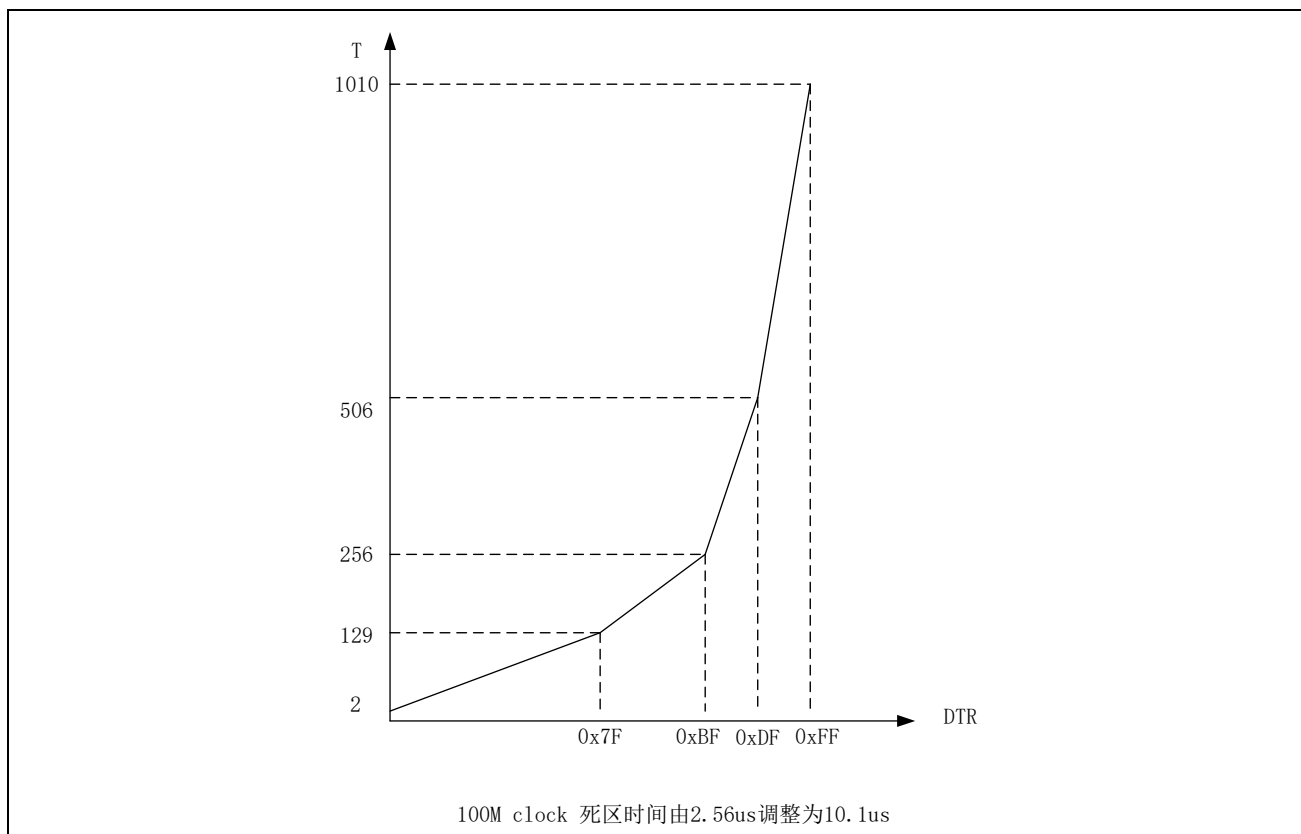
图 14-42 死区时间
