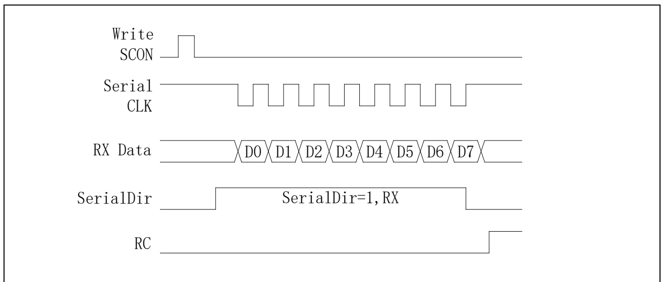
图 22-3 Mode0 接收数据
