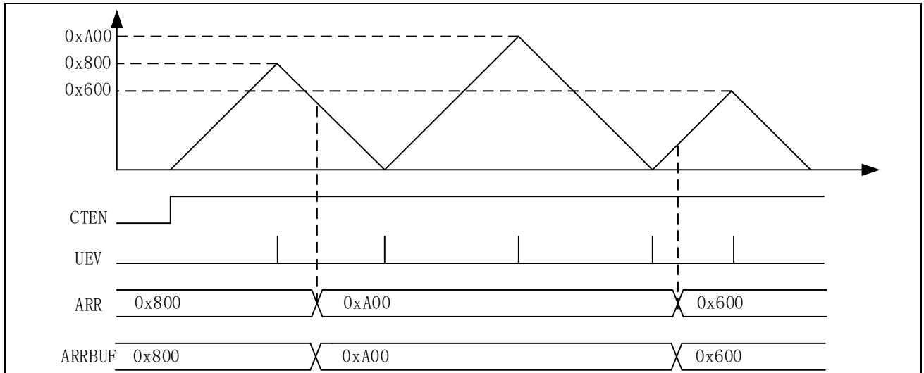
图 14-25 三角波模式下缓存无效
