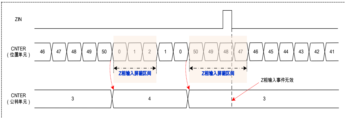
图 17-25 公转计数模式-混合计数 Z 相屏蔽动作例 2
