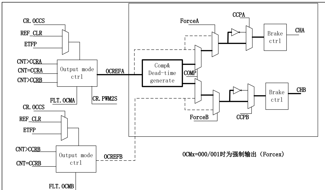
图 14-39 互补 PWM 输出框图
