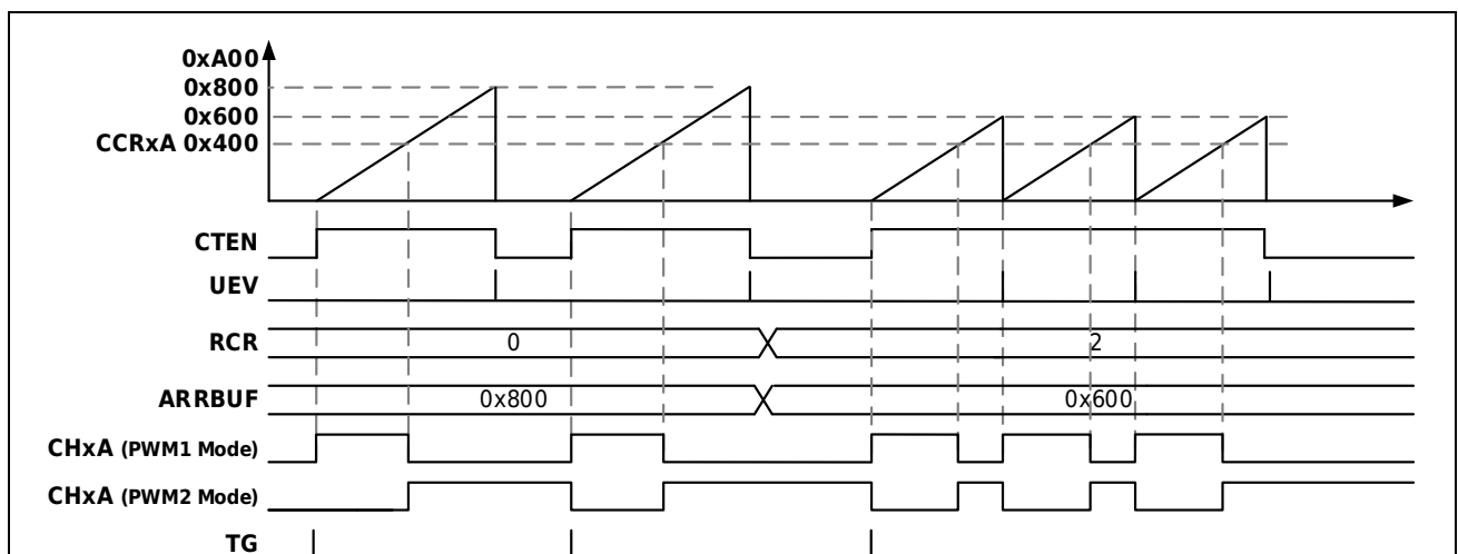
图 14-44 锯齿波上计数单脉冲模式
