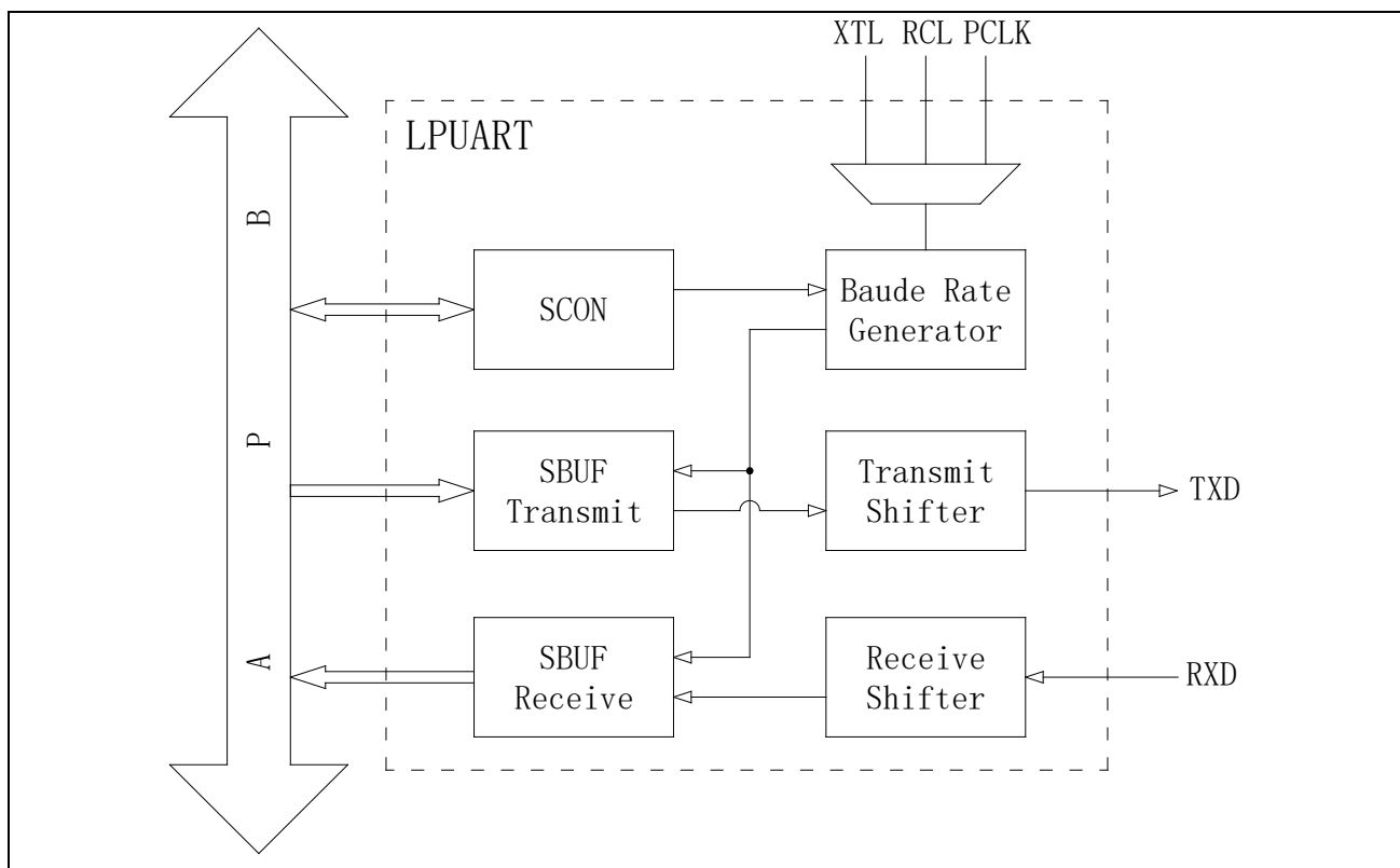
图 22-1 结构框图
