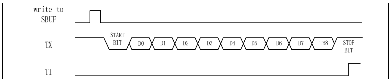
图 16-6 Mode2 发送数据
