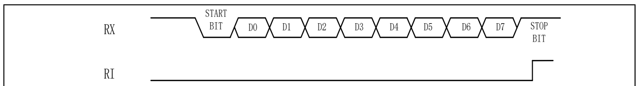
图 15-5 Mode1 接收数据
