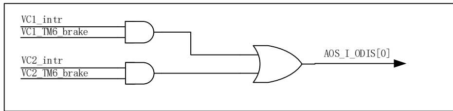
图 12-29 VC 刹车控制示意图
