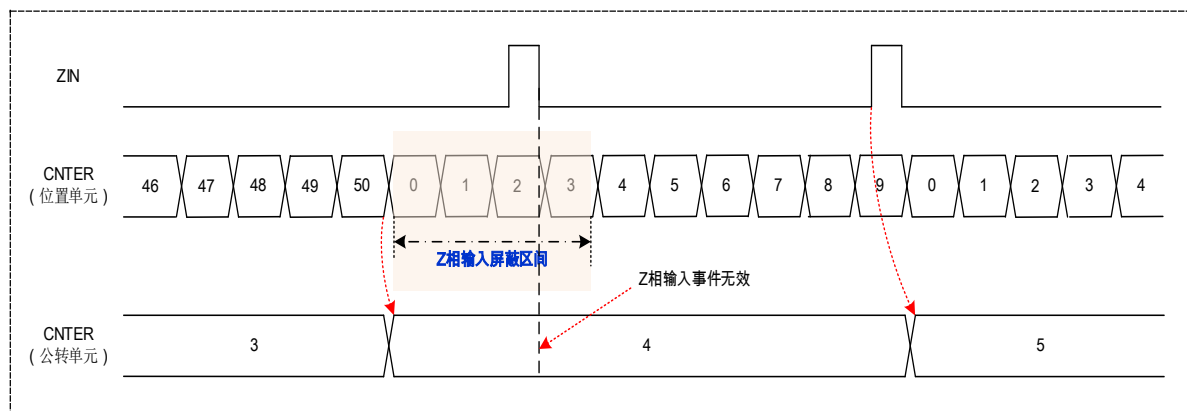
图 12-24 公转计数模式-混合计数 Z 相屏蔽动作例 1
