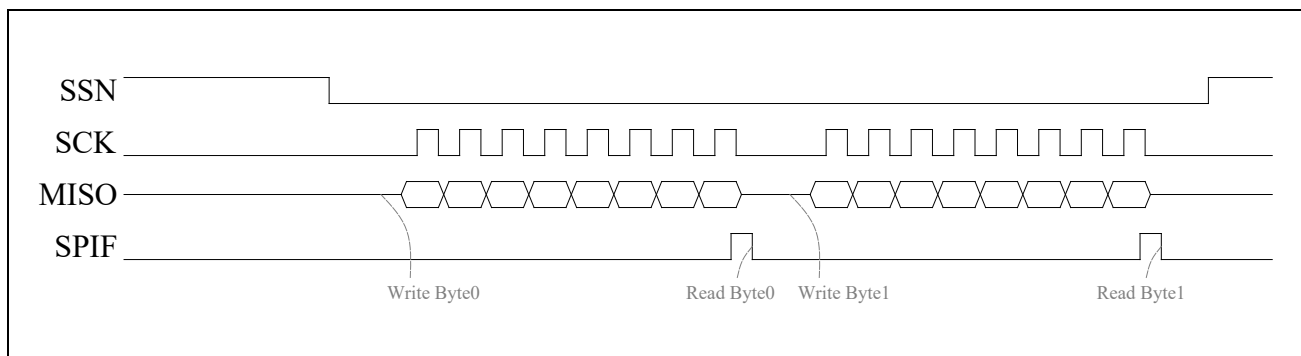
图 18-2 从机发送示意图
