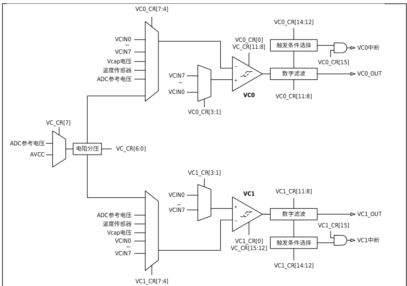
图 22-1 VC 框架图
