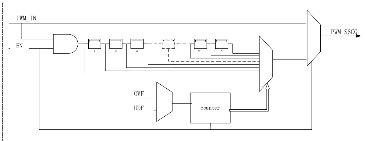
图 12-10 PWM 展频输出示意图
