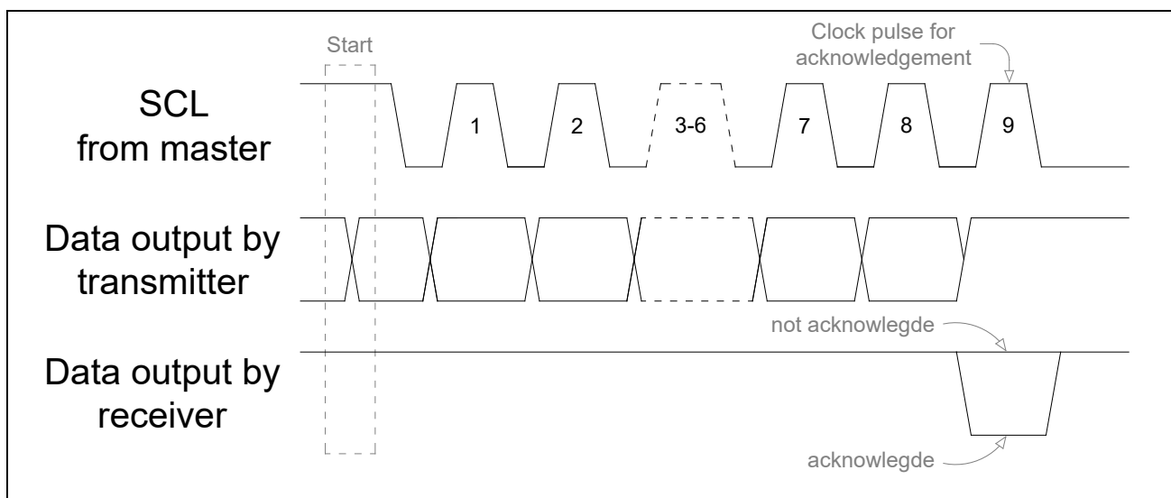
图 17-4 I2C 总线上应答信号
