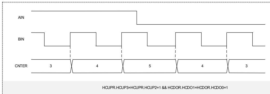
图 12-20 位置模式时方向计数动作
