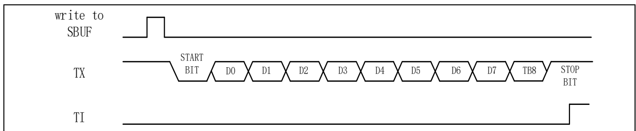
图 15-8 Mode3 发送数据
