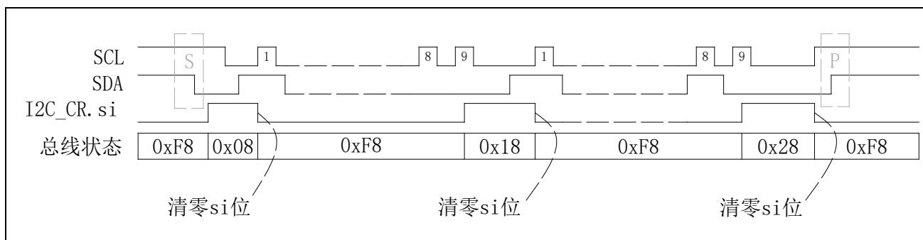
图 17-7 主发送模式数据同步图
