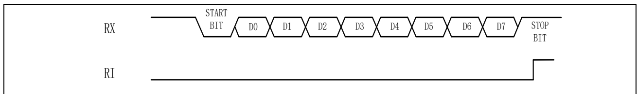
图 16-5 Mode1 接收数据
