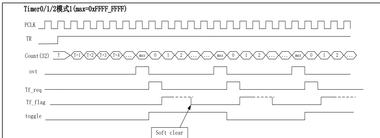
图 9-4 模式 1 时序图
