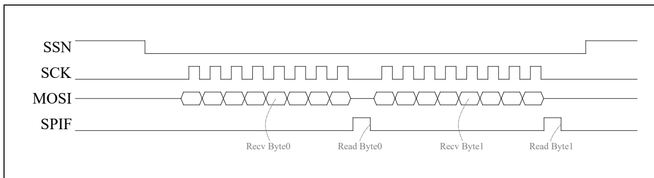
图 18-1 从机接收示意图
