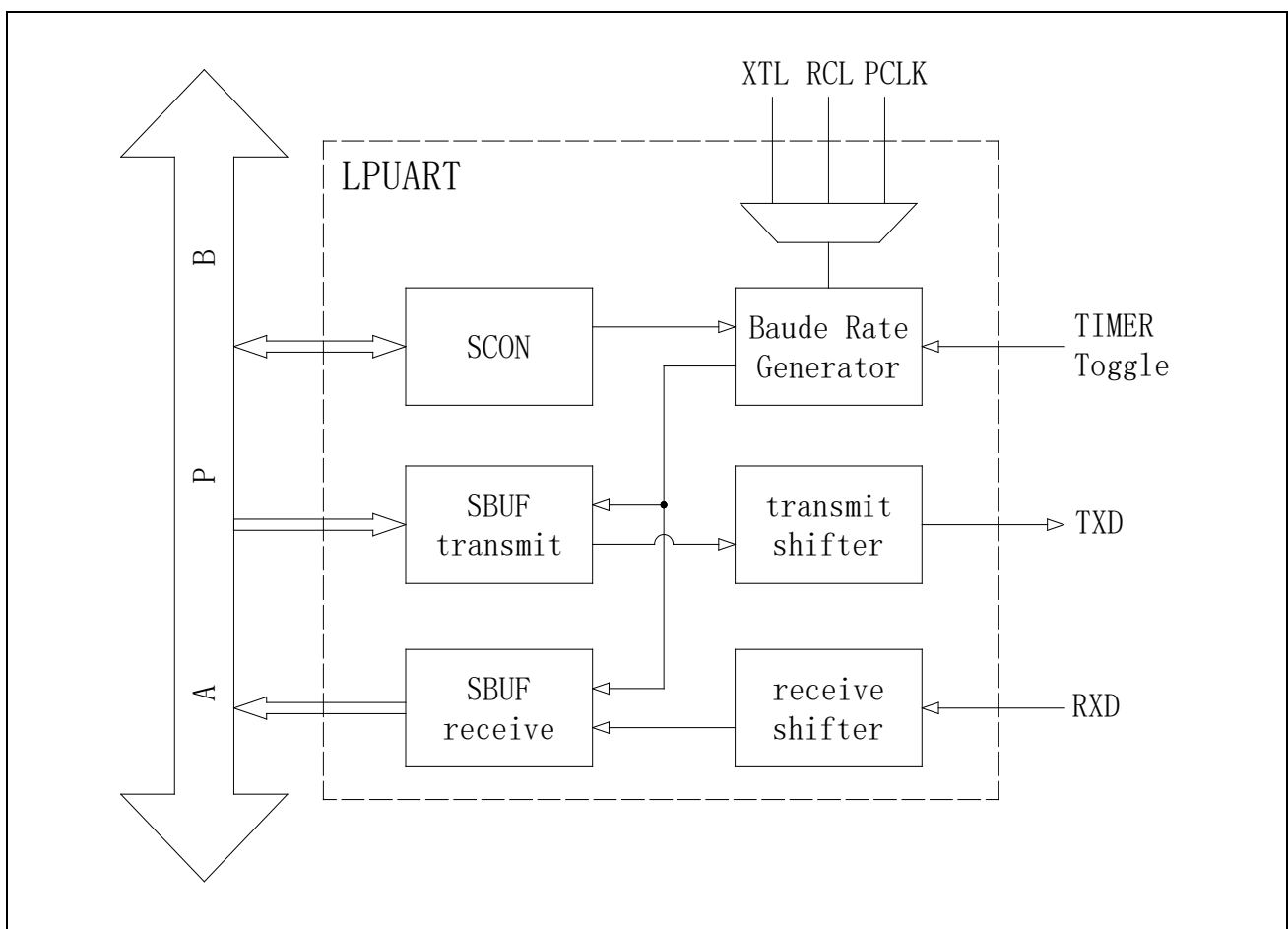
图 16-1 LPUART 结构框图
