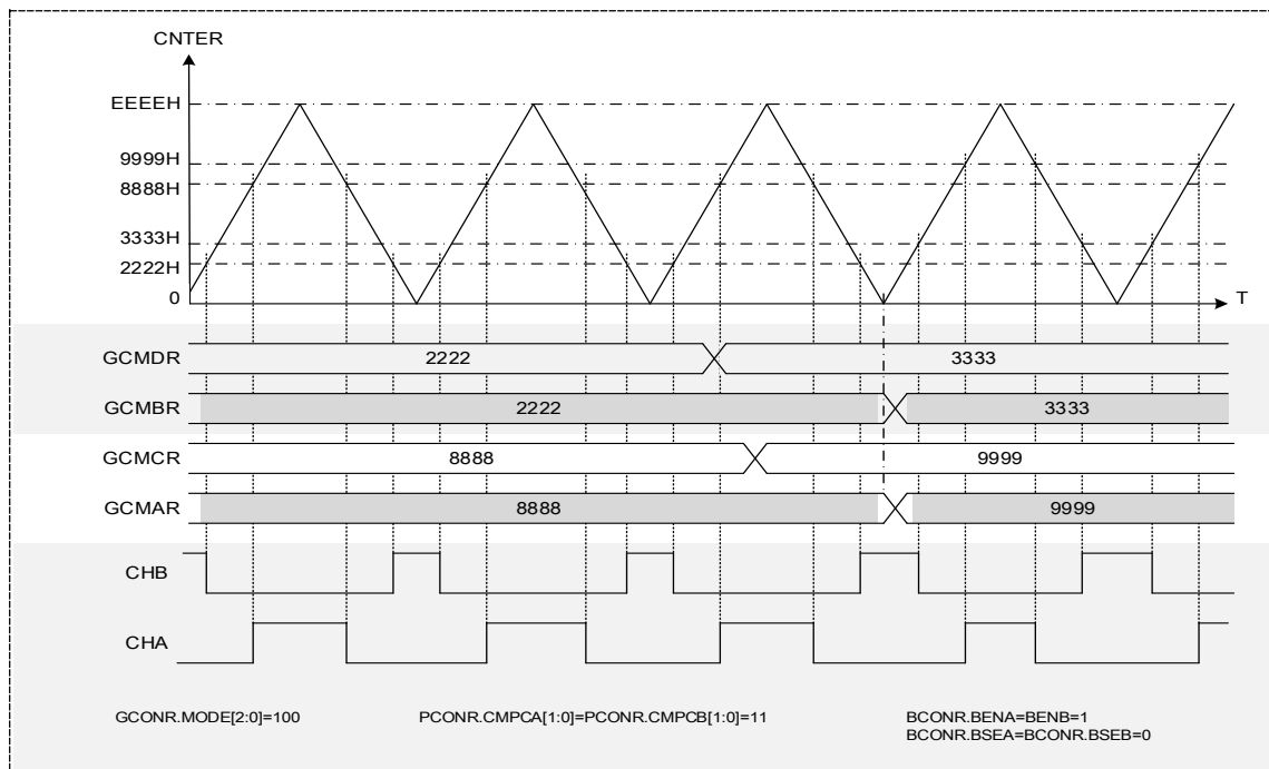
图 12-12 三角波 A 模式时软件设定 GCMBR 互补 PWM 波输出
