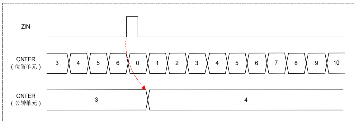
图 12-21 公转模式时 Z 相计数动作
