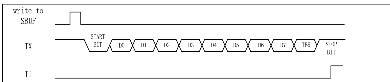
图 15-6 Mode2 发送数据
