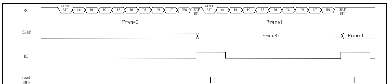
图 15-8 接收缓存
