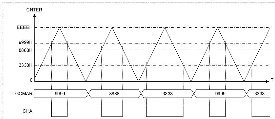
图 12-11 CHA 输出 PWM 波
