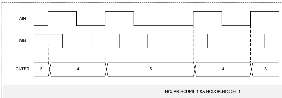
图 12-17 位置模式时相位差计数动作设定(1 倍)
