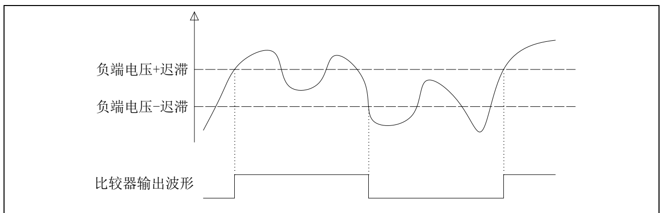
图 22-3 VC 迟滞功能
