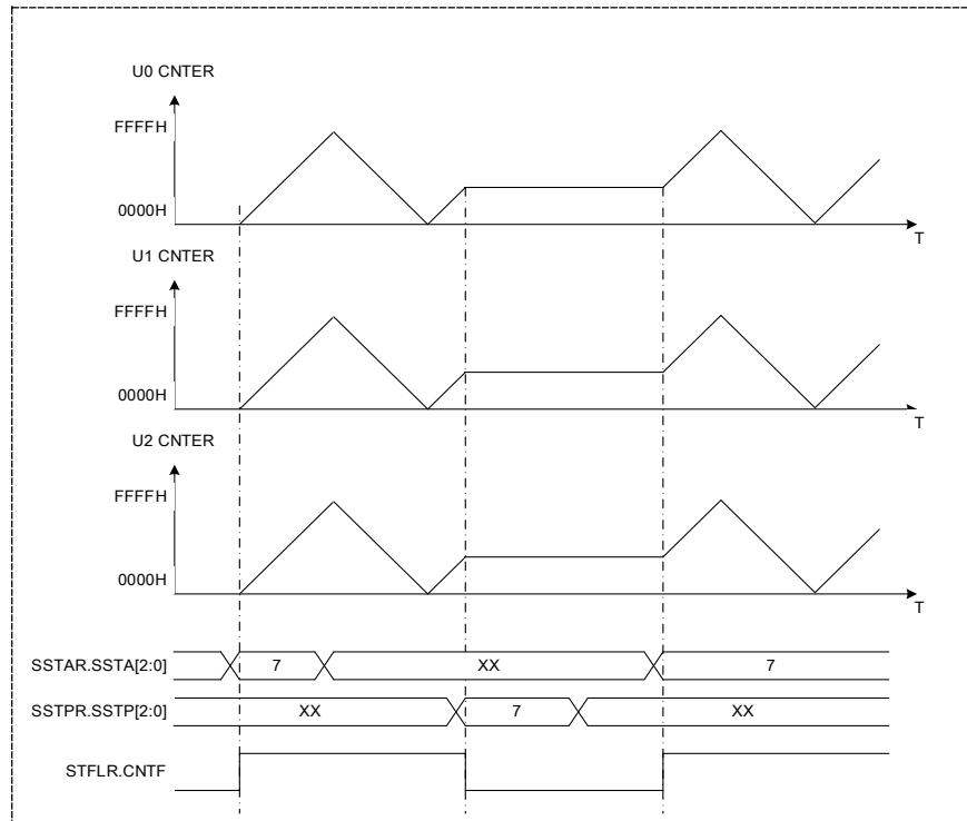
图 12-7 软件同步动作
