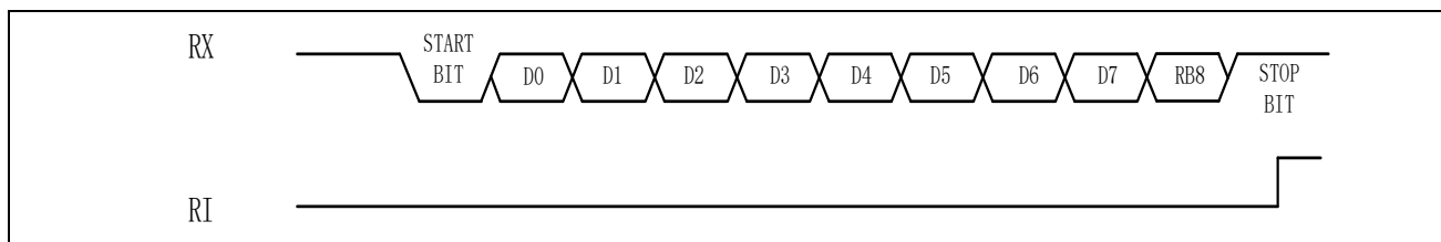
图 16-7 Mode2 接收数据
