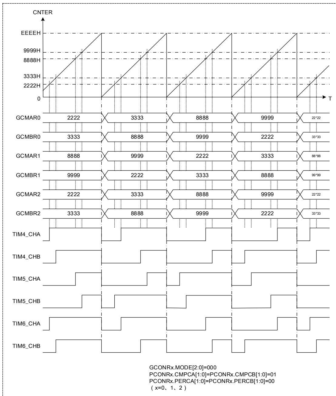
图 12-14 6 相 PWM 波
