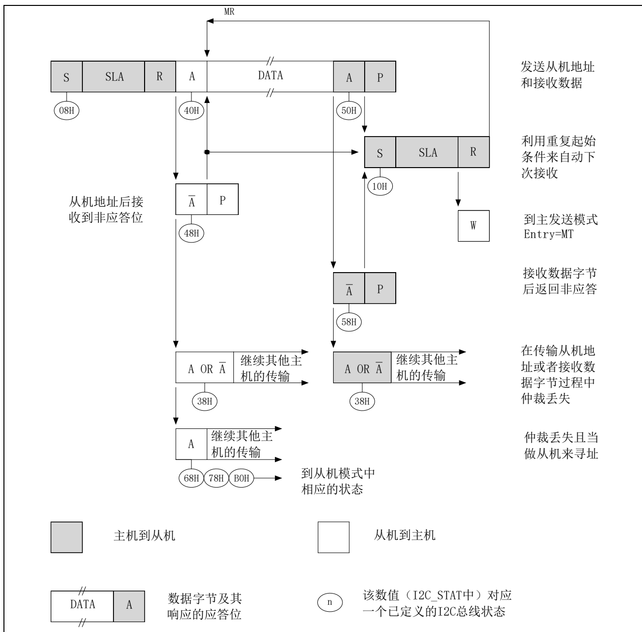
图 17-10 I2C 主机接收状态图
