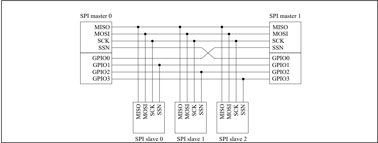
图 18-6 SPI 多主机/多从机系统的示意图
