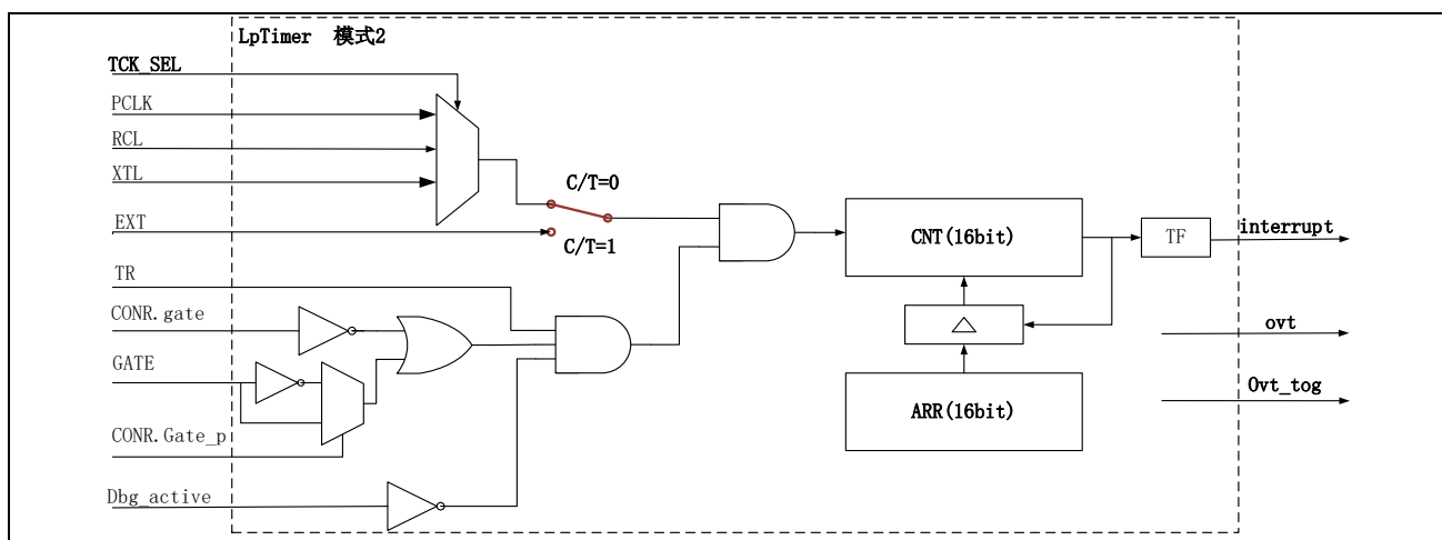
图 10-3 LpTimer 模式 2
