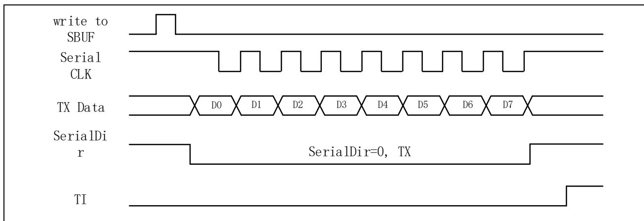
图 16-2 Mode0 发送数据
