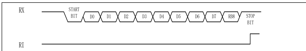
图 15-7 Mode2 接收数据
