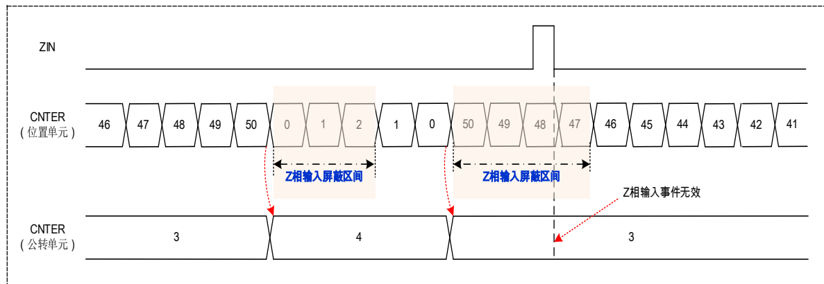
图 12-25 公转计数模式-混合计数 Z 相屏蔽动作例 2
