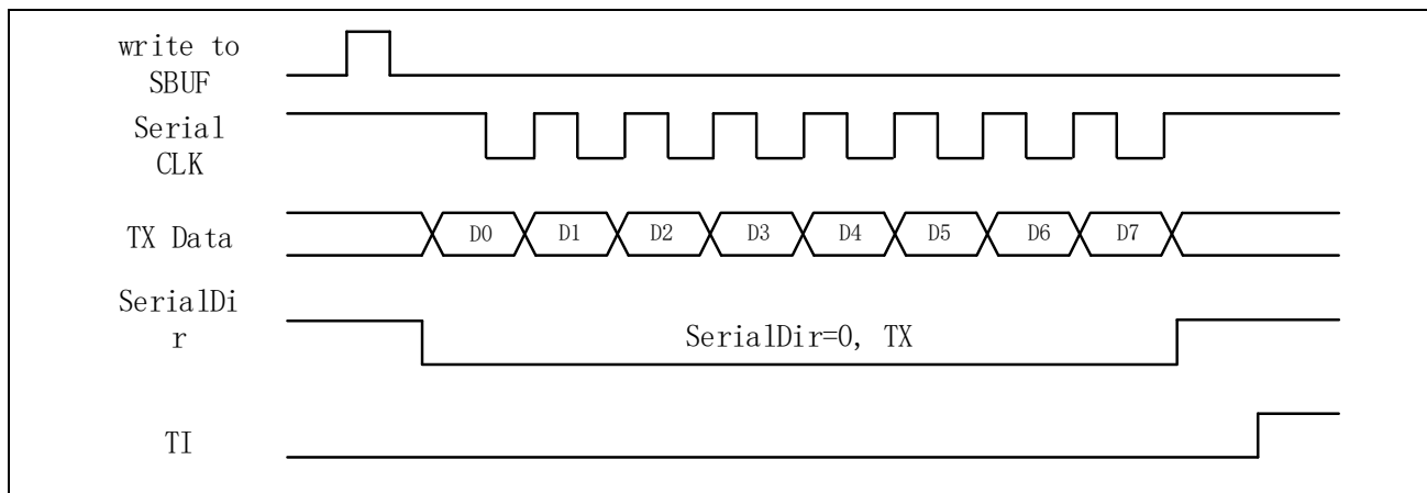
图 15-2 Mode0 发送数据
