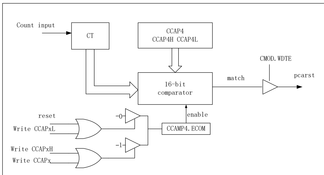
图 11-5 PCA WDT 功能框图
