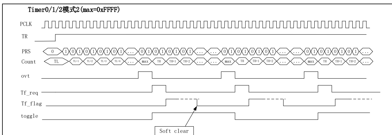
图 9-5 模式 2 时序图 (预分频设置为 2)
