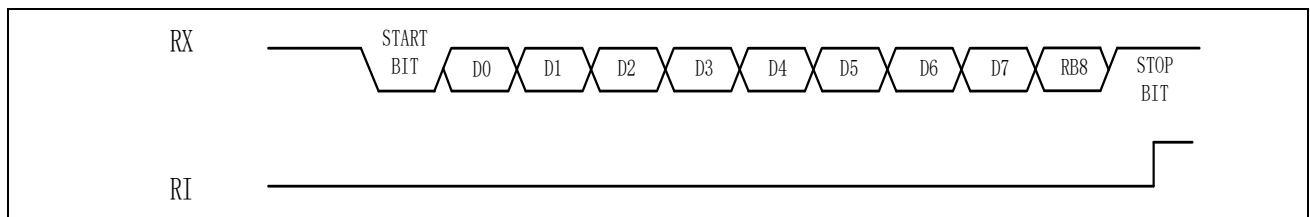
图 15-9 Mode3 接收数据
