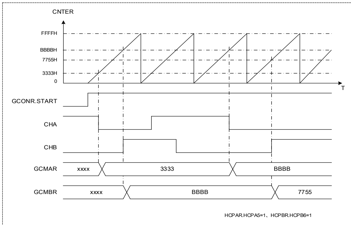
图 12-5 捕获输入动作
