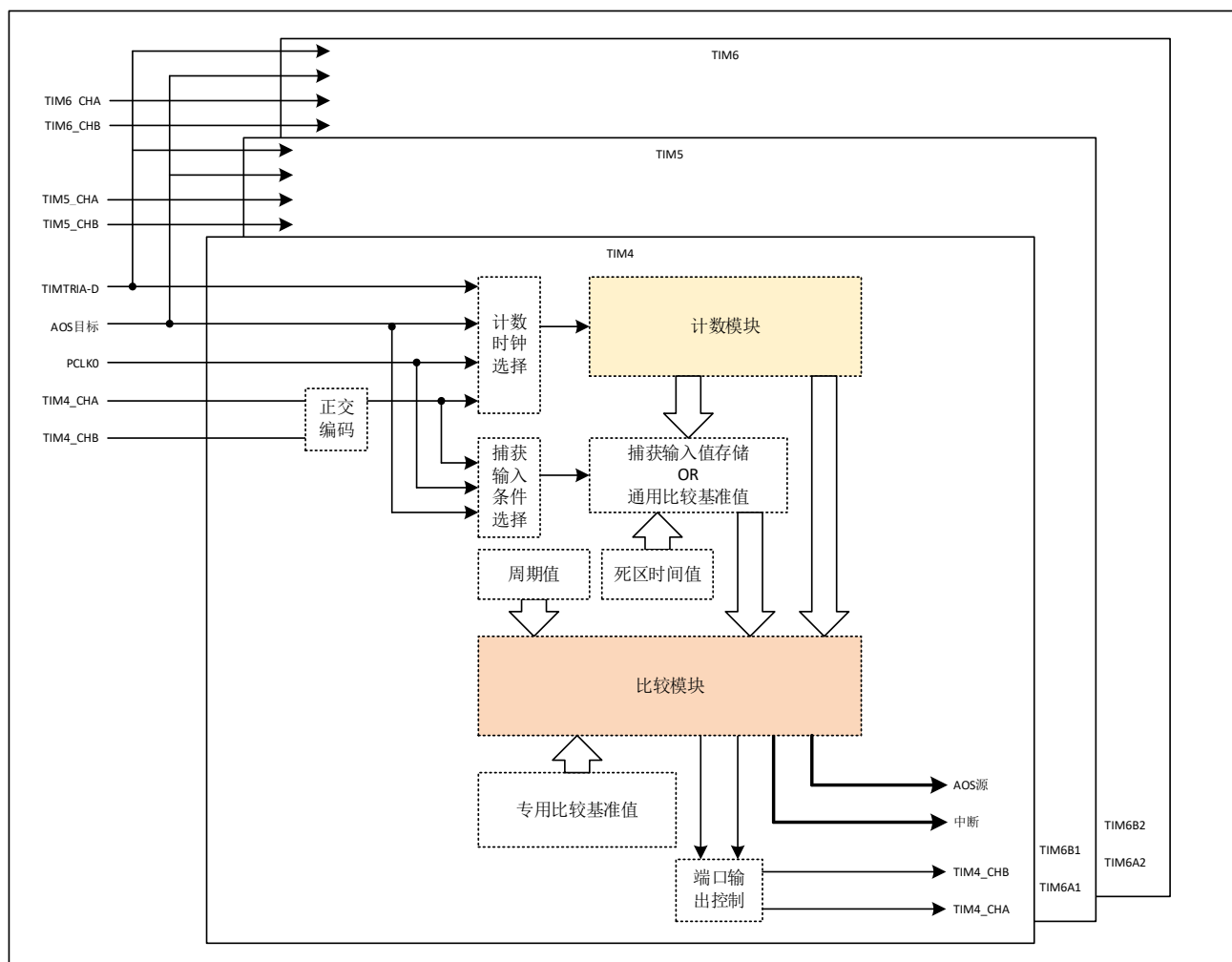
图 12-1 Advanced Timer 框图
