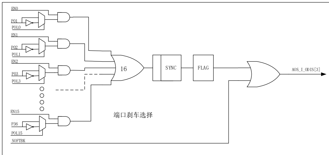
图 12-27 端口刹车与软件刹车示意图
