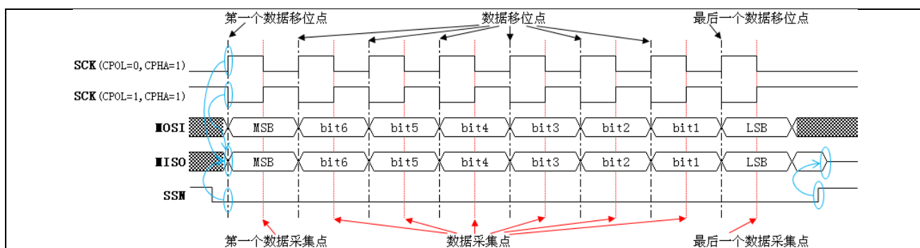
图 18-5 从机 CPHA 为 1 时数据帧格式
