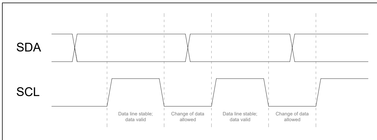
图 17-3 I2C 总线上位传输
