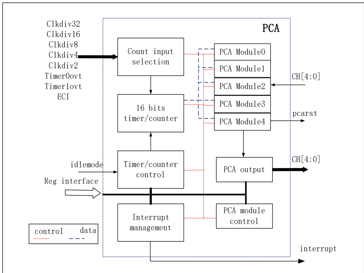
图 11-1 PCA 整体框图
