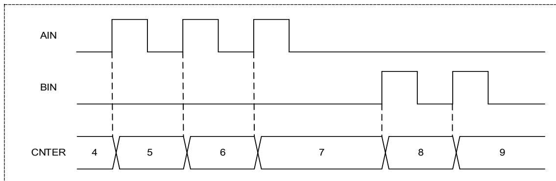
图 12-16 位置模式时基本计数动作
