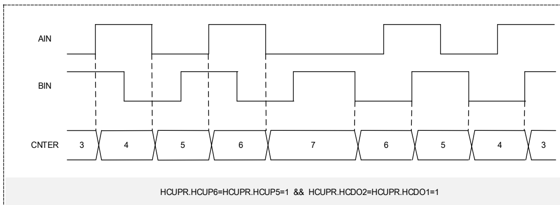
图 12-18 位置模式时相位差计数动作设定(2 倍)
