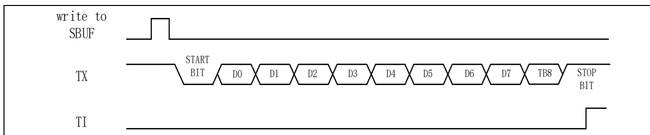
图 16-8 Mode3 发送数据
