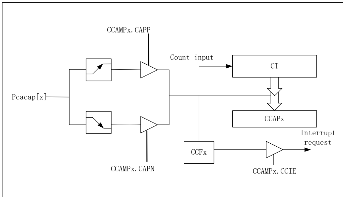
图 11-3 PCA 捕获功能框图
