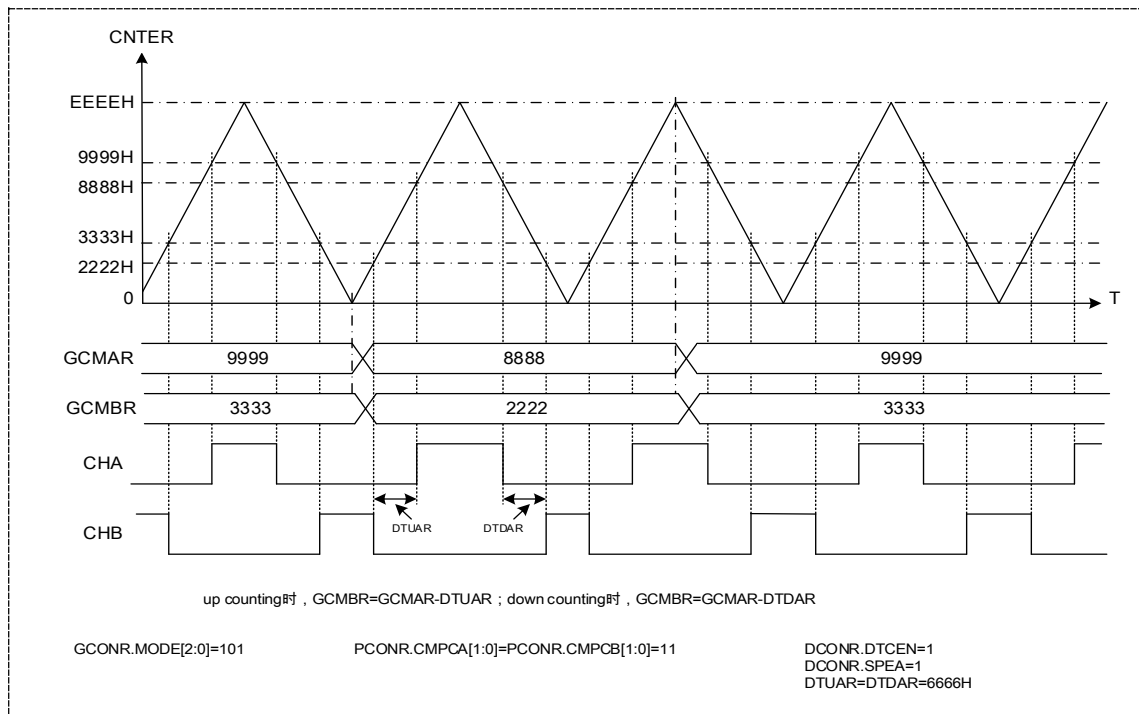
图 12-13 三角波 B 模式时硬件设定 GCMBR 互补 PWM 波输出（对称死区）
