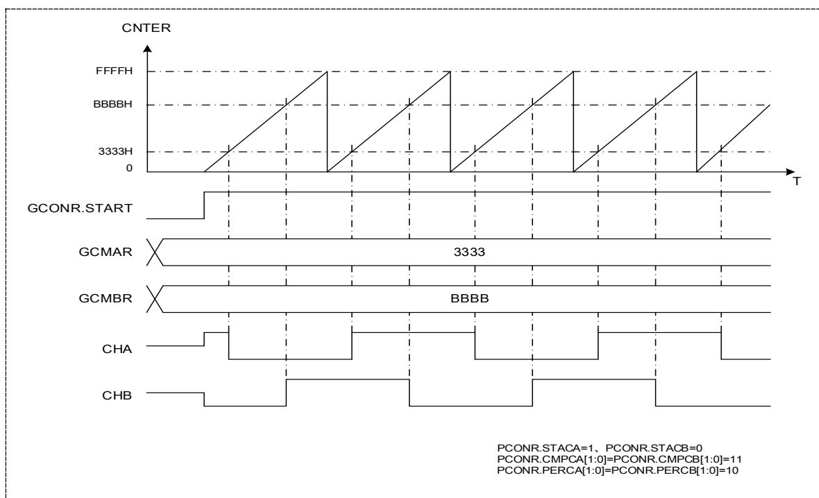
图 12-4 比较输出动作
