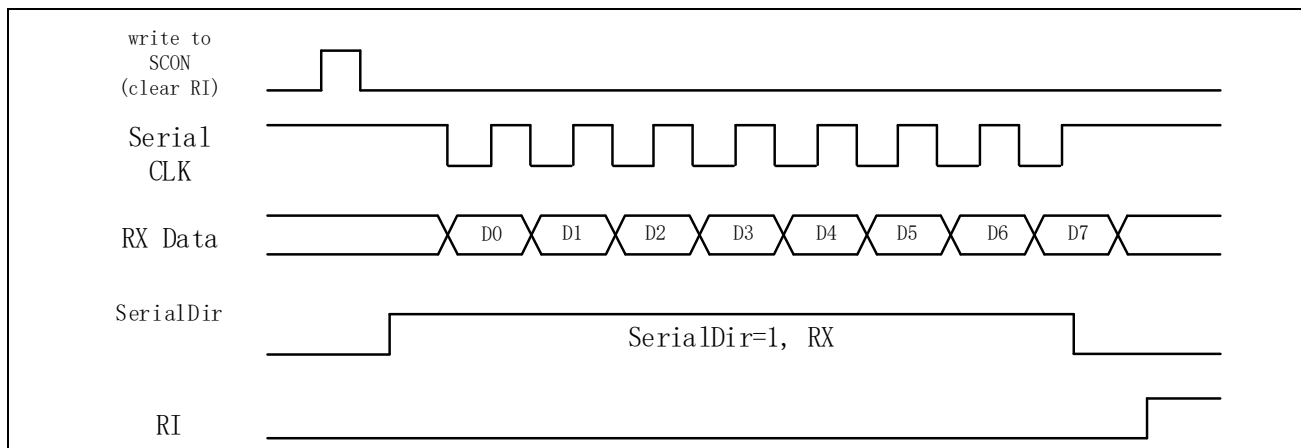
图 16-3 Mode0 接收数据
