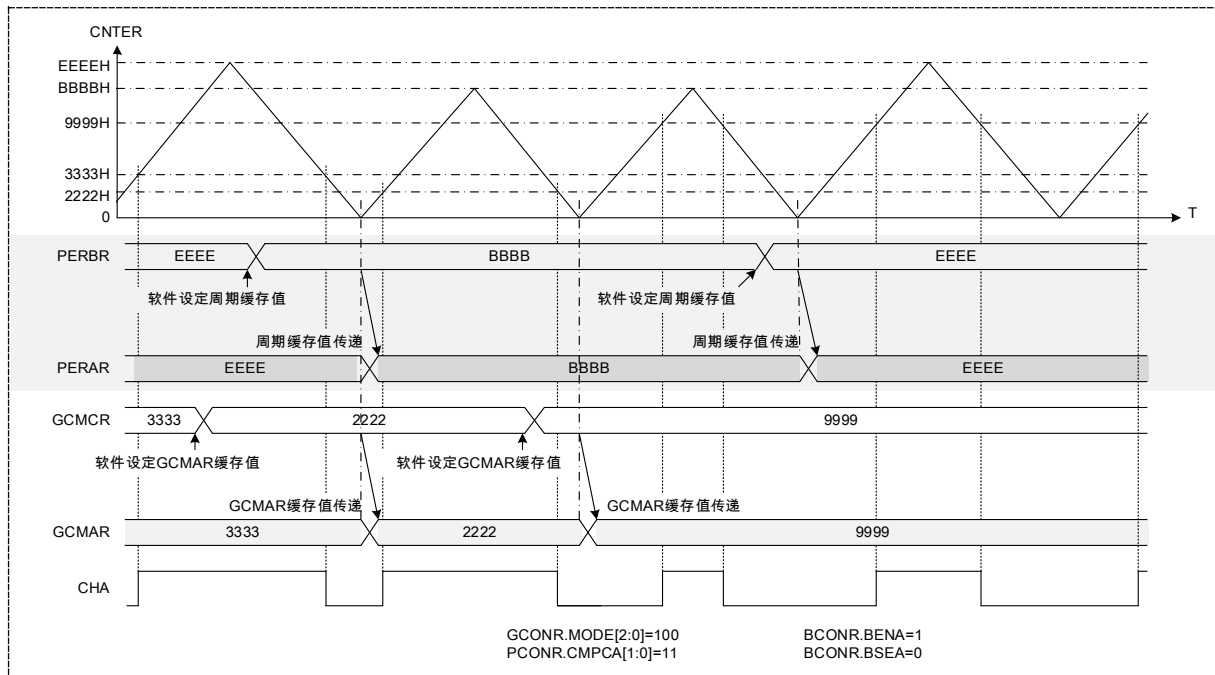
图 12-9 单缓存方式比较输出时序
