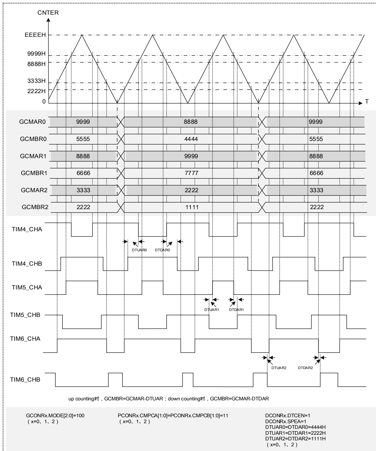
图 12-15 三角波 A 模式时带死区时间三相互补 PWM 波输出
