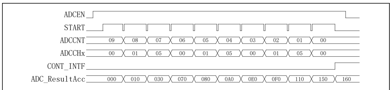
图 21-4 ADC 连续转换累加过程示例
