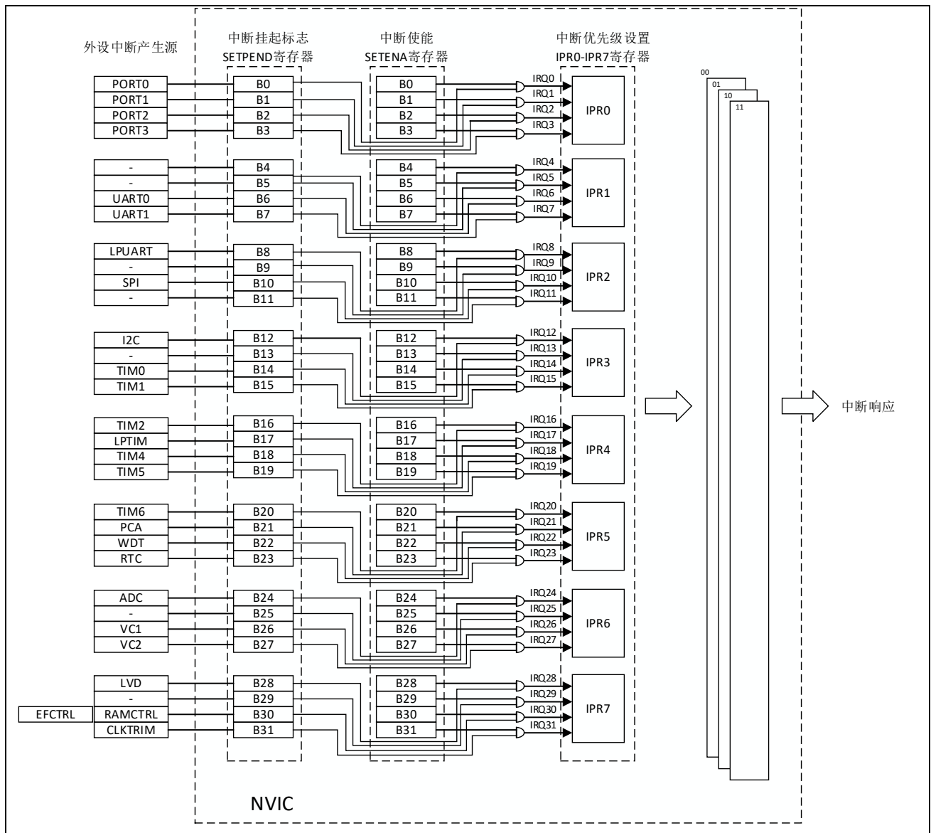
图 5-7 中断结构图
