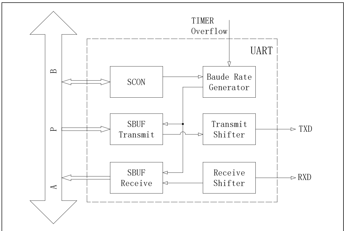
图 15-1 UART 结构框图
