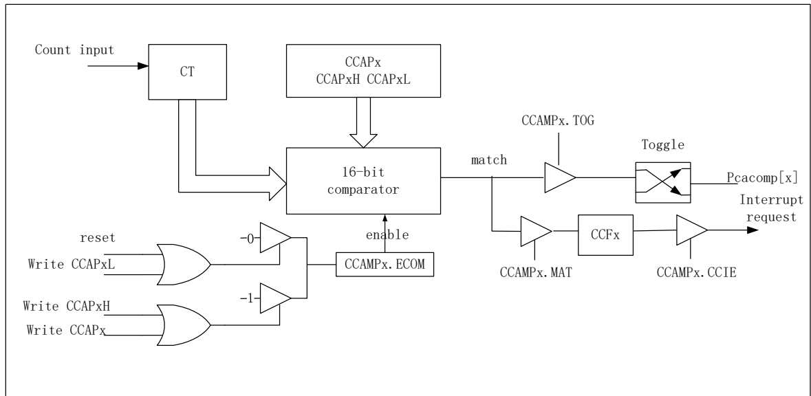
图 11-4 PCA 比较功能框图
