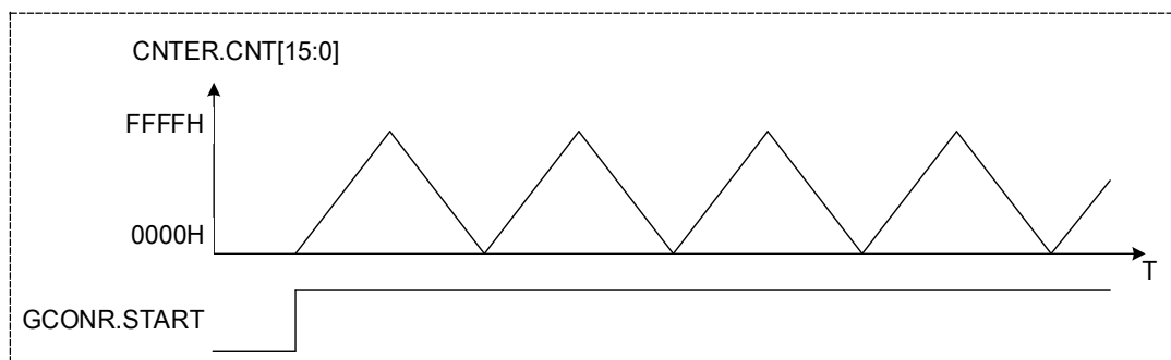
图 12-3 三角波波形
