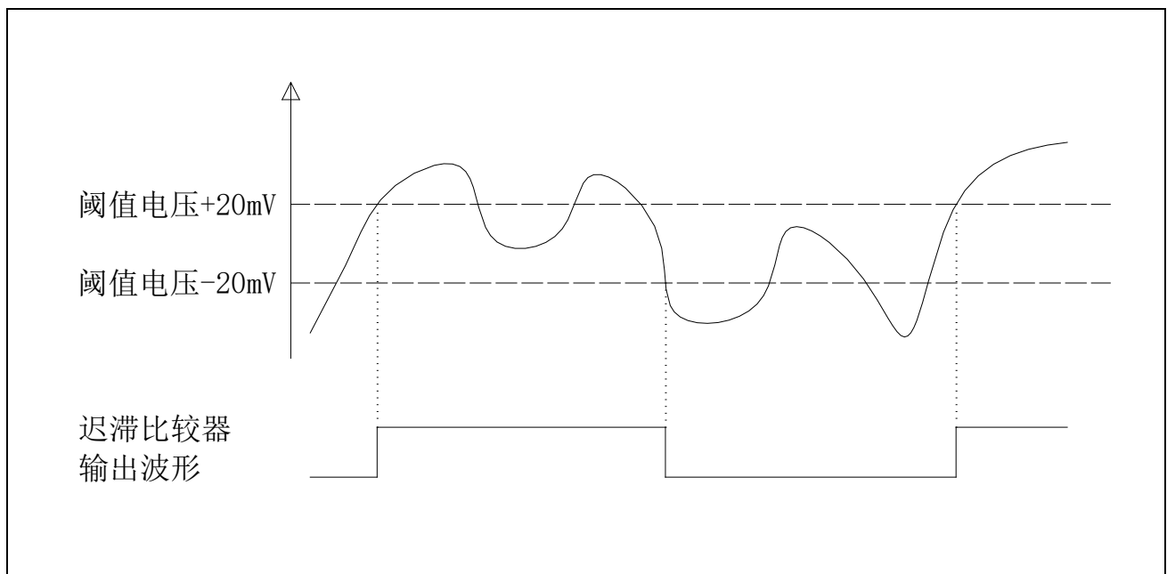
图 23-3 LVD 迟滞响应
