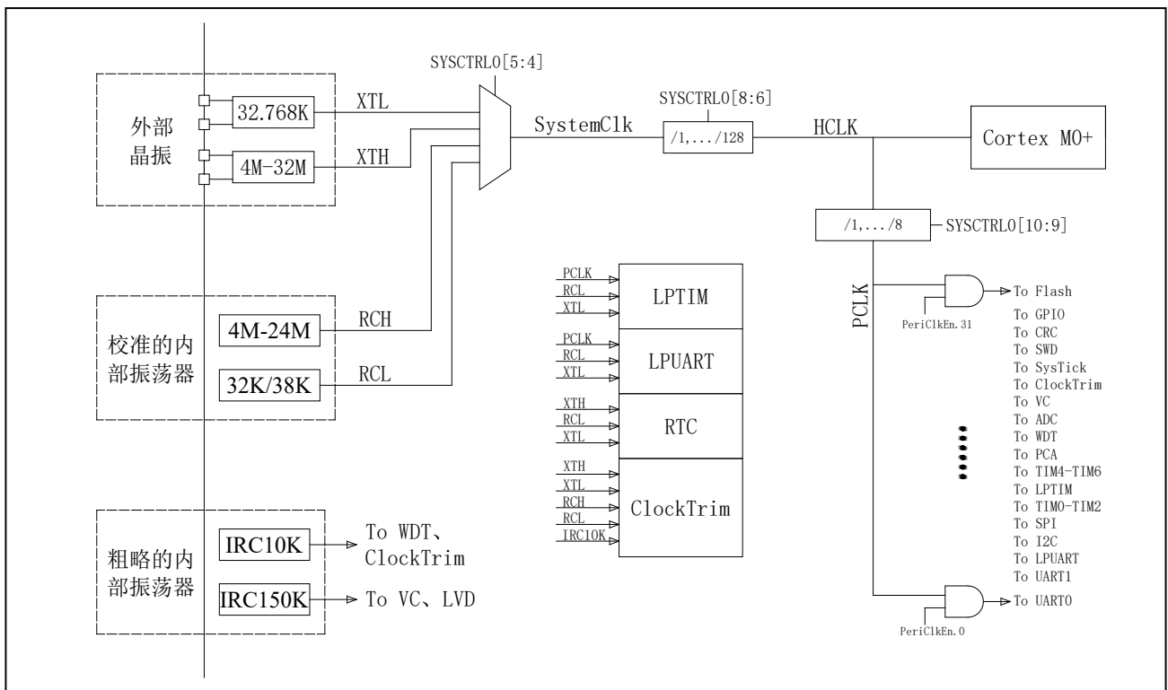
图 3-1 时钟控制模块框图
