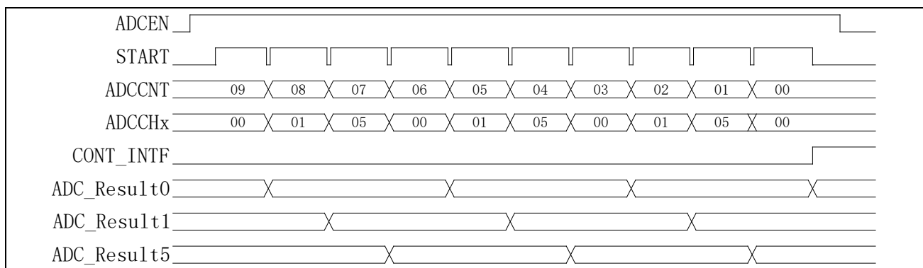
图 21-3 ADC 连续转换过程示例
