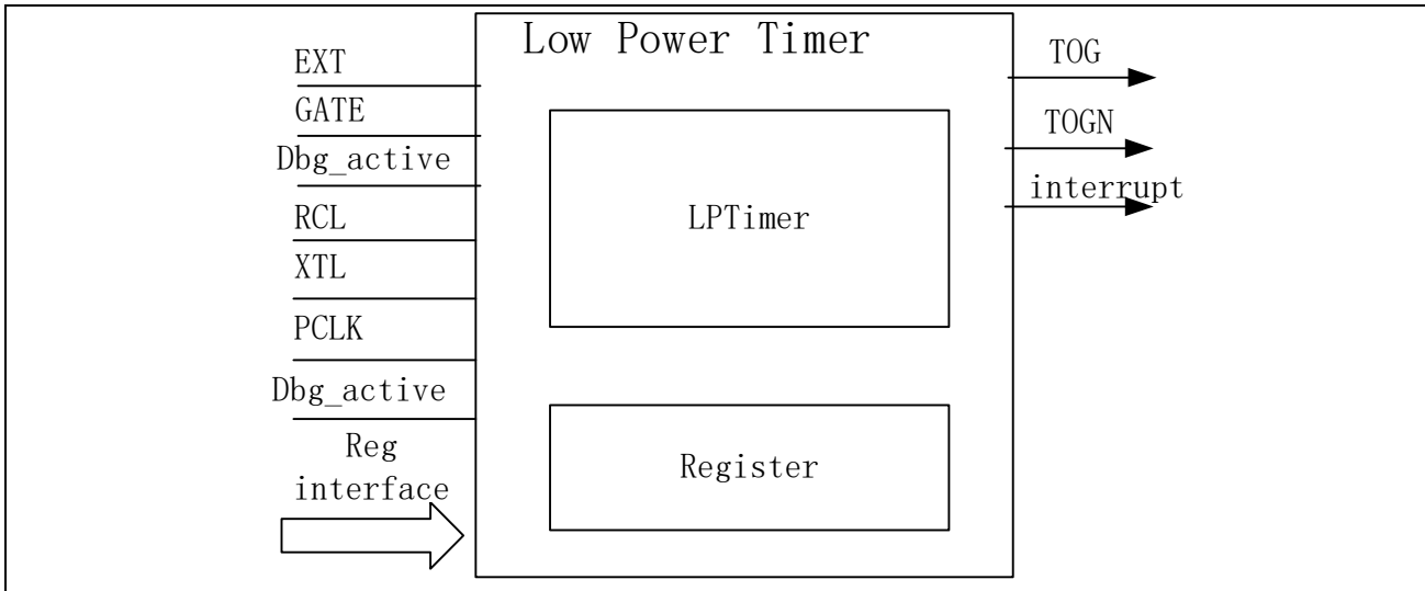
图 10-1 LPTimer 框图
