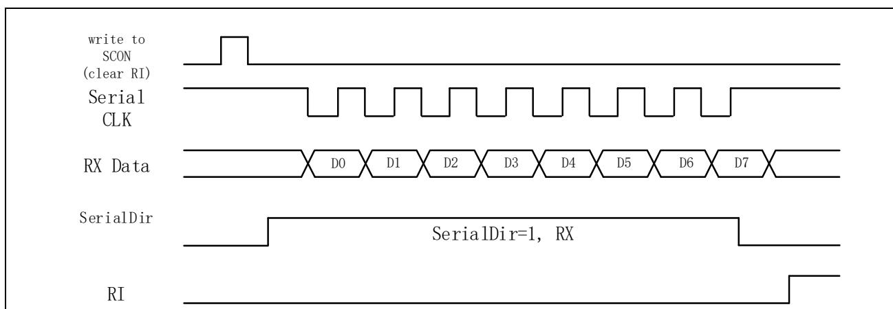
图 15-3 Mode0 接收数据
