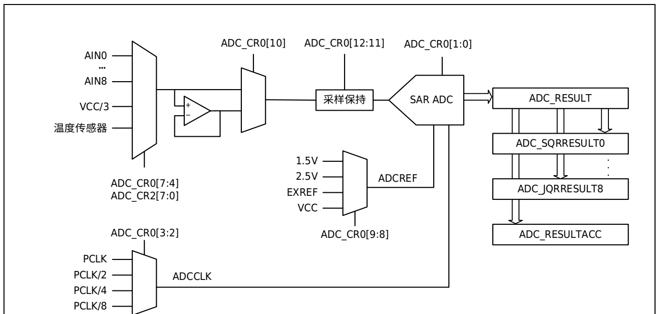
图 21-1 ADC 示意框图
