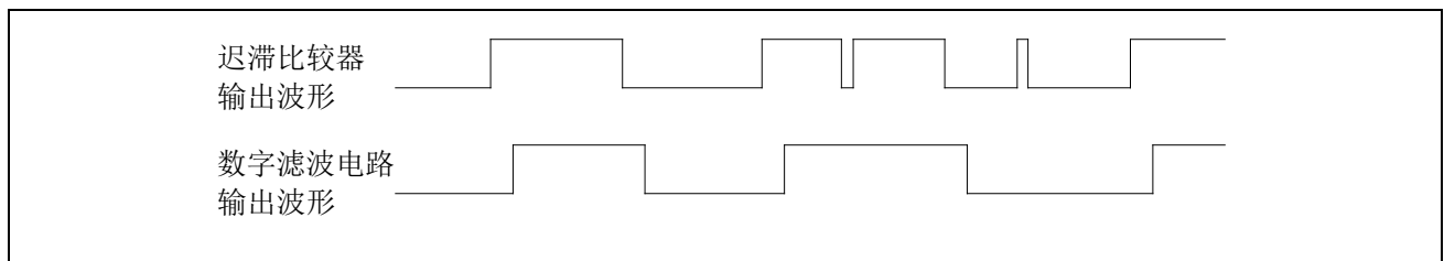
图 23-2 LVD 滤波输出
