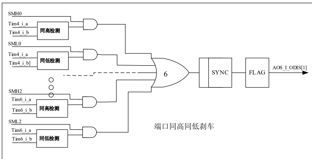
图 12-28 输出同高同低刹车示意图
