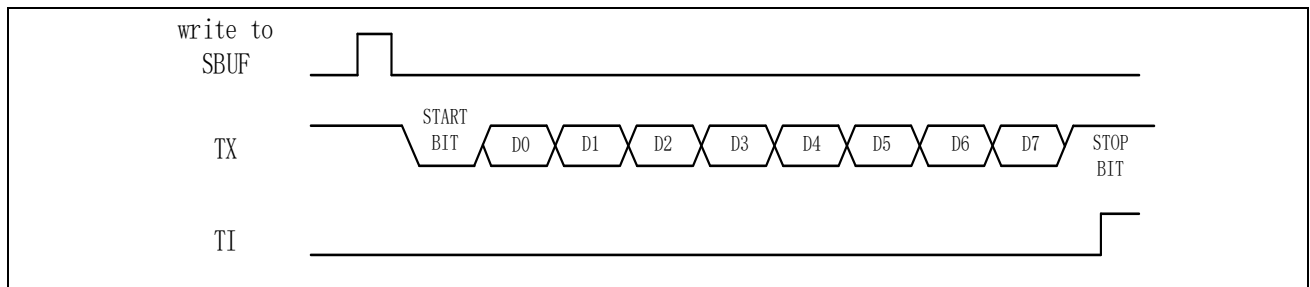
图 16-4 Mode1 发送数据
