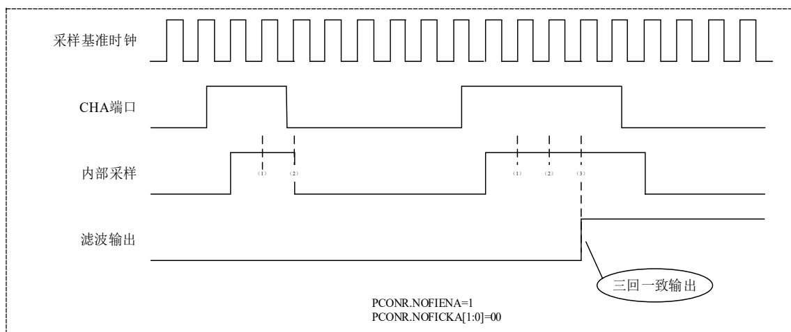
图 12-6 捕获输入端口的滤波功能
