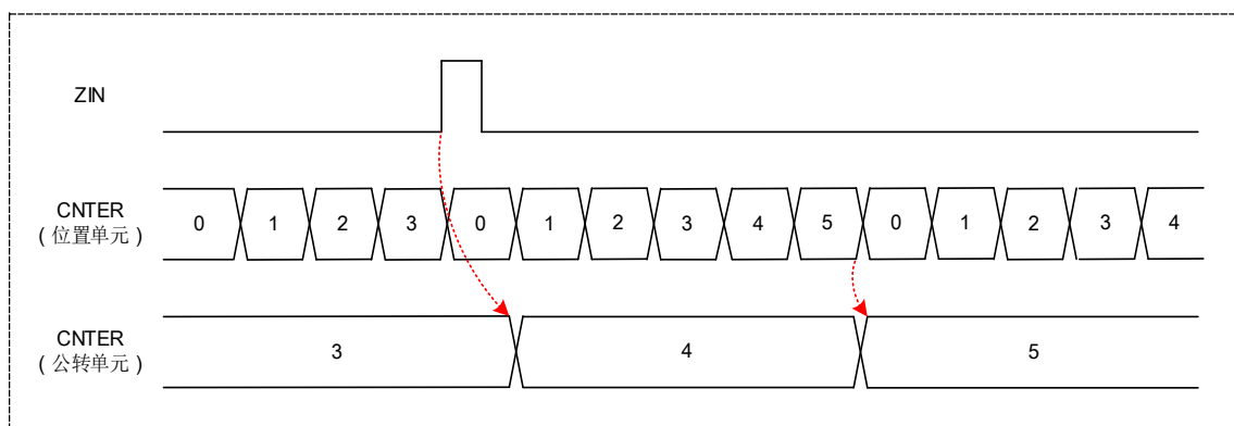
图 12-23 公转模式时 Z 相计数和位置计数器输出混合计数动作
