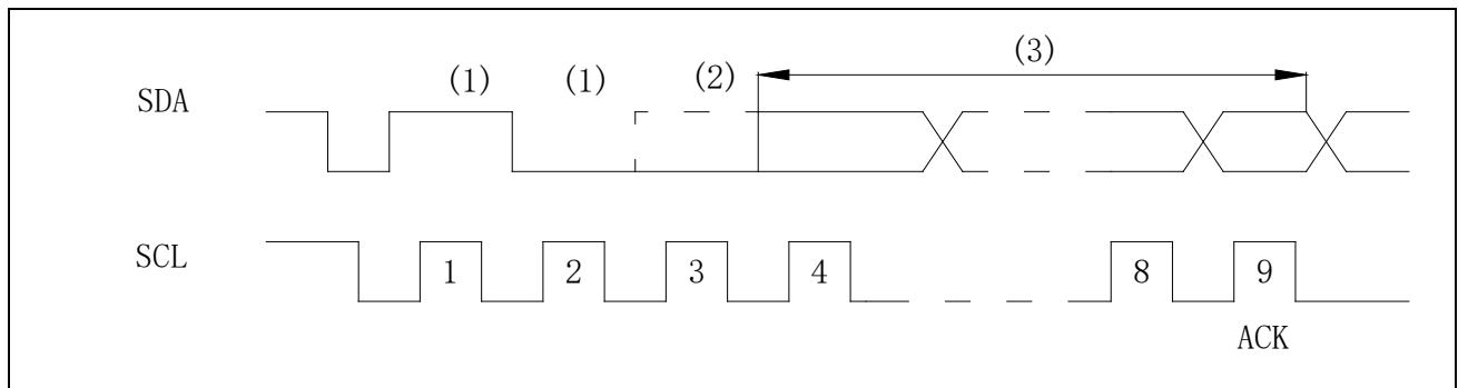
图 17-5 I2C 总线上的仲裁
