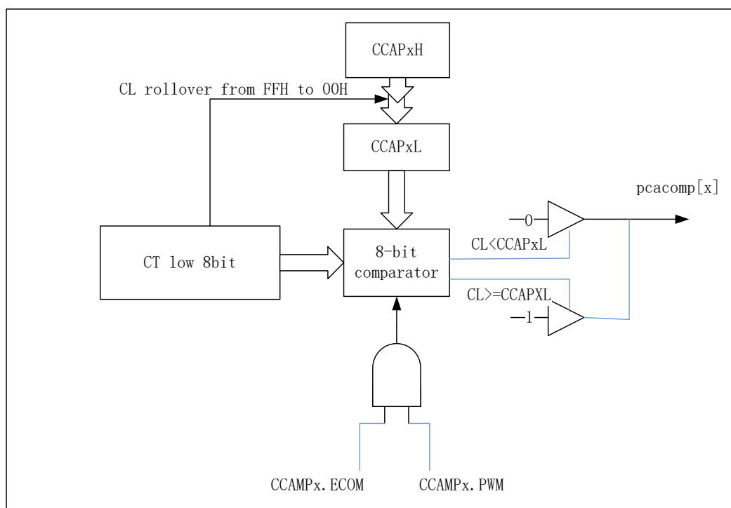
图 11-6 PCA PWM 功能框图
