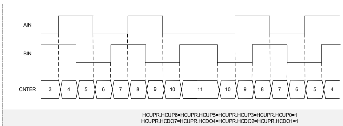
图 12-19 位置模式时相位差计数动作设定(4 倍)
