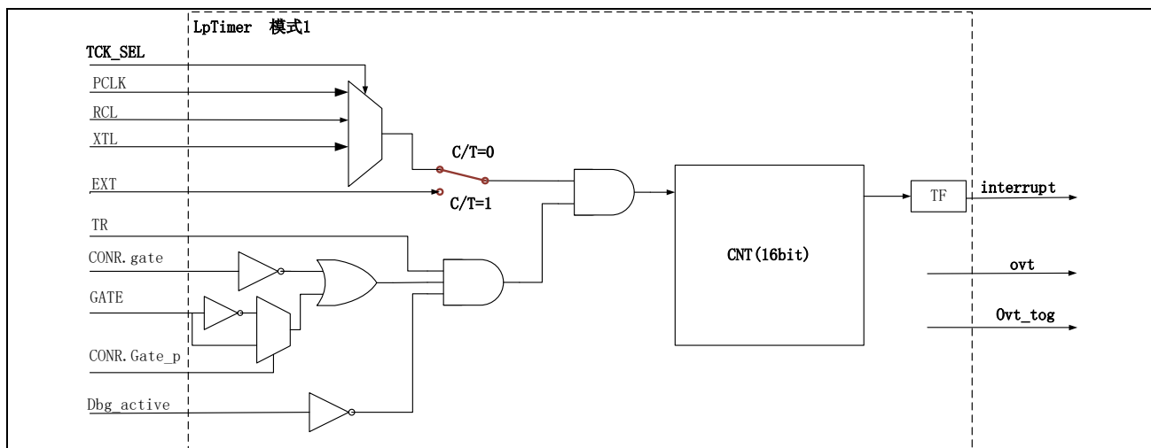
图 10-2 LpTimer 模式 1
