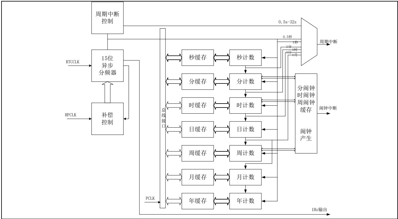
图 13-1 RTC 框图
