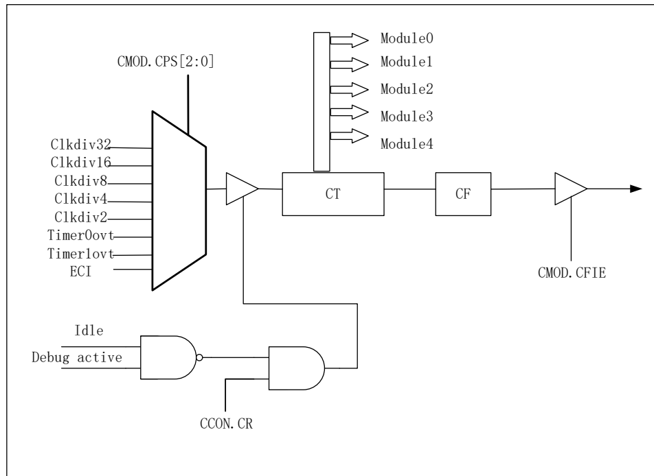
图 11-2 PCA 计数器框图
