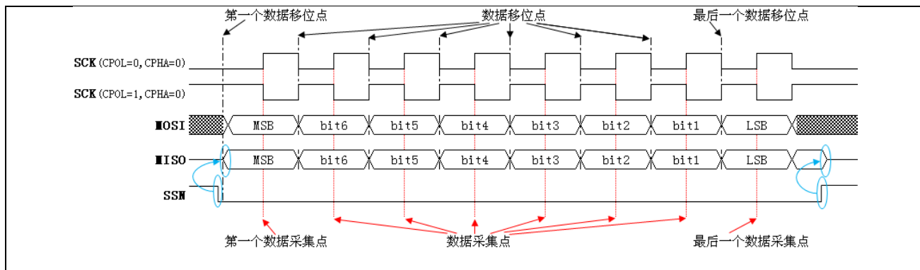
图 18-4 从机 CPHA 为 0 时数据帧格式
