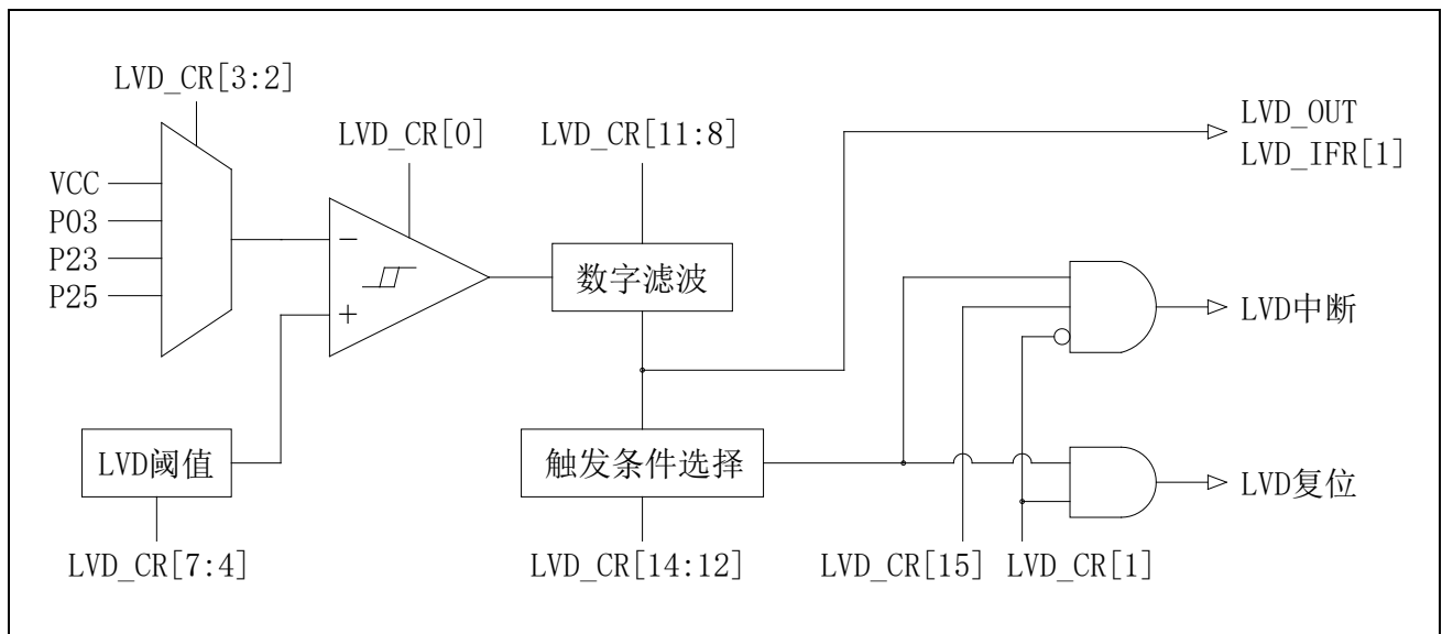
图 23-1 LVD 框图
