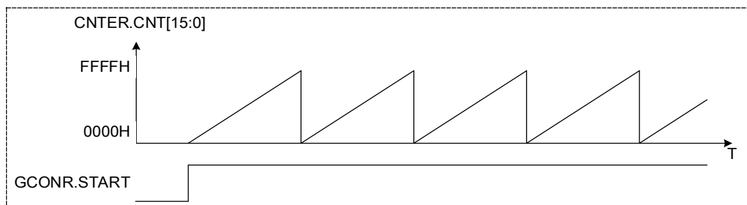
图 12-2 锯齿波波形（递加计数）
