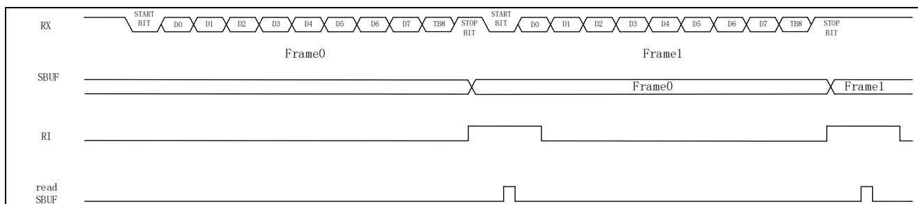
图 16-10 接收缓存
