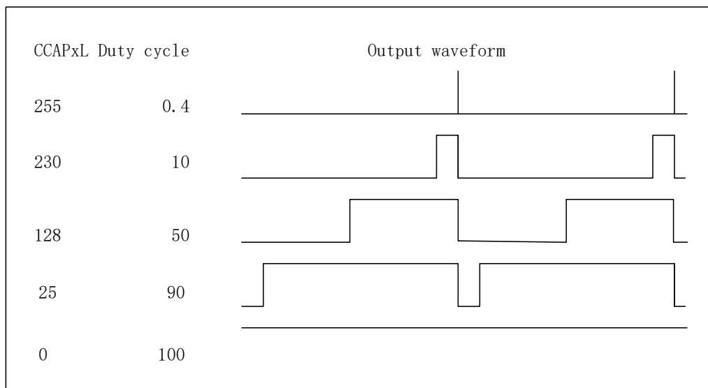
图 11-7 PCA PWM 输出波形
