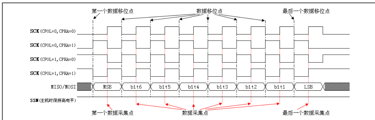
图 18-3 主机模式帧格式
