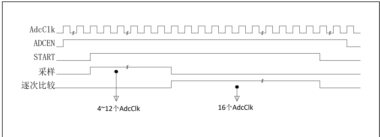
图 21-2 ADC 转换时序图
