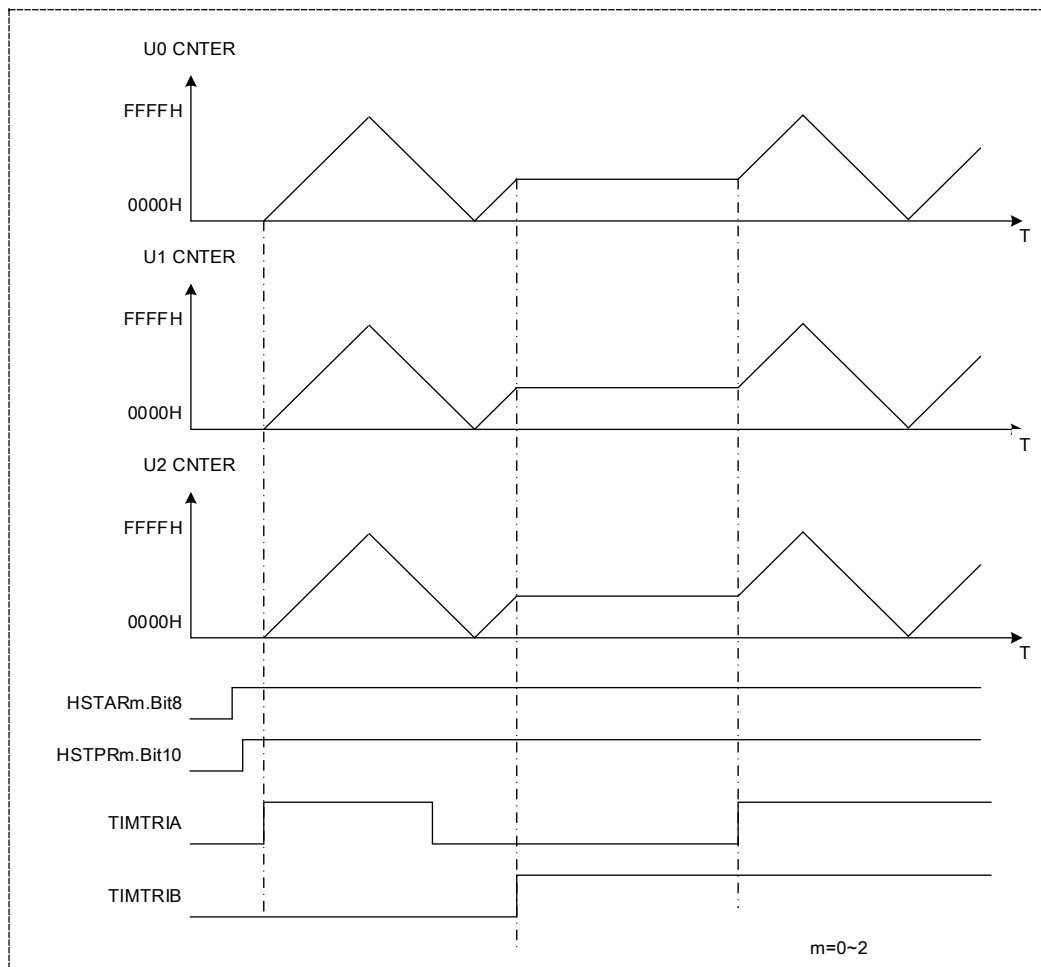
图 12-8 硬件同步动作
