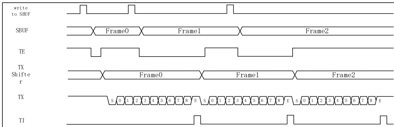
图 16-11 发送缓存
