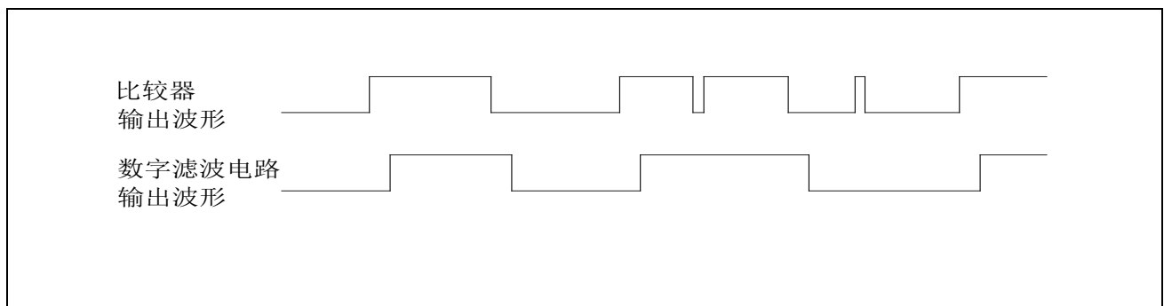
图 22-2 VC 滤波响应时间
