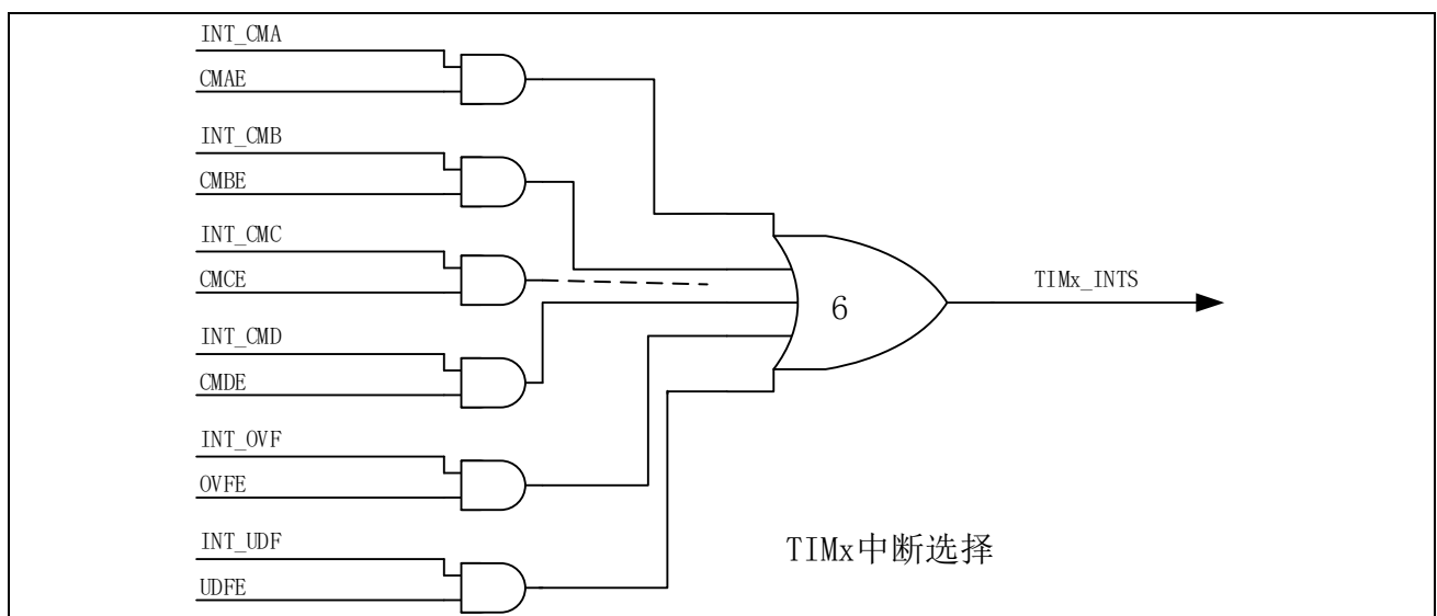
图 12-30 Timer4/5/6 中断选择
