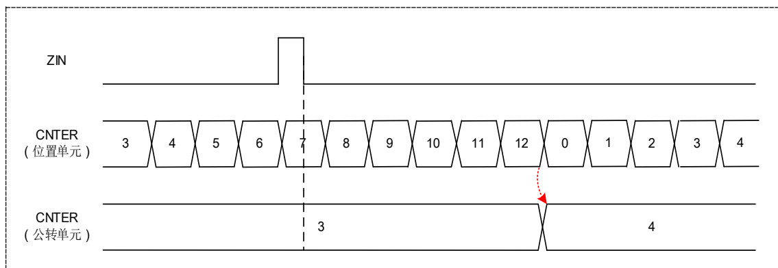
图 12-22 公转模式时位置计数器输出计数动作
