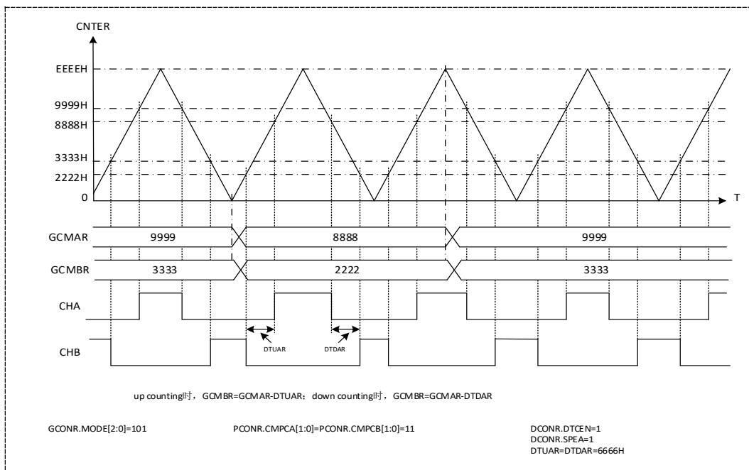
图 11-13 三角波 B 模式时硬件设定 GCMBR 互补 PWM 波输出（对称死区）
