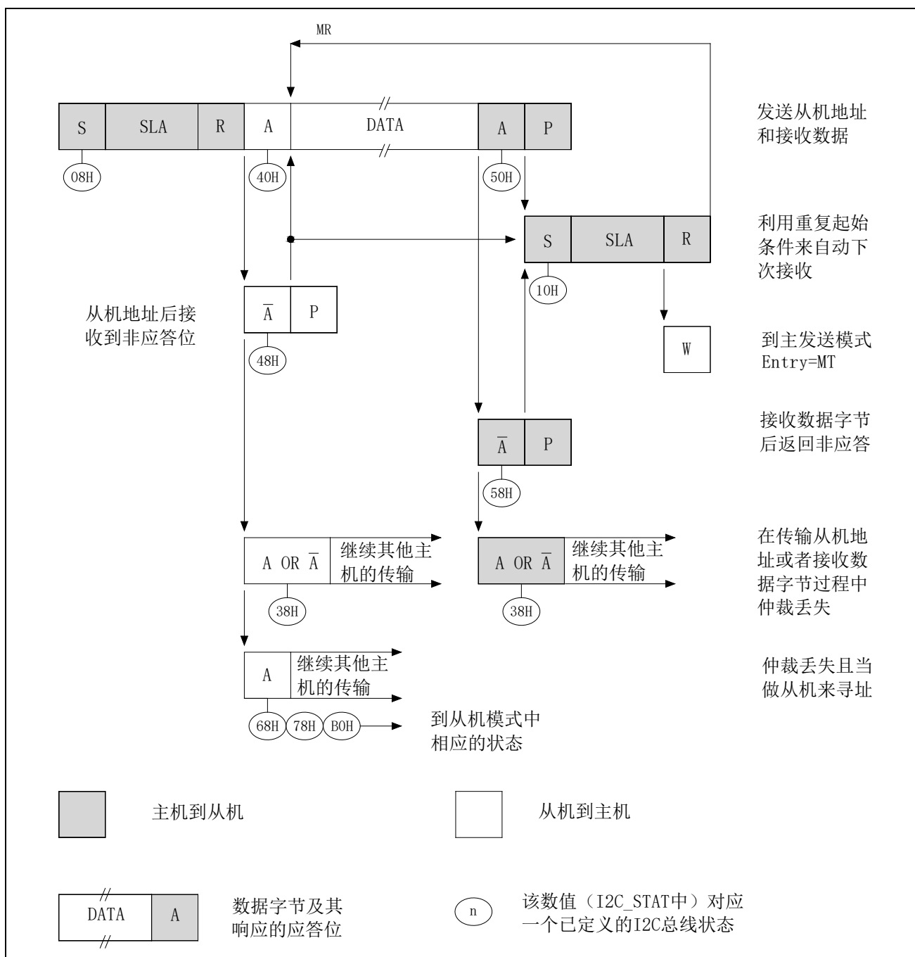
图 14-10 I2C 主机接收状态图
