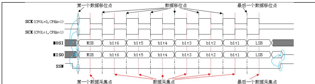
图 15-5 从机 CHPA 为 1 时数据帧格式
