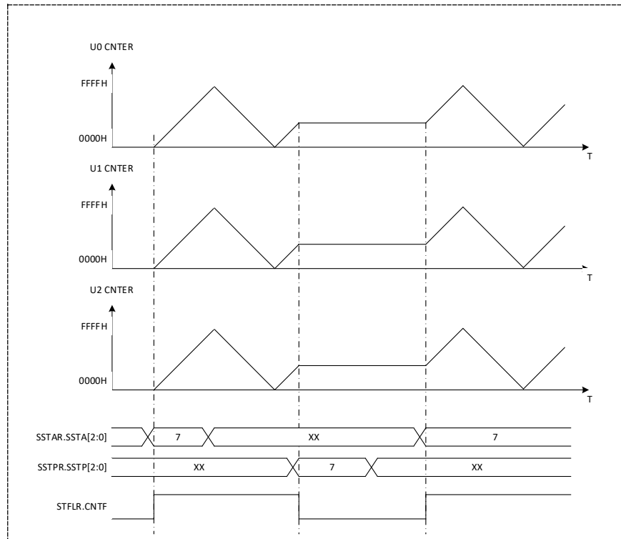
图 11-7 软件同步动作
