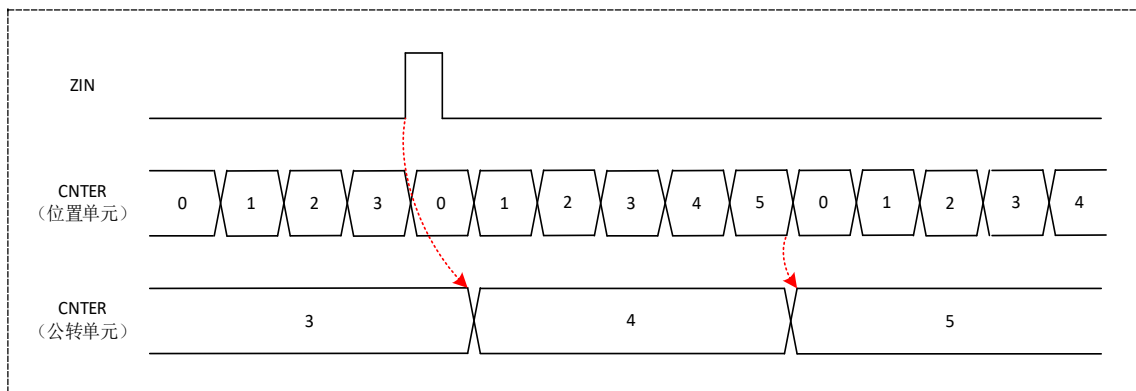
图 11-23 公转模式时 Z 相计数和位置计数器输出混合计数动作
