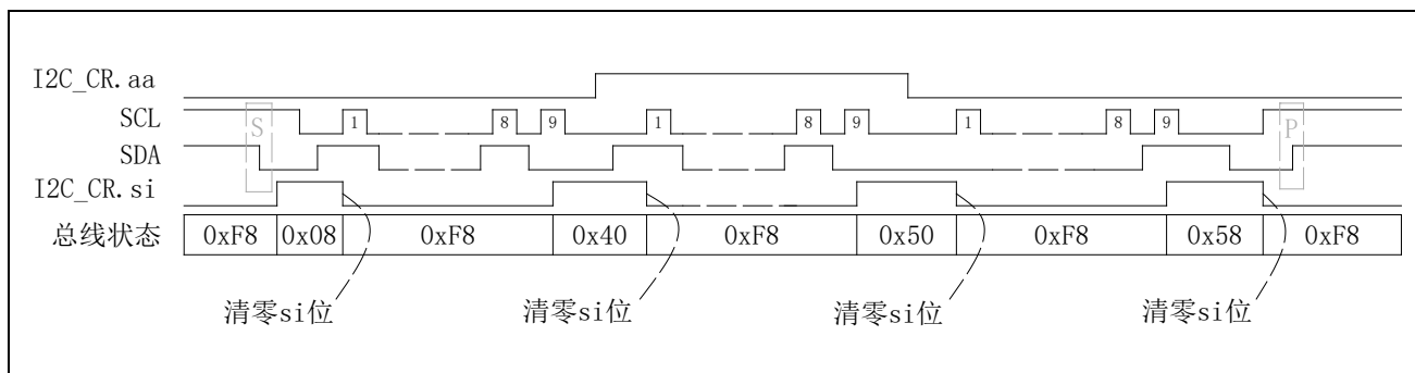
图 14-9 主接收模式数据同步图
