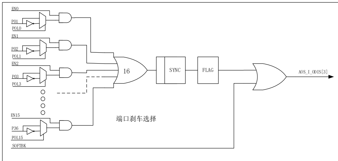
图 11-27 端口刹车与软件刹车示意图
