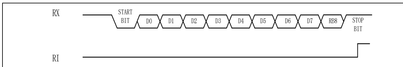
图 13-7 Mode2 接收数据
