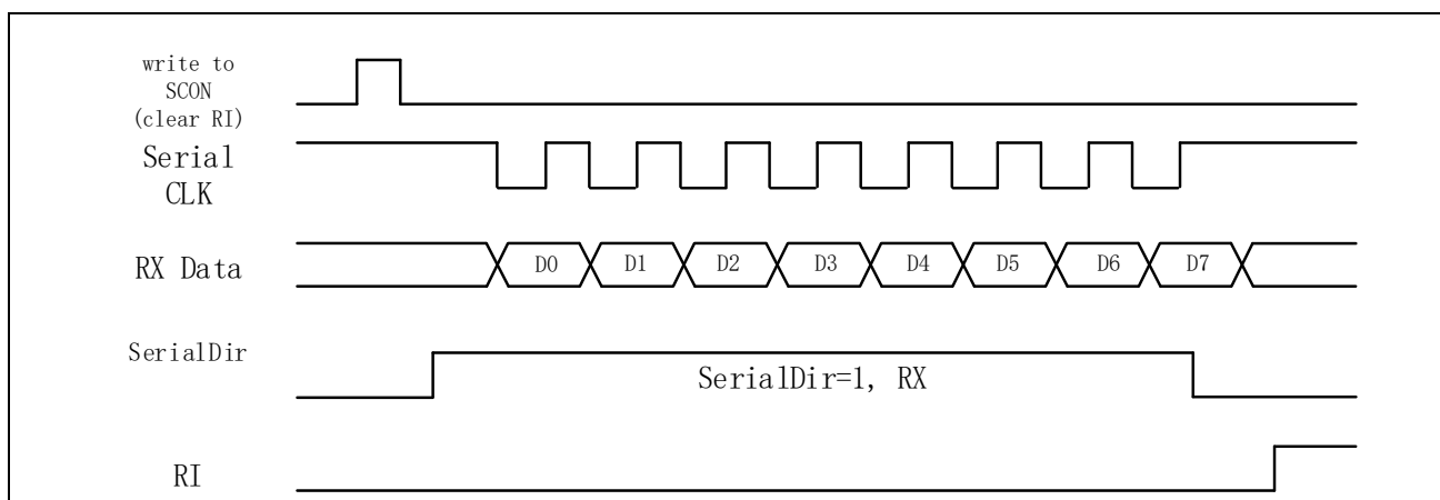
图 13-3 Mode0 接收数据
