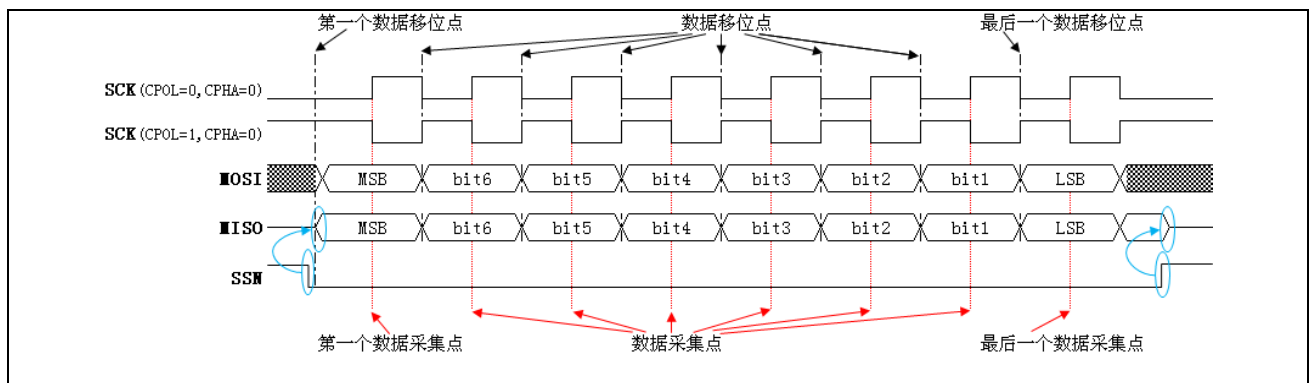
图 15-4 从机 CPHA 为 0 时数据帧格式
