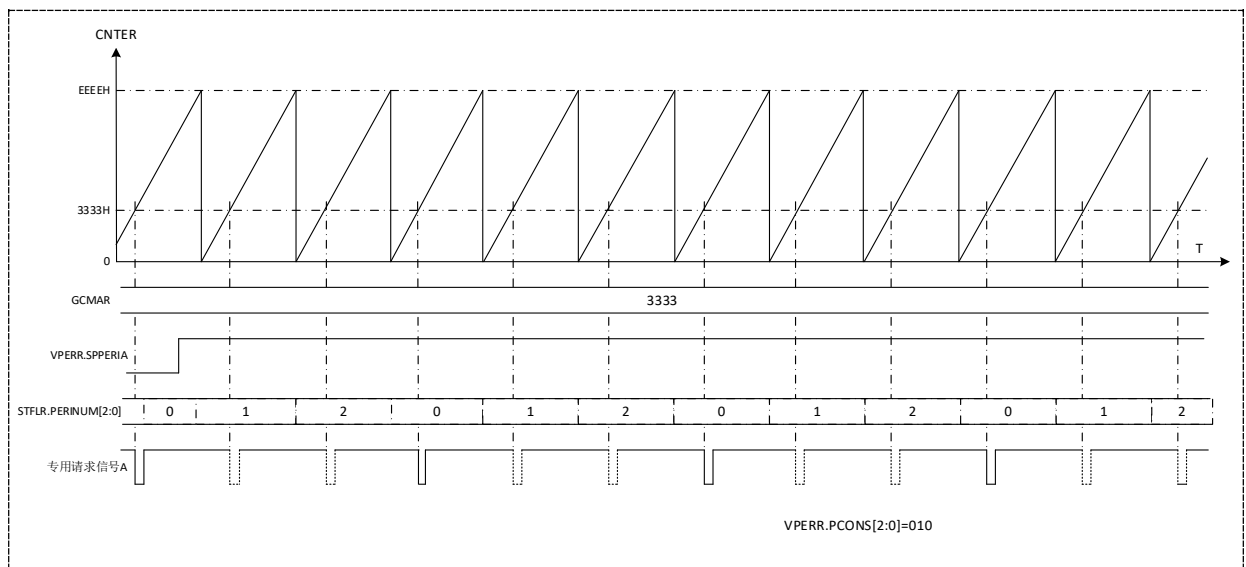
图 11-26 周期间隔有效请求信号动作
