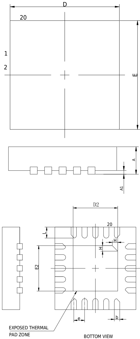
QFN20 封装
