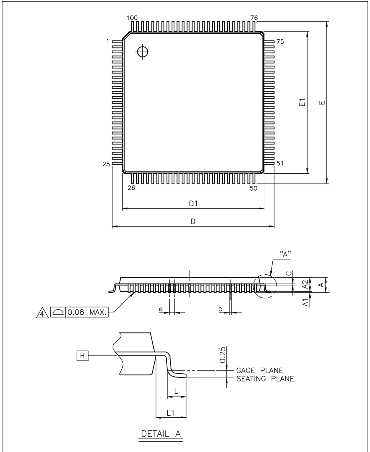
图 61. LQFP100 – 14 x 14 mm 100 引脚薄型正方扁平封装图
