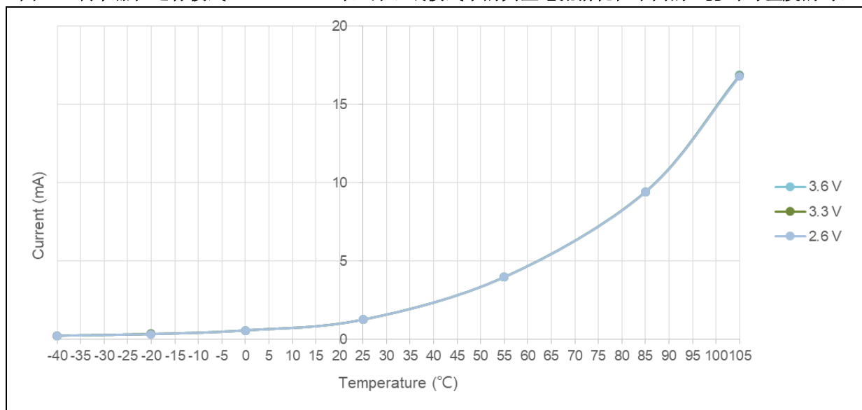
图 11. 调节器在运行模式, LDO 1.2V 时, 深睡眠模式下的典型电流消耗在不同的 V DD 时与温度的对比
