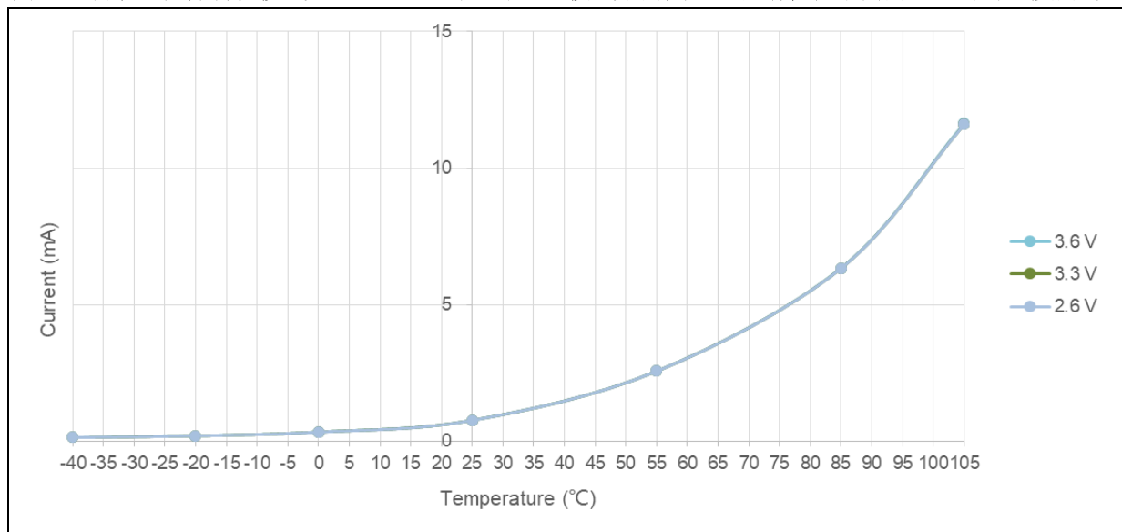
图 12. 调节器在低功耗模式, LDO 1.1V 时, 深睡眠模式下的典型电流消耗在不同的 V DD 时与温度的对比
