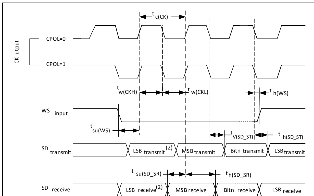
图 45. I 2 S 从模式时序图 (Philips 协议)
