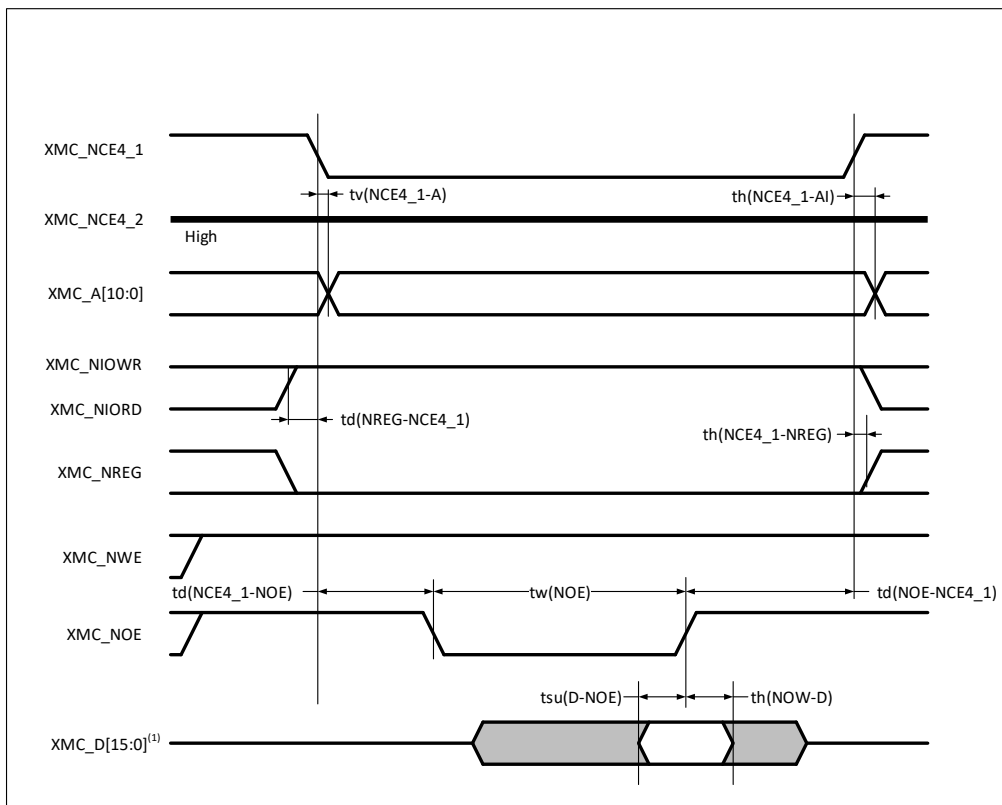
图 36. 属性存储空间读操作的 PC 卡/CF 卡控制器波形
