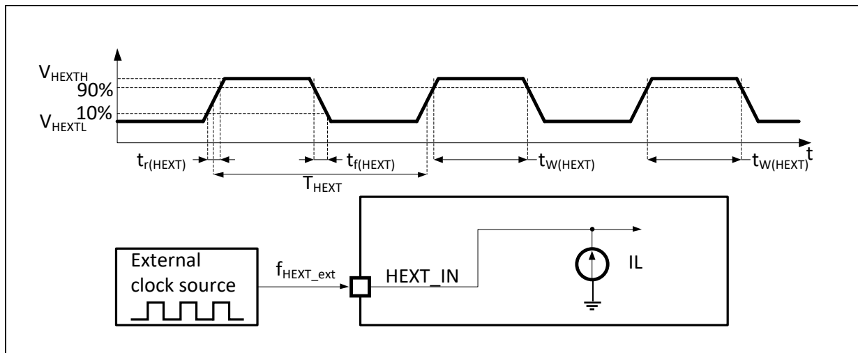
图 17. 外部高速时钟源的交流时序图
