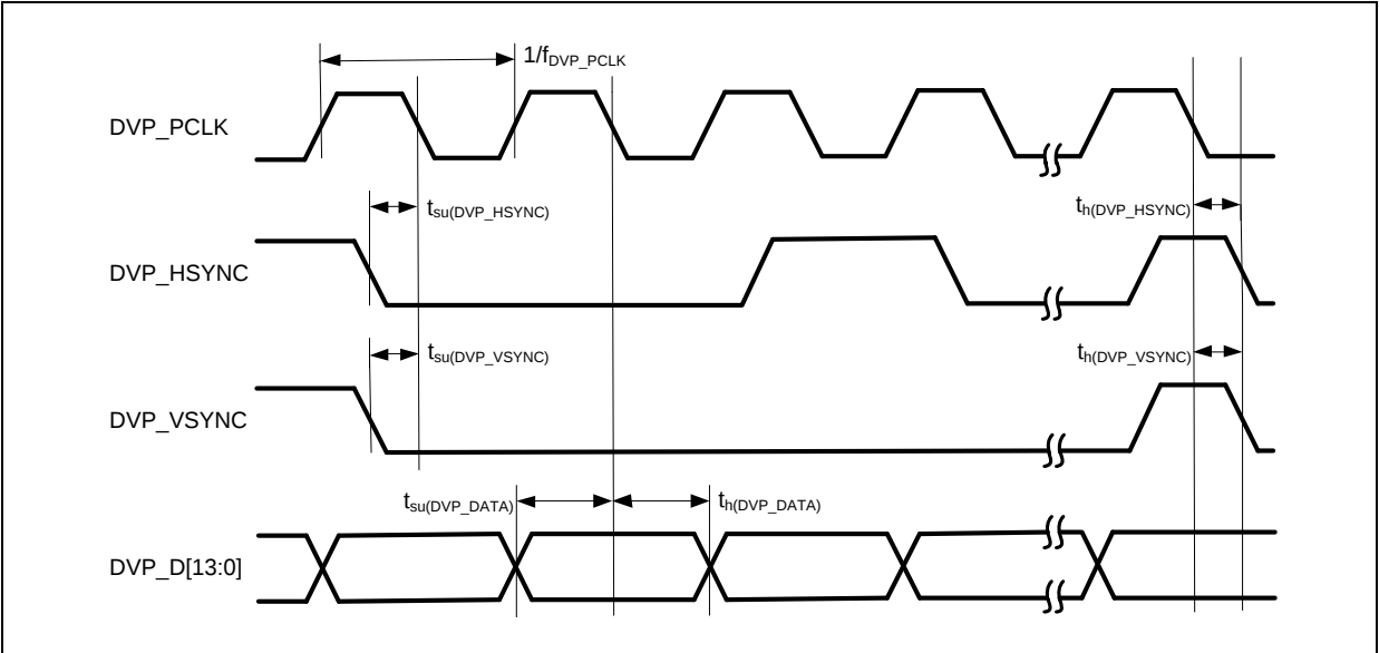
图 54. DVP 时序图
