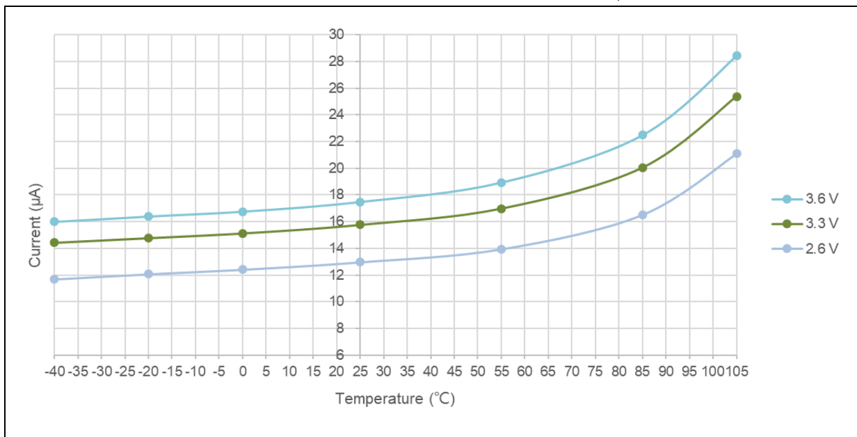
图 14. 待机模式下的典型电流消耗在不同的 V_{DD} 时与温度的对比 (AT32F435/437xD 外其它型号)
