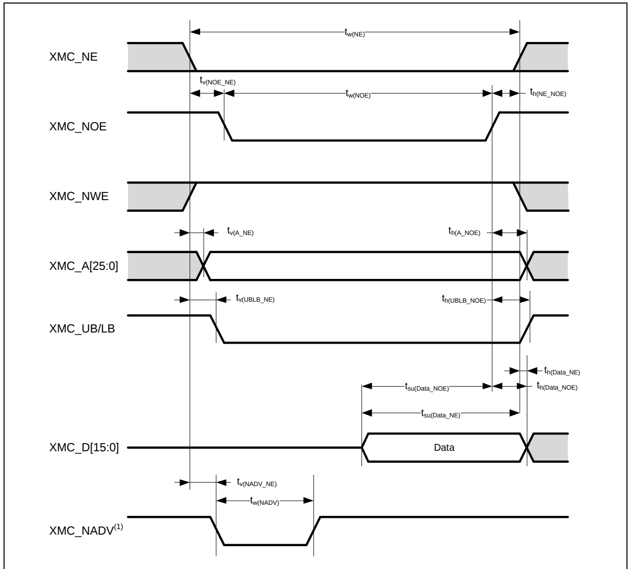
图 22. 异步非总线复用的 SRAM/PSRAM/NOR 读操作波形
