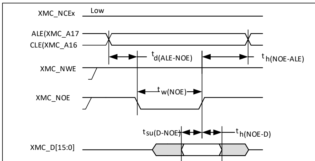
图 32. NAND 控制器在通用存储空间的读操作波形
