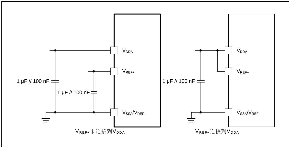
图 57. 供电电源和参考电源去耦线路（具有外部 V_{REF+} 引脚封装）
