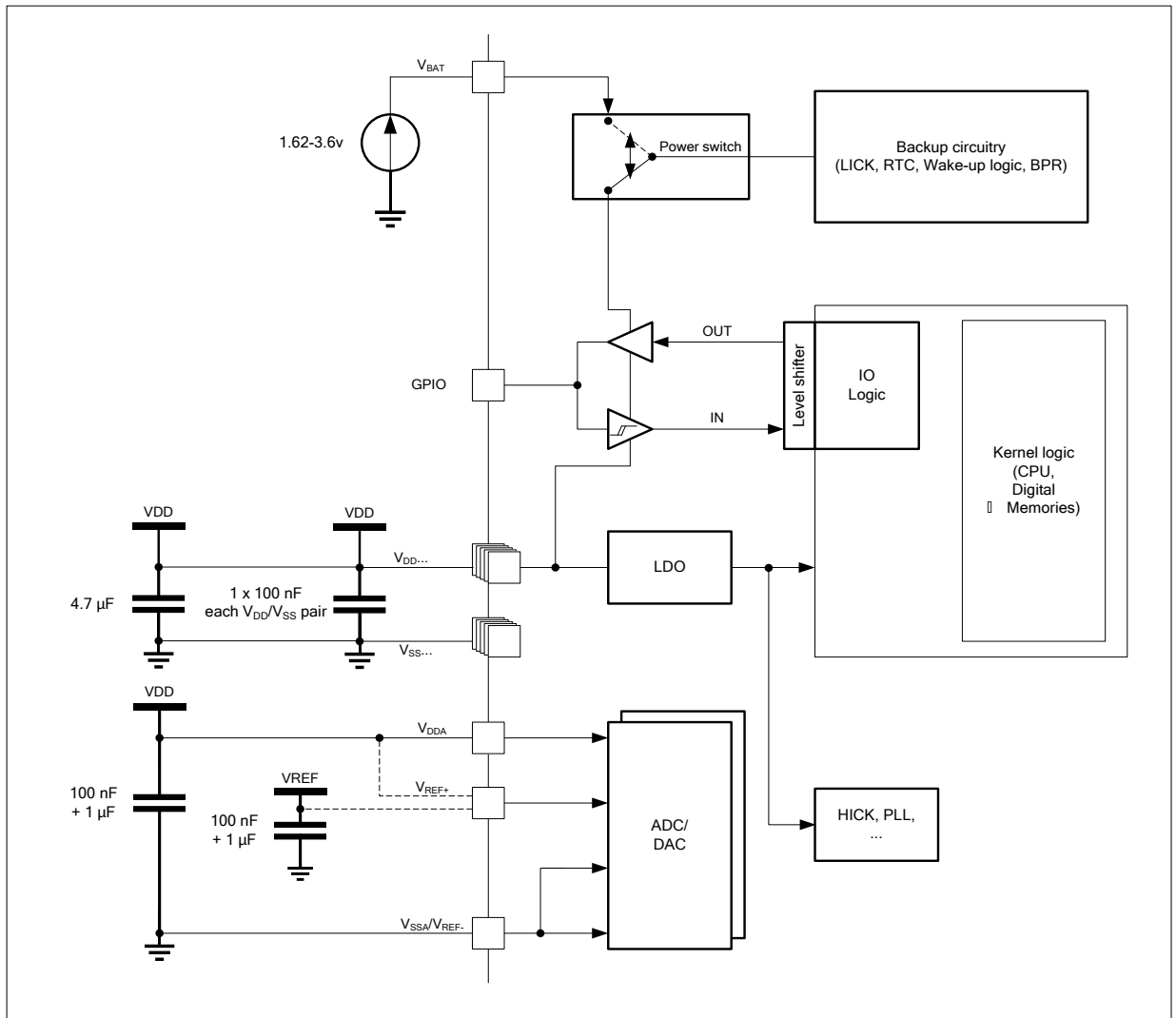
图 9. 供电方案
