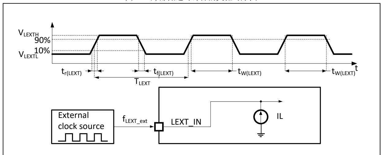
图 19. 外部低速时钟源的交流时序图
