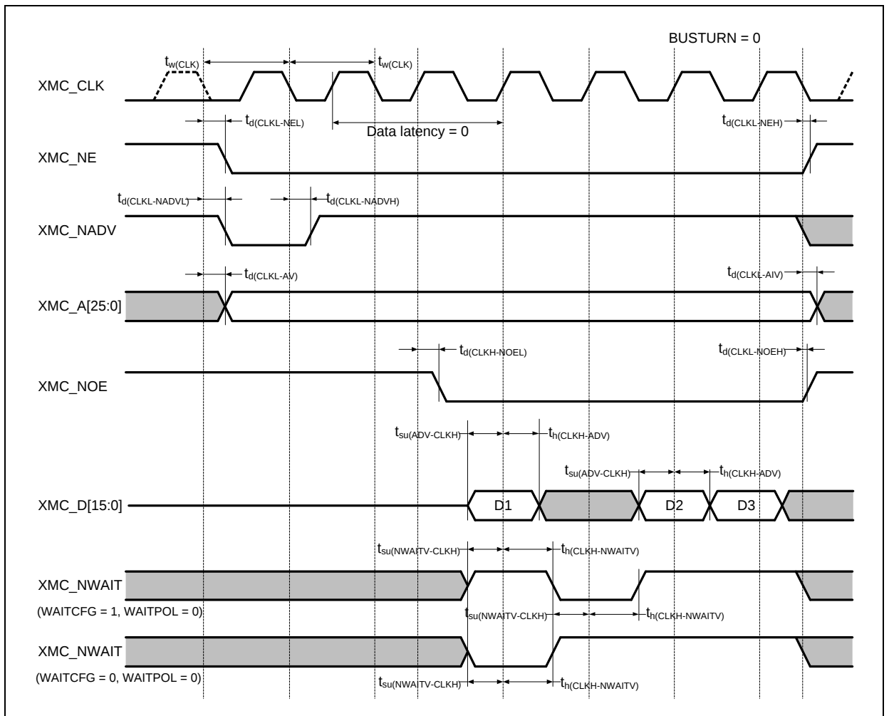
图 26. 同步非总线复用 PSRAM/NOR 读操作波形
