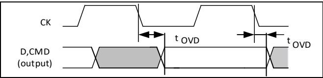
图 49. SD 默认模式
