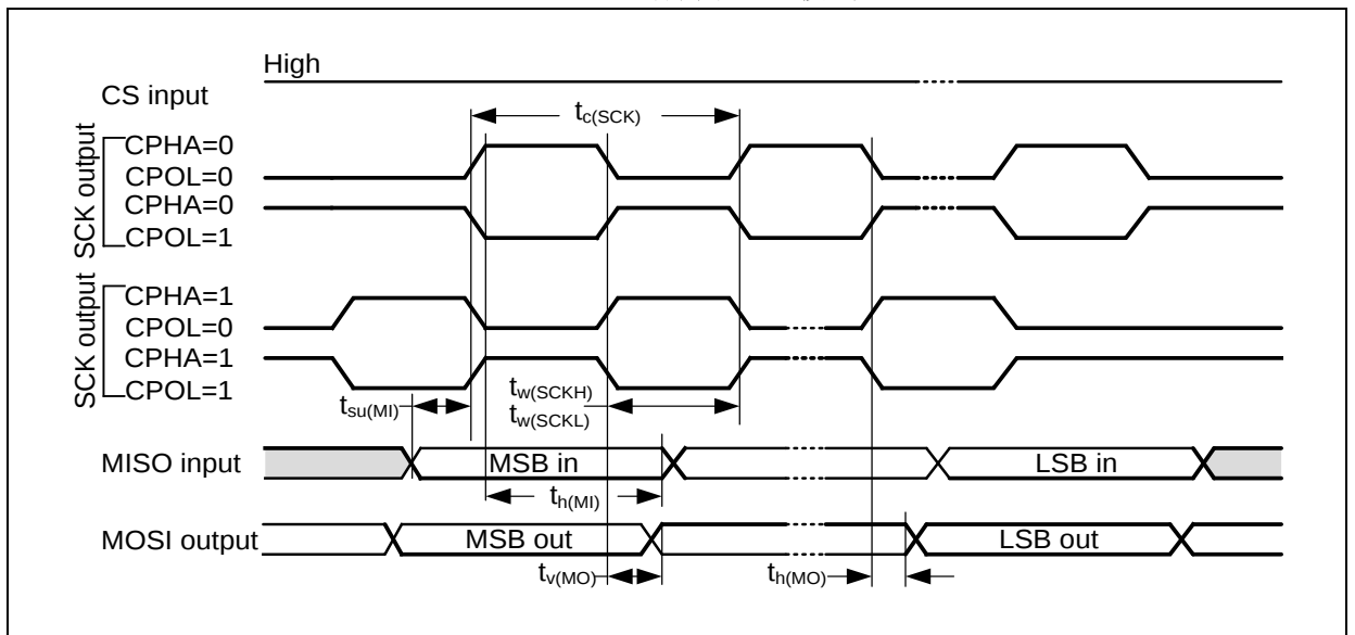
图 44. SPI 时序图 - 主模式
