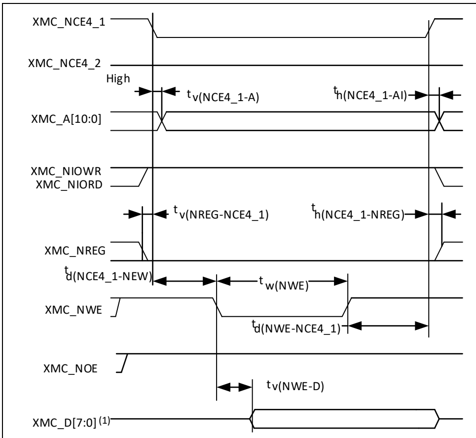
图 37. 属性存储空间写操作的 PC 卡/CF 卡控制器波形
