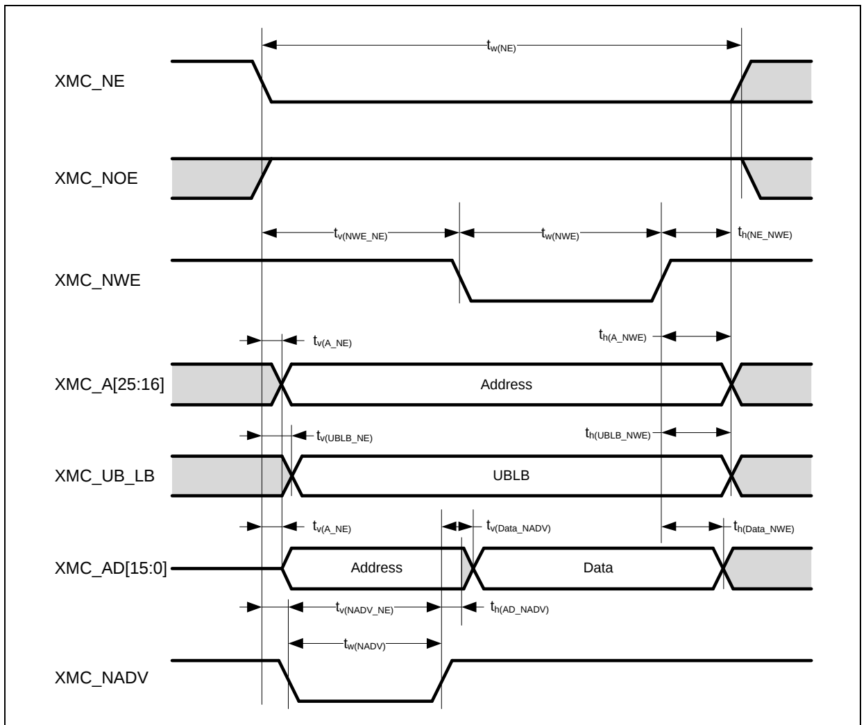
图 25. 异步总线复用 PSRAM/NOR 写操作波形
