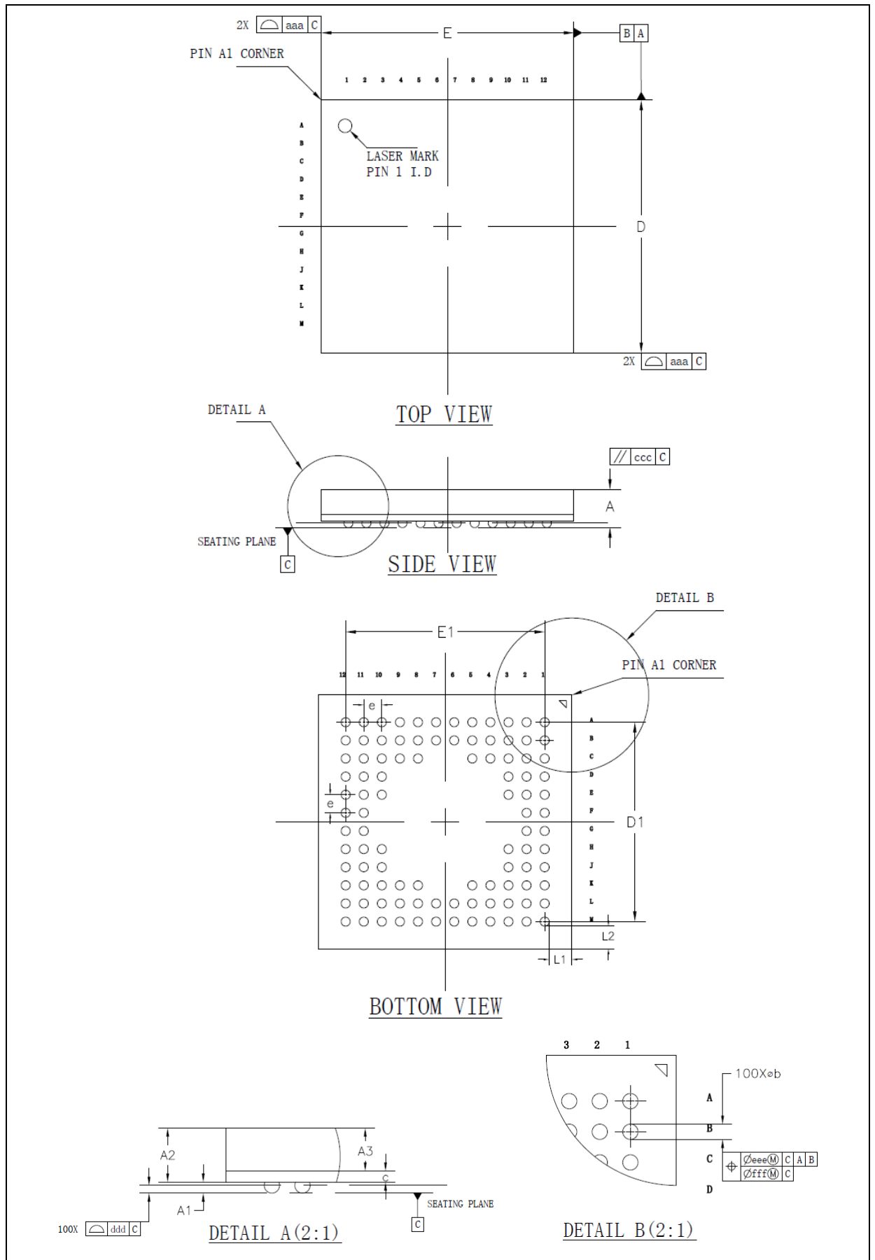
图 62. BGA100 – 7 x 7 mm 100 焊球阵列封装图
