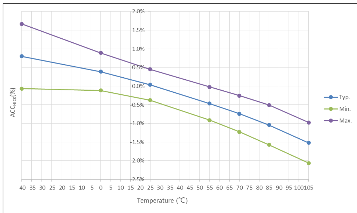
图 20. HICK 时钟精度与温度的对比
