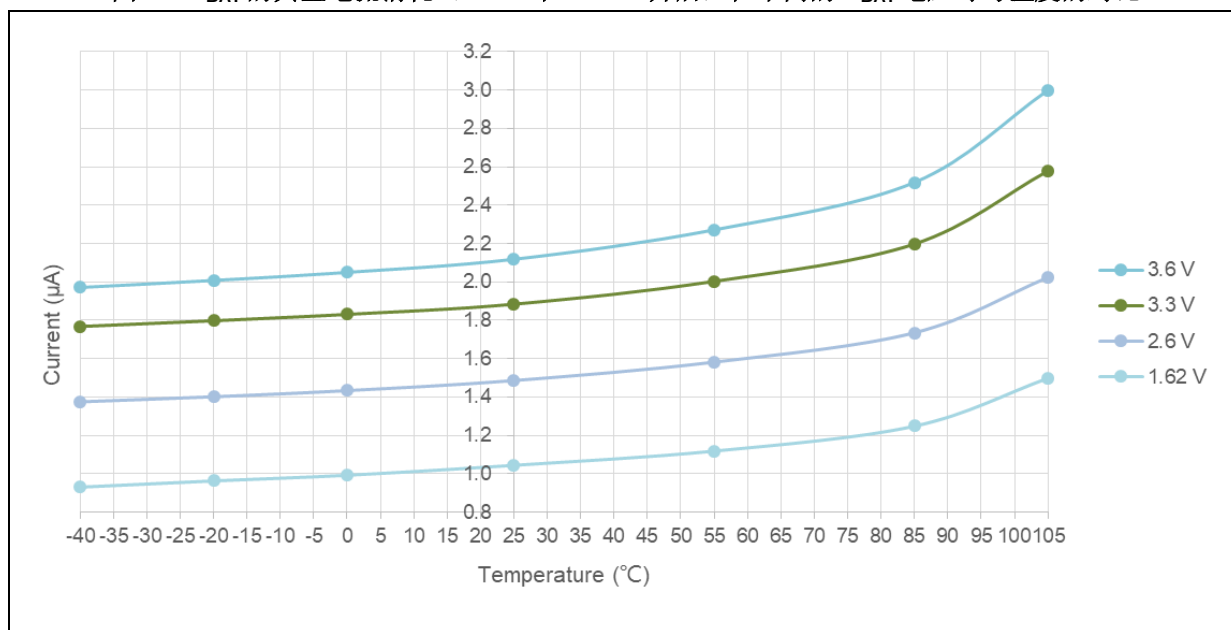
图 15. V_{BAT} 的典型电流消耗 (LEXT 和 ERTC 开启) 在不同的 V_{BAT} 电压时与温度的对比
