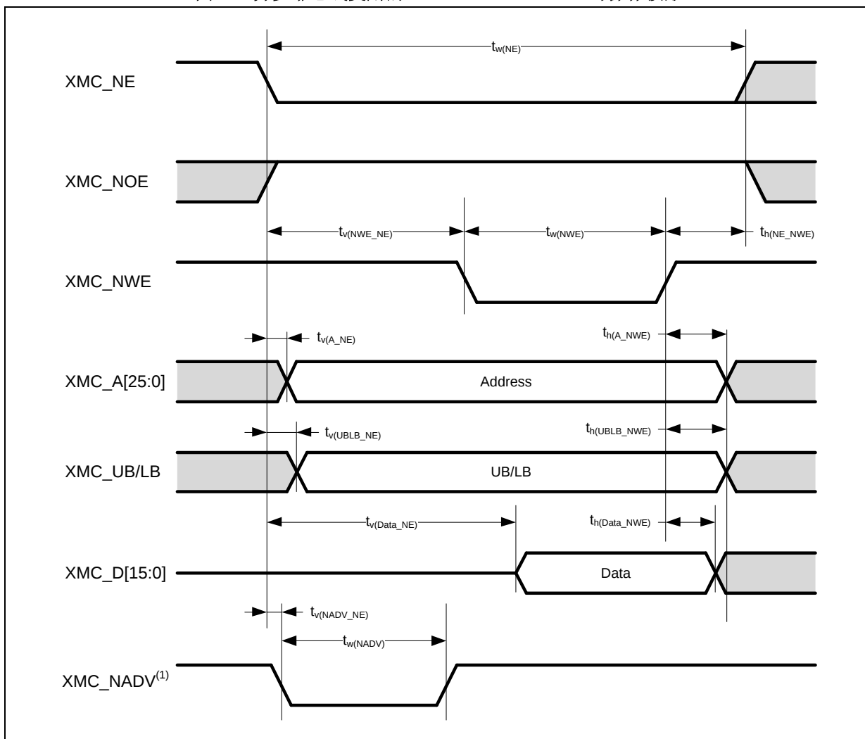
图 23. 异步非总线复用的 SRAM/PSRAM/NOR 写操作波形
