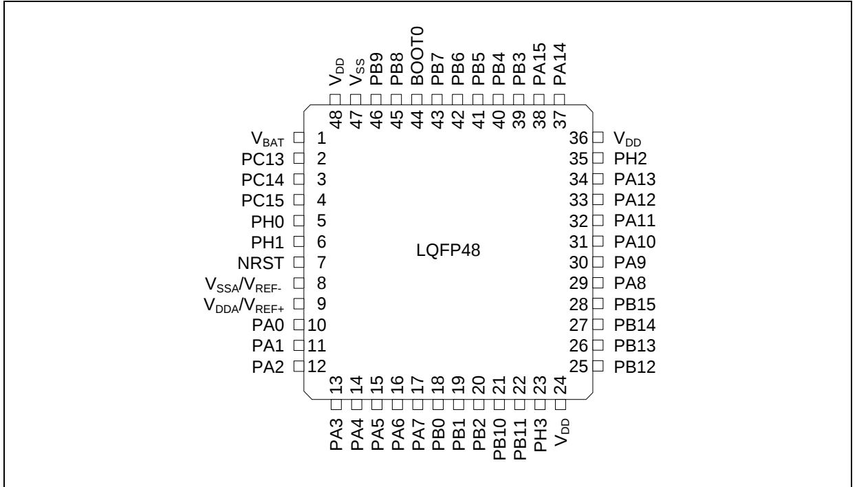
图 6. AT32F435 系列 LQFP48 引脚分布
