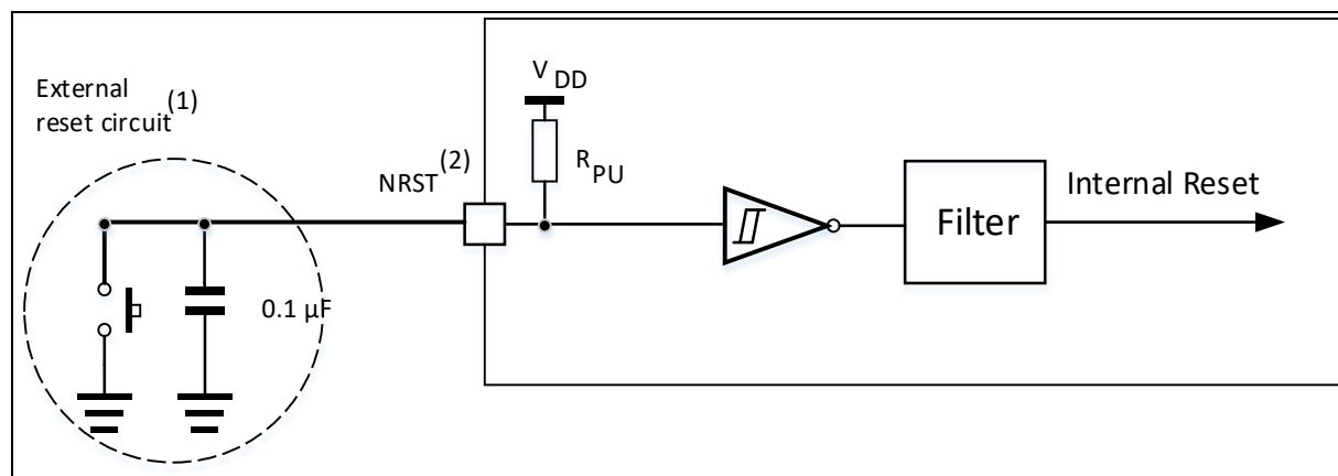
图 21. 建议的 NRST 引脚保护
