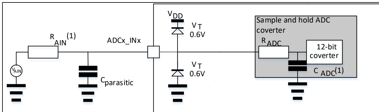
图 56. 使用 ADC 典型的连接图
