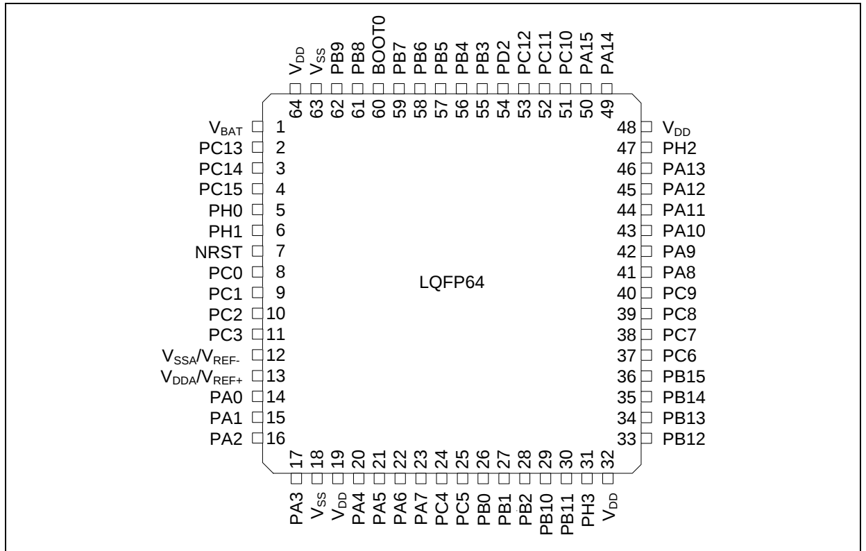
图 5. AT32F435/437 系列 LQFP64 引脚分布
