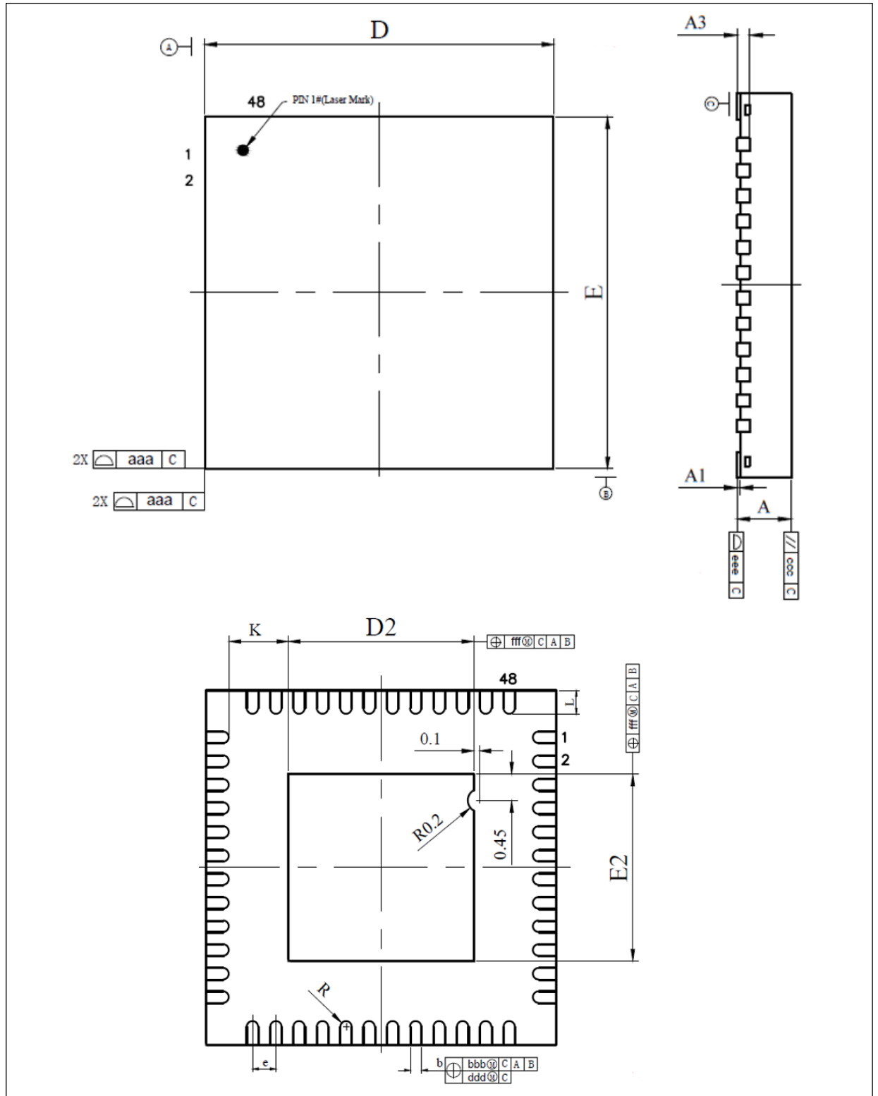
图 65. QFN48 – 6 x 6 mm 48 引脚正方扁平无引线封装图
