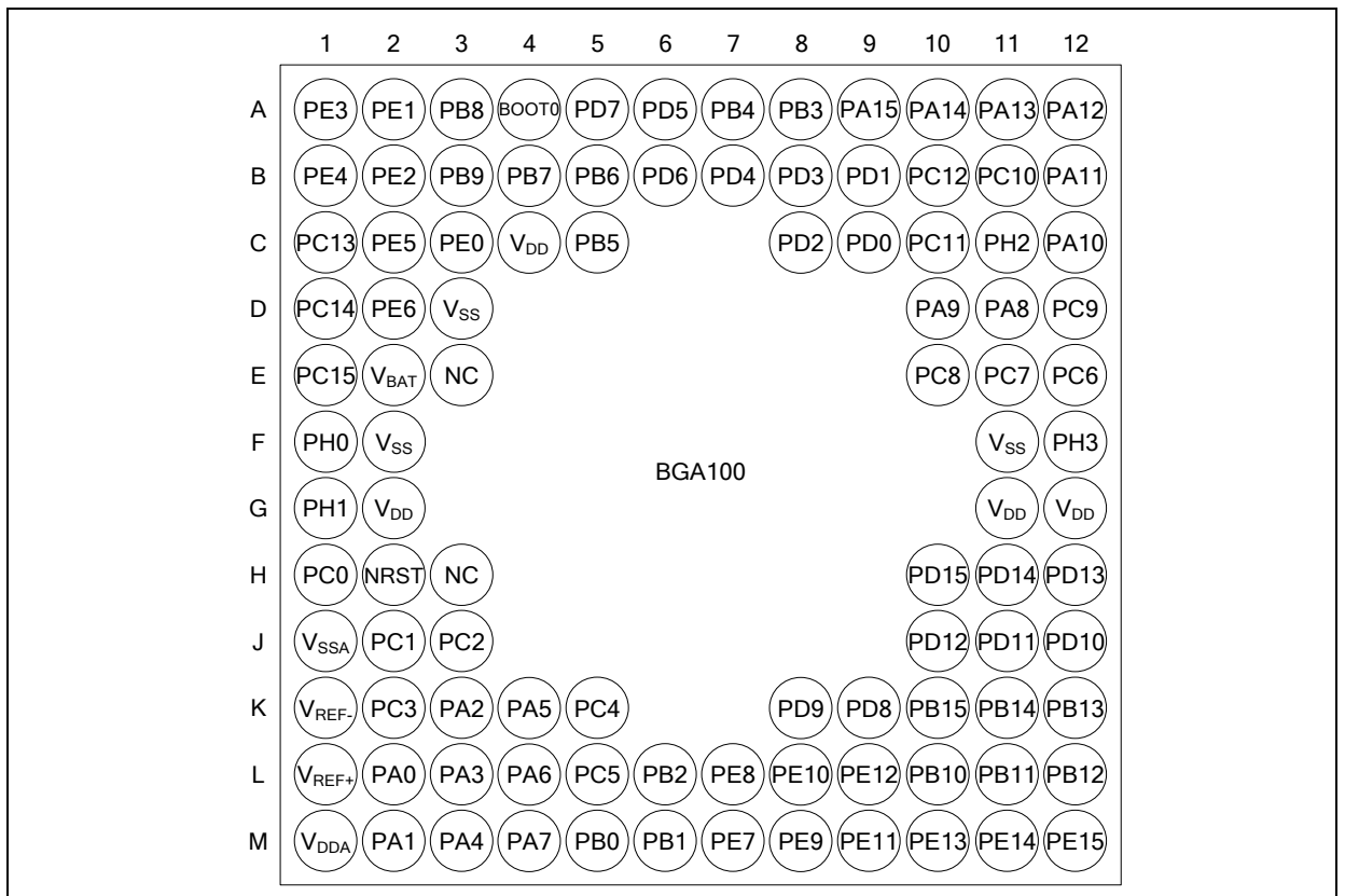
图 4. AT32F435/437 系列 BGA100 焊球布局
