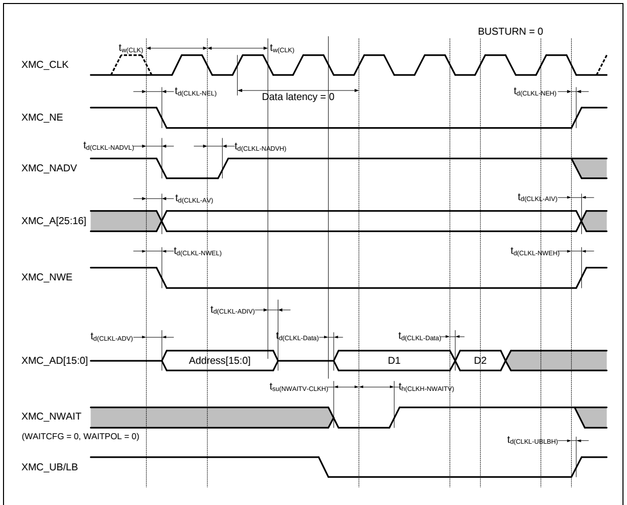
图 29. 同步总线复用 PSRAM 写操作波形
