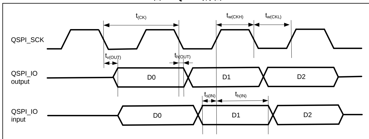
图 47. QSPI 时序图
