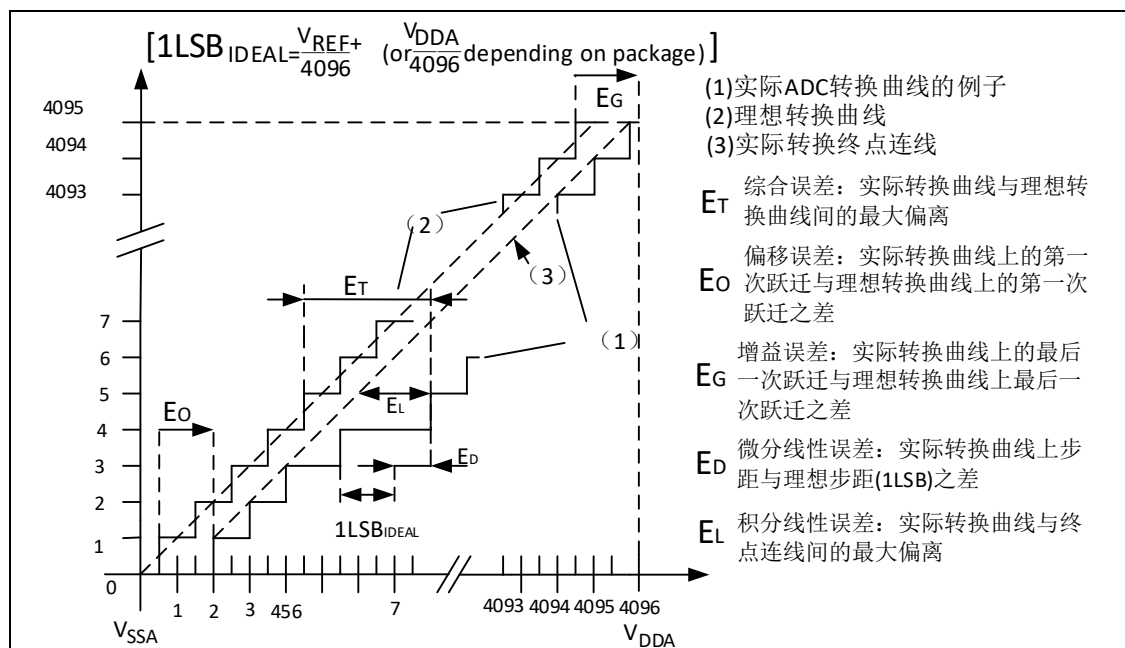
图 55. ADC 精度特性
