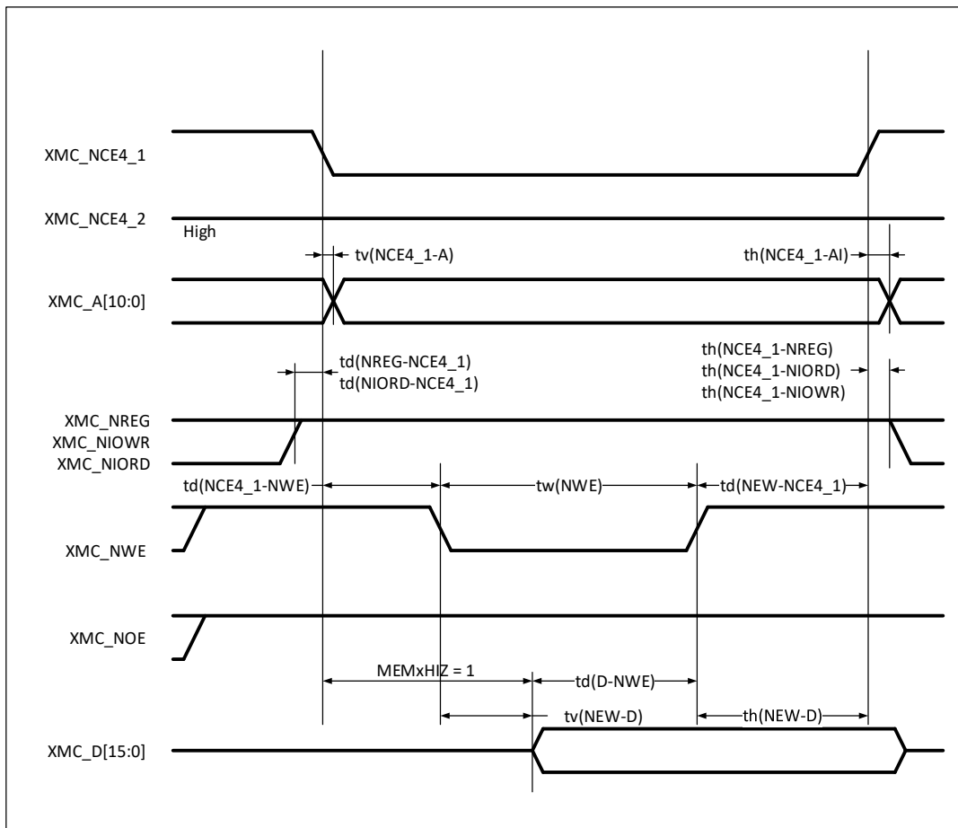
图 35. 通用存储空间写操作的 PC 卡/CF 卡控制器波形
