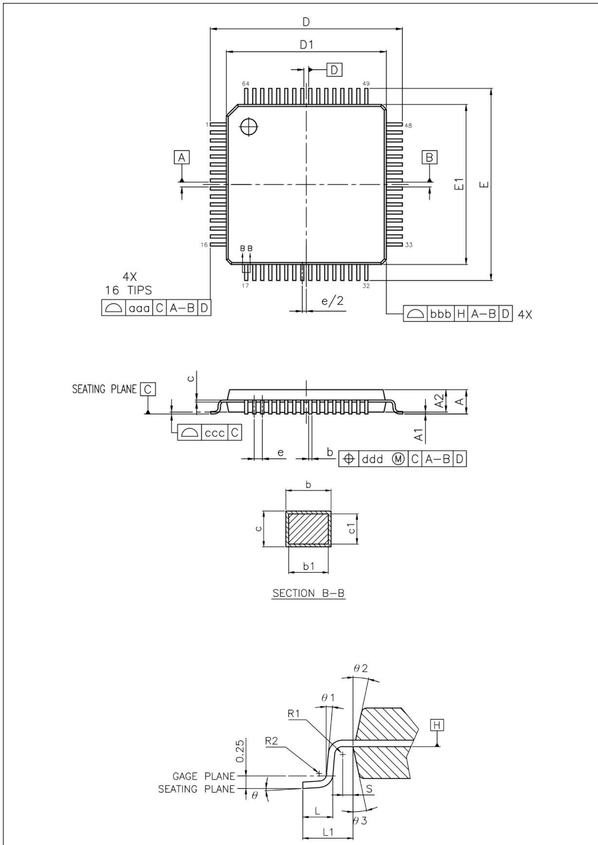
图 63. LQFP64 – 10 x 10 mm 64 引脚薄型正方扁平封装图
