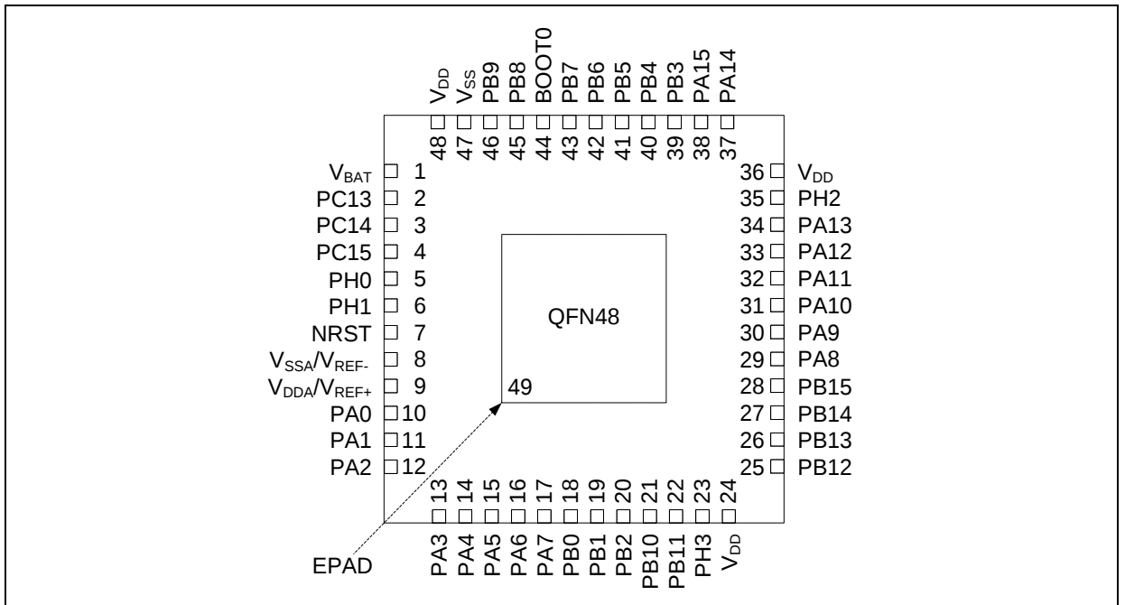
图 7. AT32F435 系列 QFN48 引脚分布
