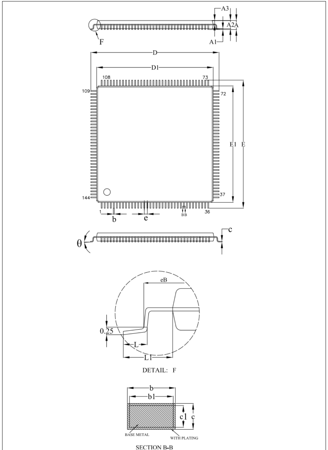
图 60. LQFP144 – 20 x 20 mm 144 引脚薄型正方扁平封装图
