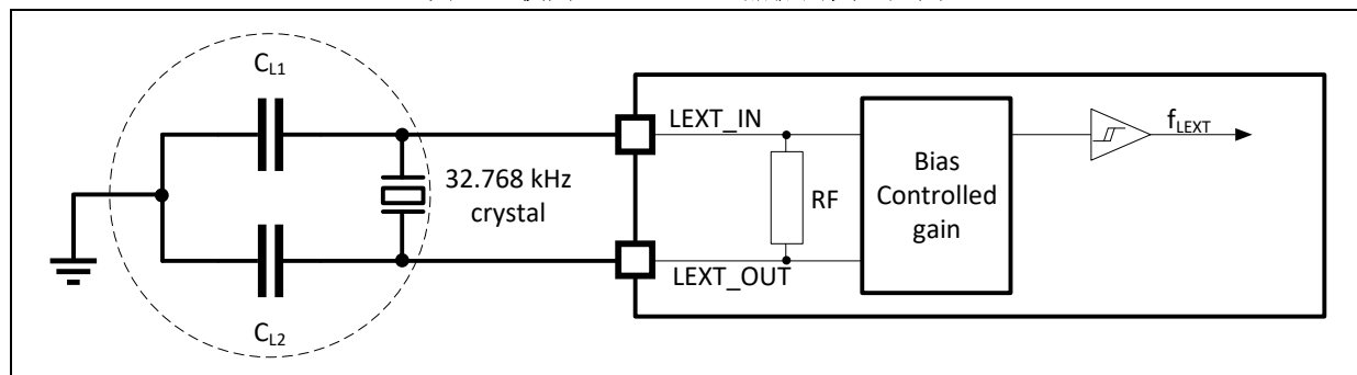
图 18. 使用 32.768 kHz 晶振的典型应用
