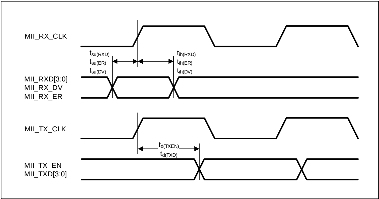
图 53. EMAC 的 MII 接口时序图
