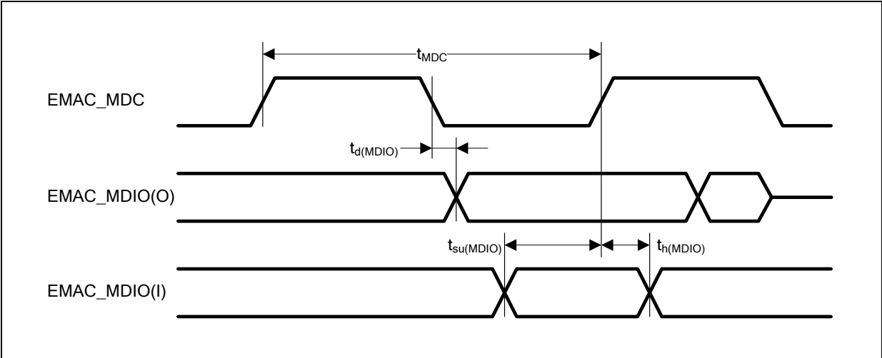
图 51. EMAC 的 SMI 接口时序图
