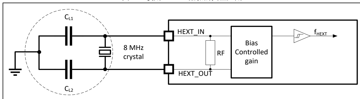
图 16. 使用 8 MHz 晶振的典型应用
