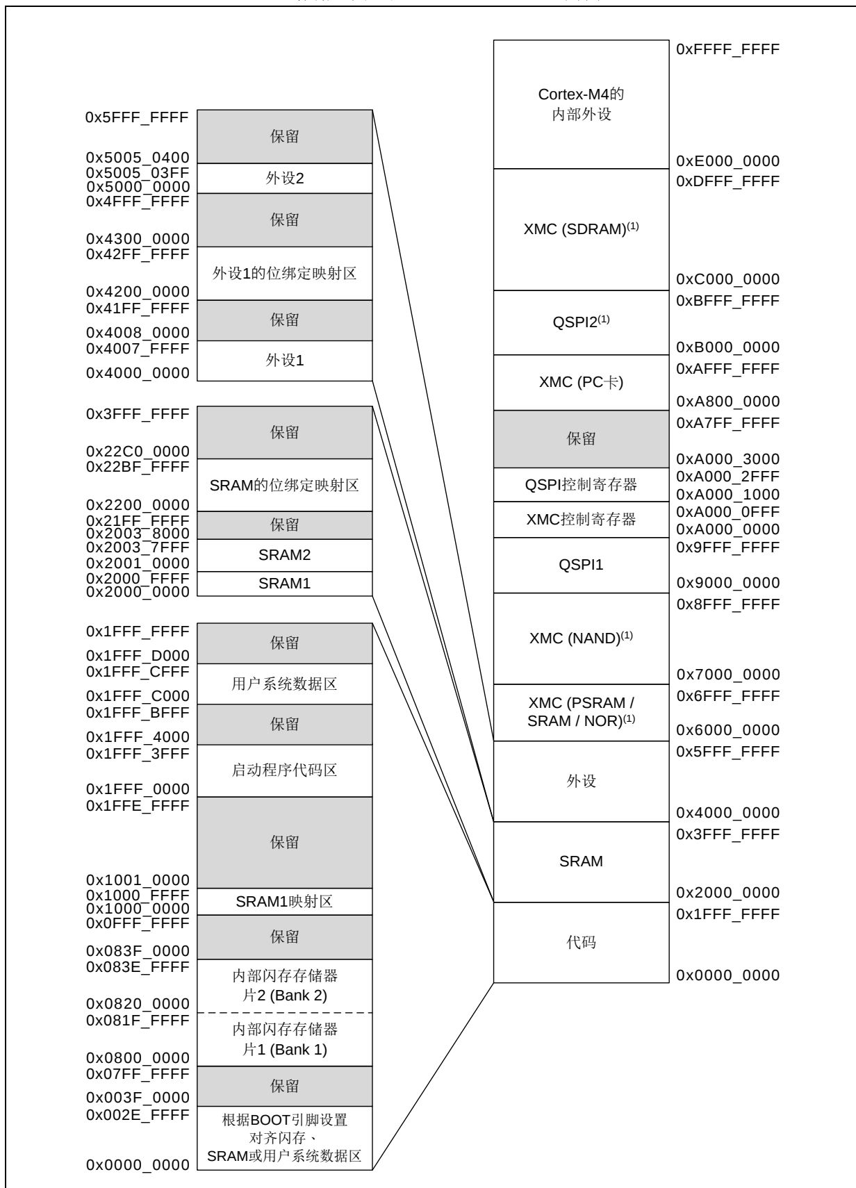
图 8. 存储器图（以 AT32F435/437xM 为例）
