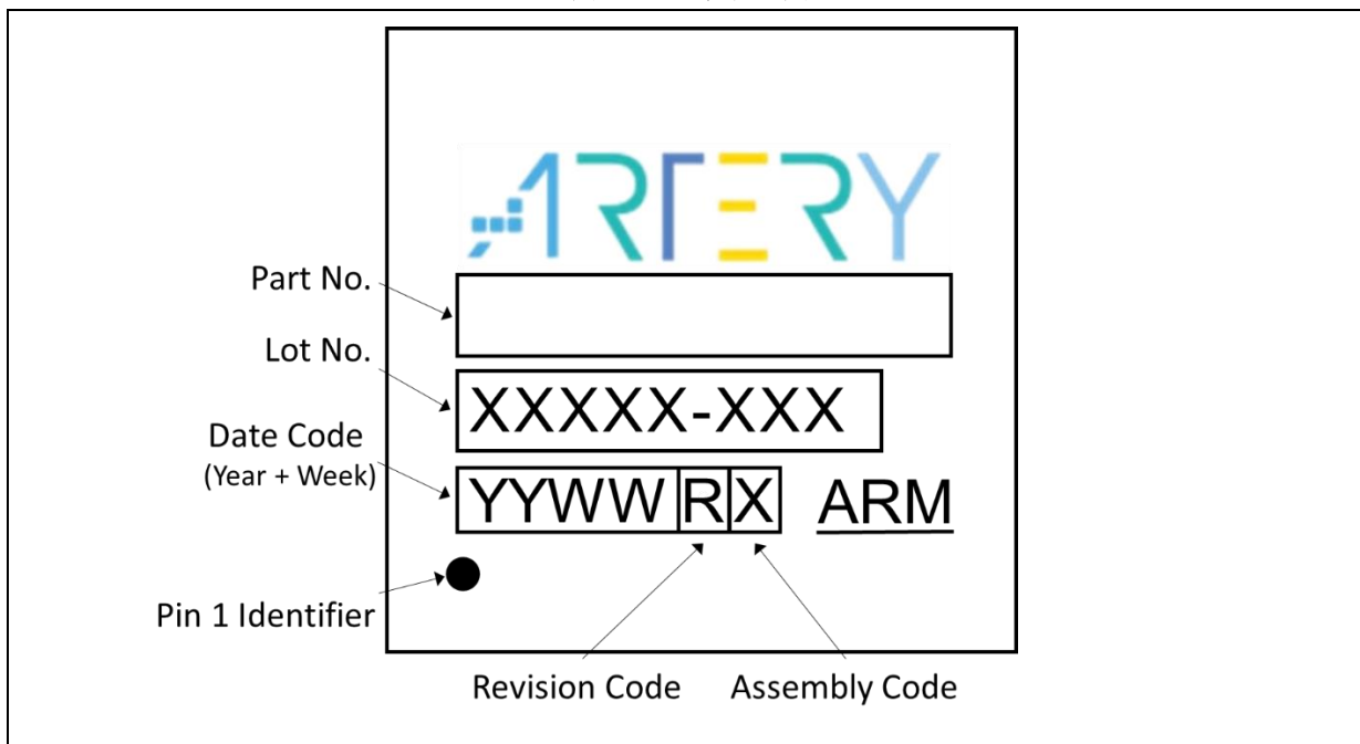
图 66. 丝印示意图
