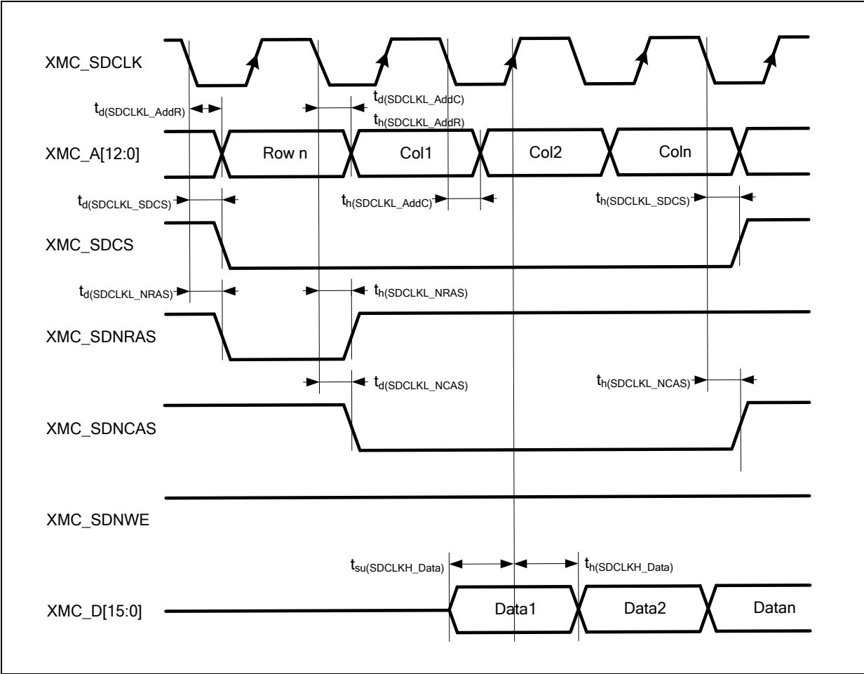
图 40. SDRAM 读操作波形
