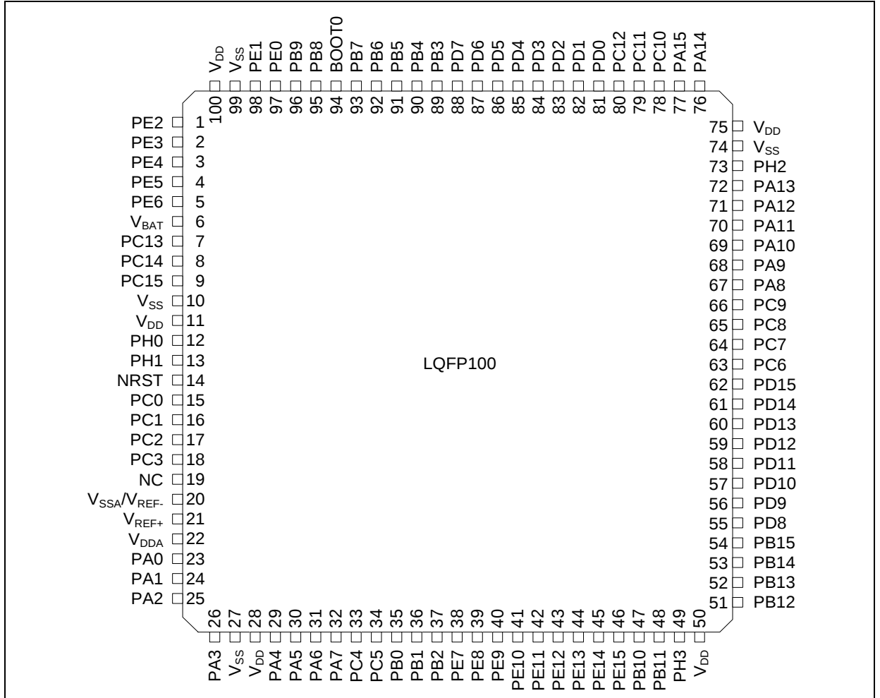
图 3. AT32F435/437 系列 LQFP100 引脚分布
