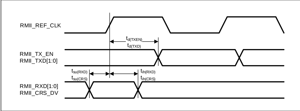
图 52. EMAC 的 RMII 接口时序图
