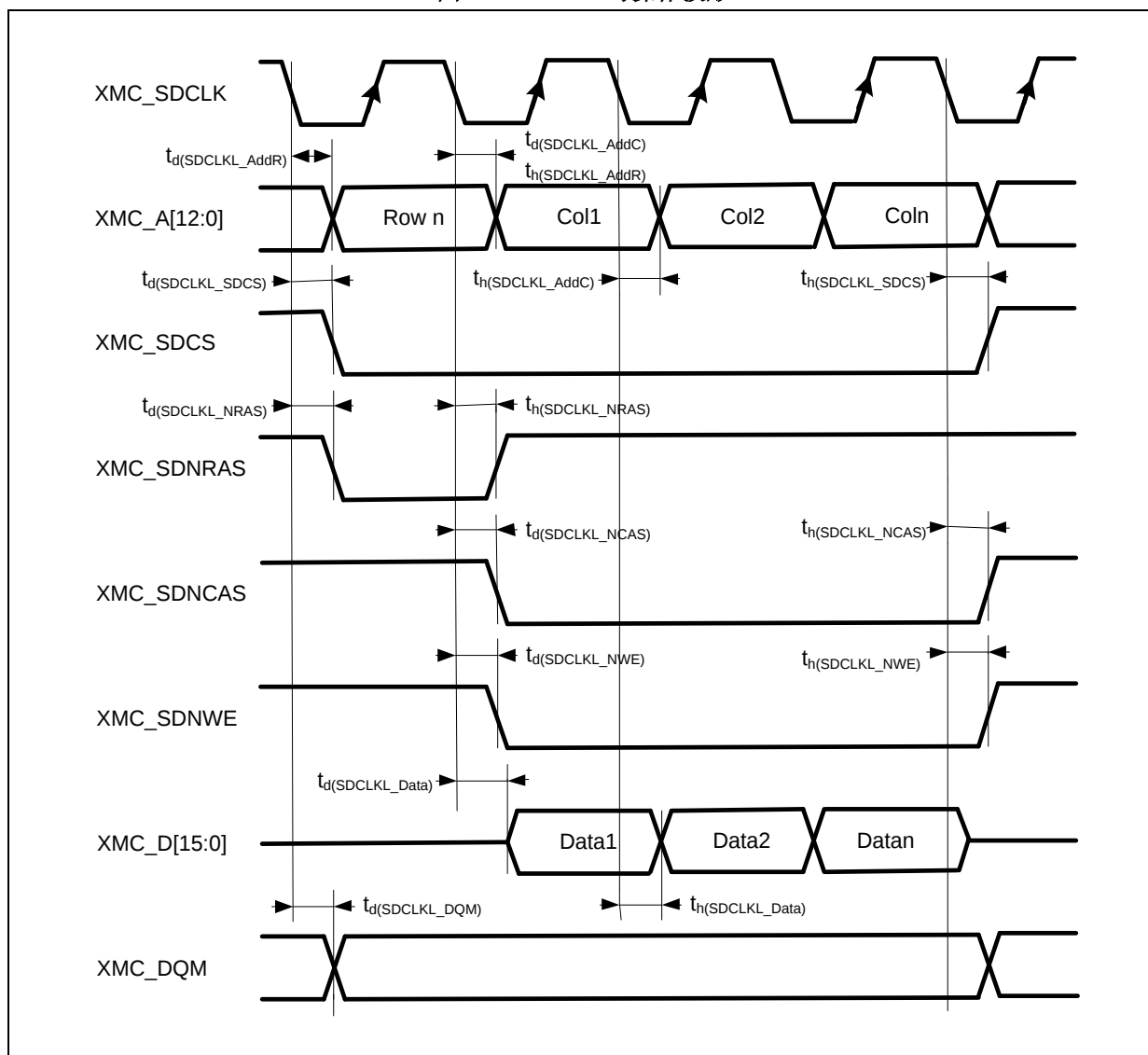
图 41. SDRAM 写操作波形
