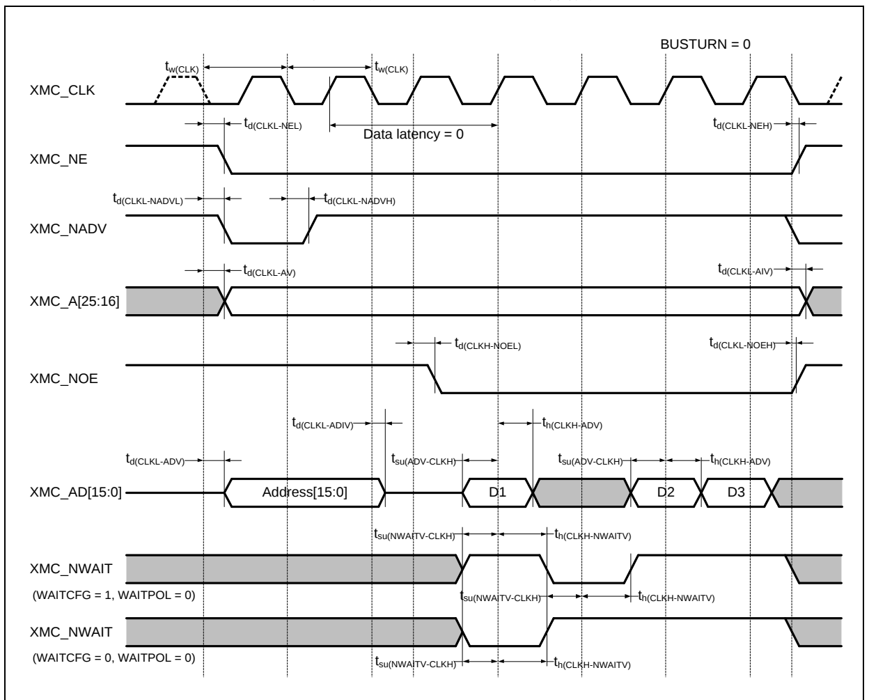
图 28. 同步总线复用 PSRAM/NOR 读操作波形
