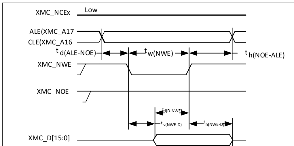
图 33. NAND 控制器在通用存储空间的写操作波形
