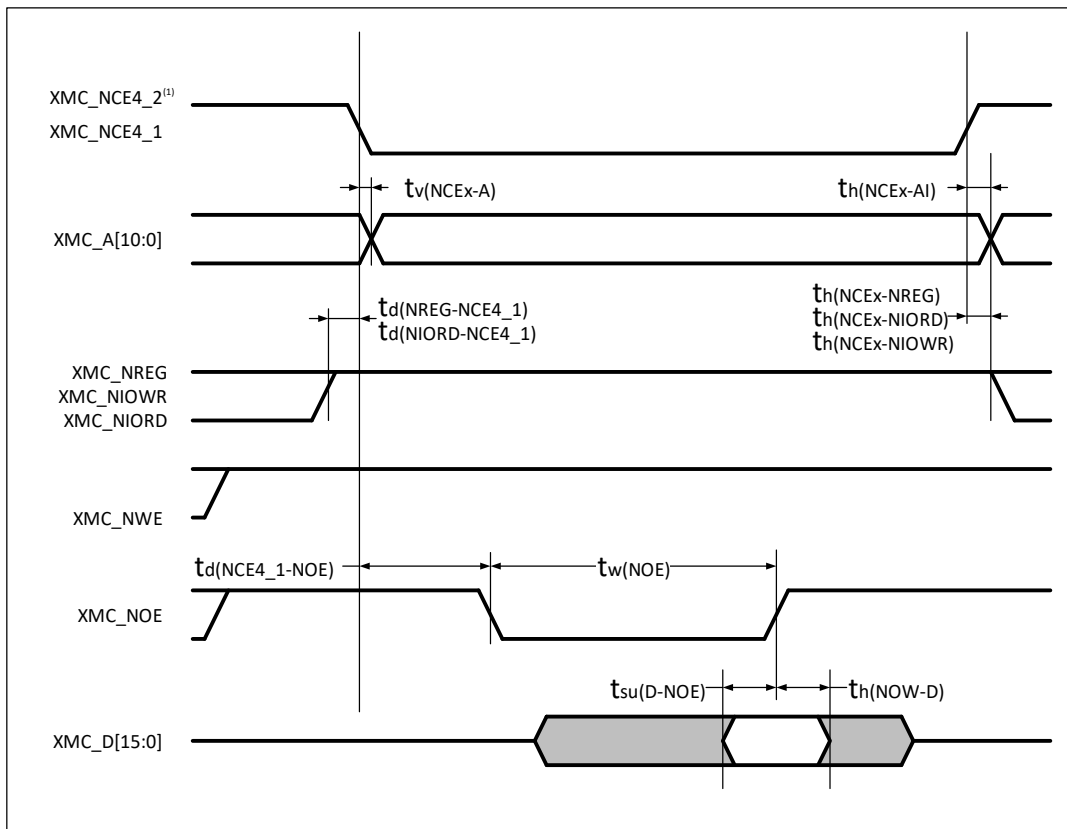
图 34. 通用存储空间读操作的 PC 卡/CF 卡控制器波形
