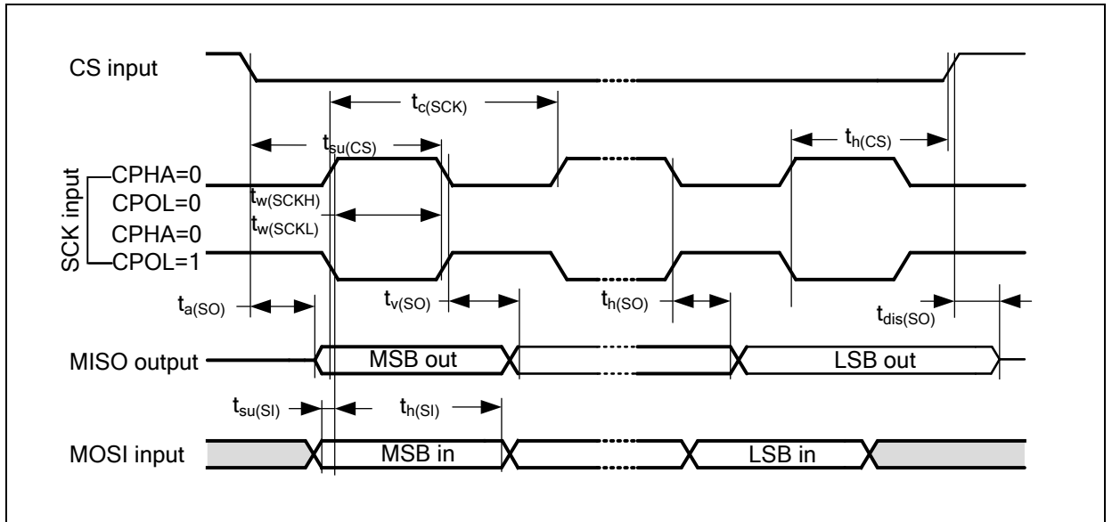
图 43. SPI 时序图 - 从模式和 CPHA = 1
