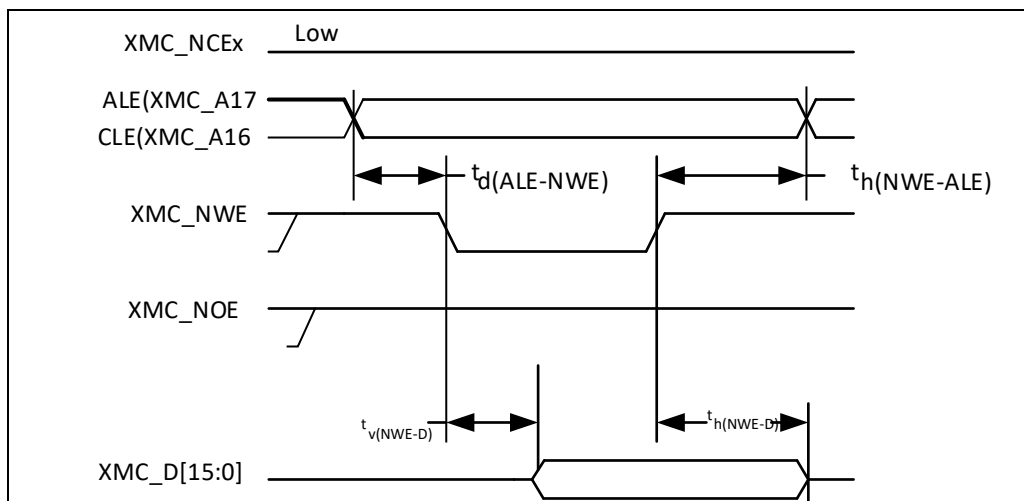
图 31. NAND 控制器写操作波形
