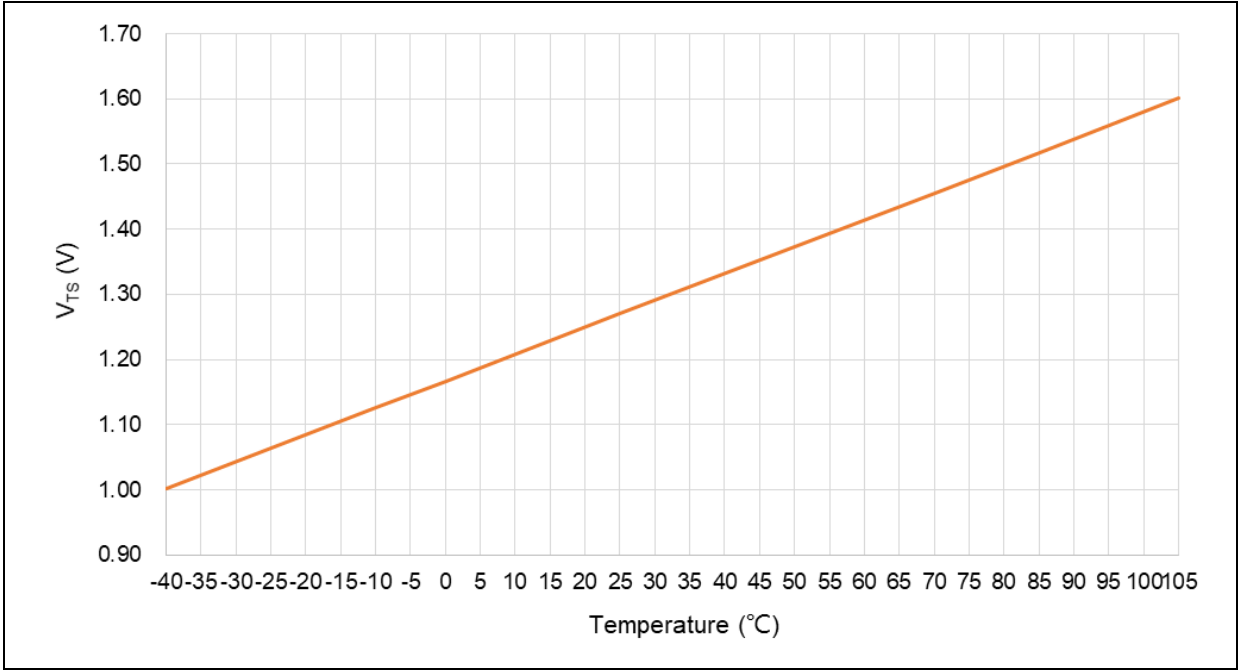
图 59. V_{TS} 对温度理想曲线图
