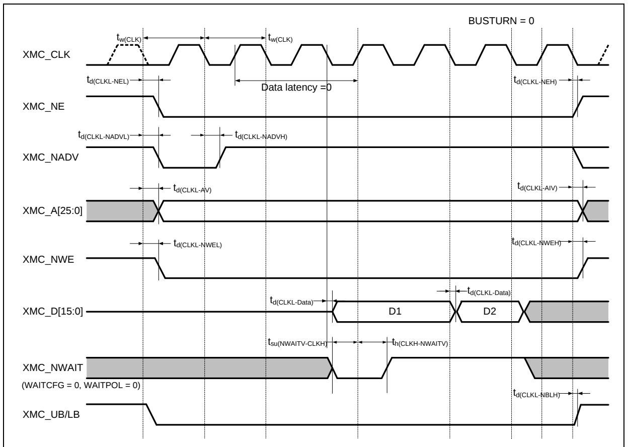
图 27. 同步非总线复用 PSRAM 写操作波形
