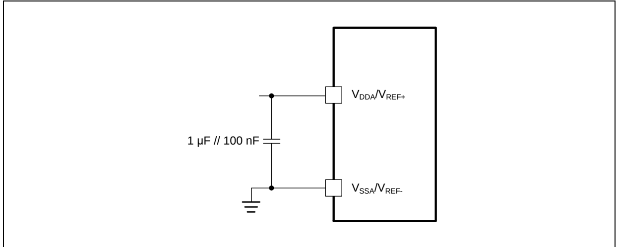
图 58. 供电电源去耦线路（无外部 V_{REF+} 引脚封装）
