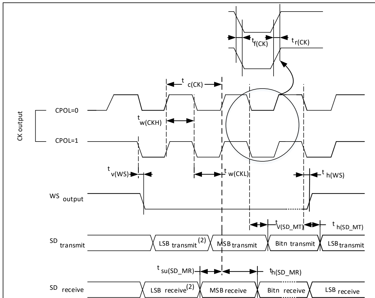
图 46. I 2 S 主模式时序图 (Philips 协议)
