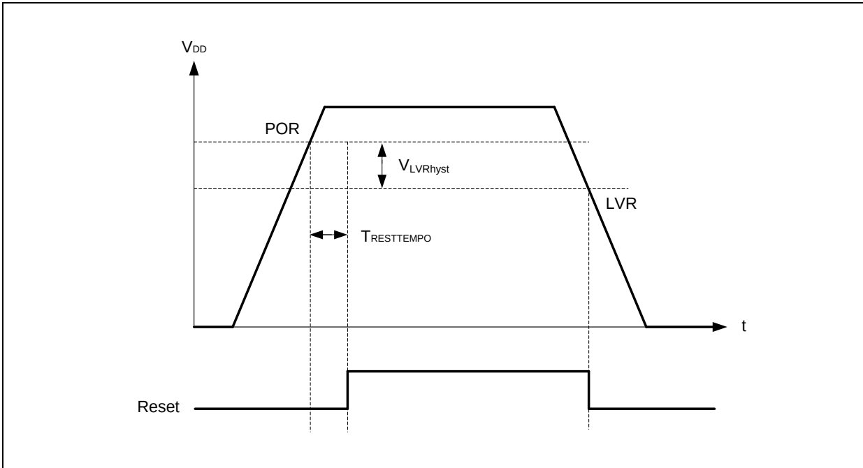
图 10. 上电复位和低电压复位的波形图
