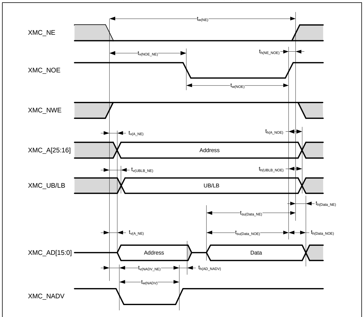
图 24. 异步总线复用 PSRAM/NOR 读操作波形
