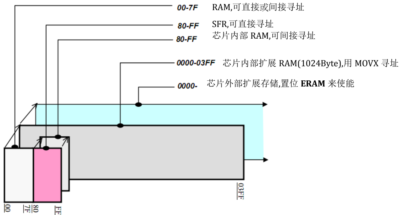
MPC89x54/58/515 RAM 空间
