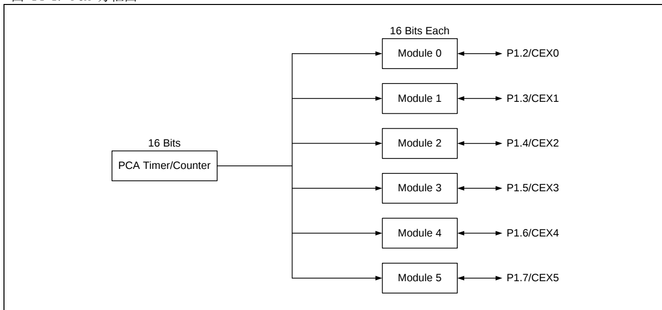
图 14-1. PCA 方框图
