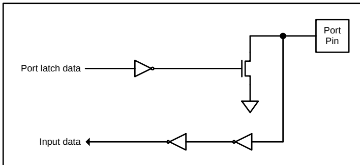
图 9-4 开漏输出
