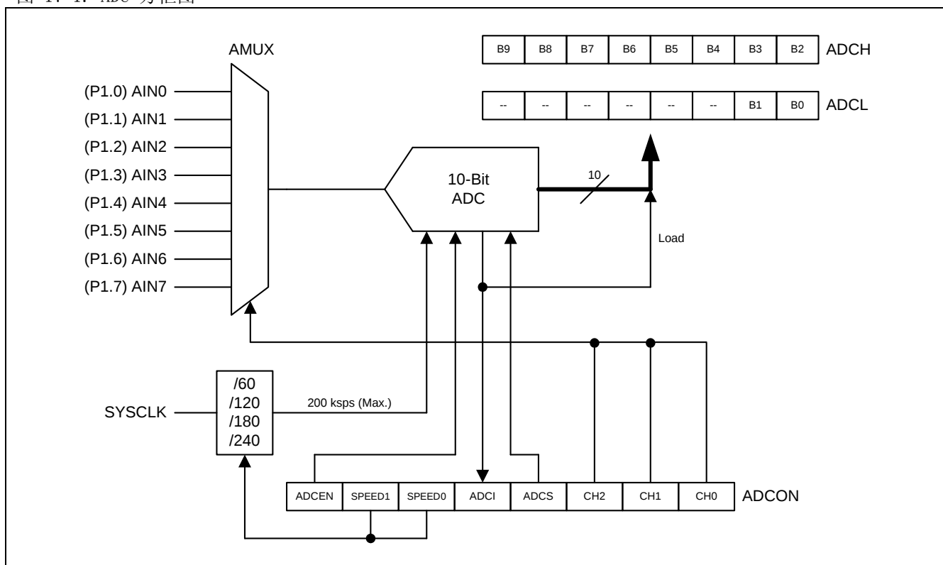
图 17-1. ADC 方框图
