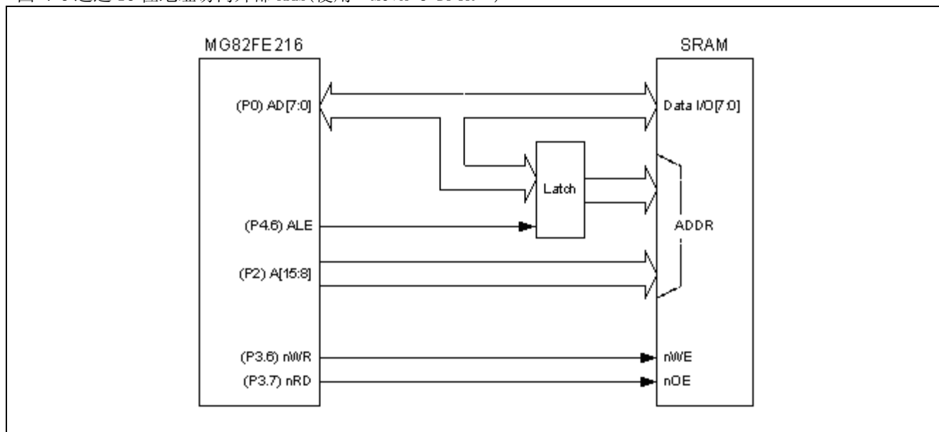
图 7-6 通过 16 位地址访问外部 RAM(使用 ‘MOVX @ DPTR’ )
