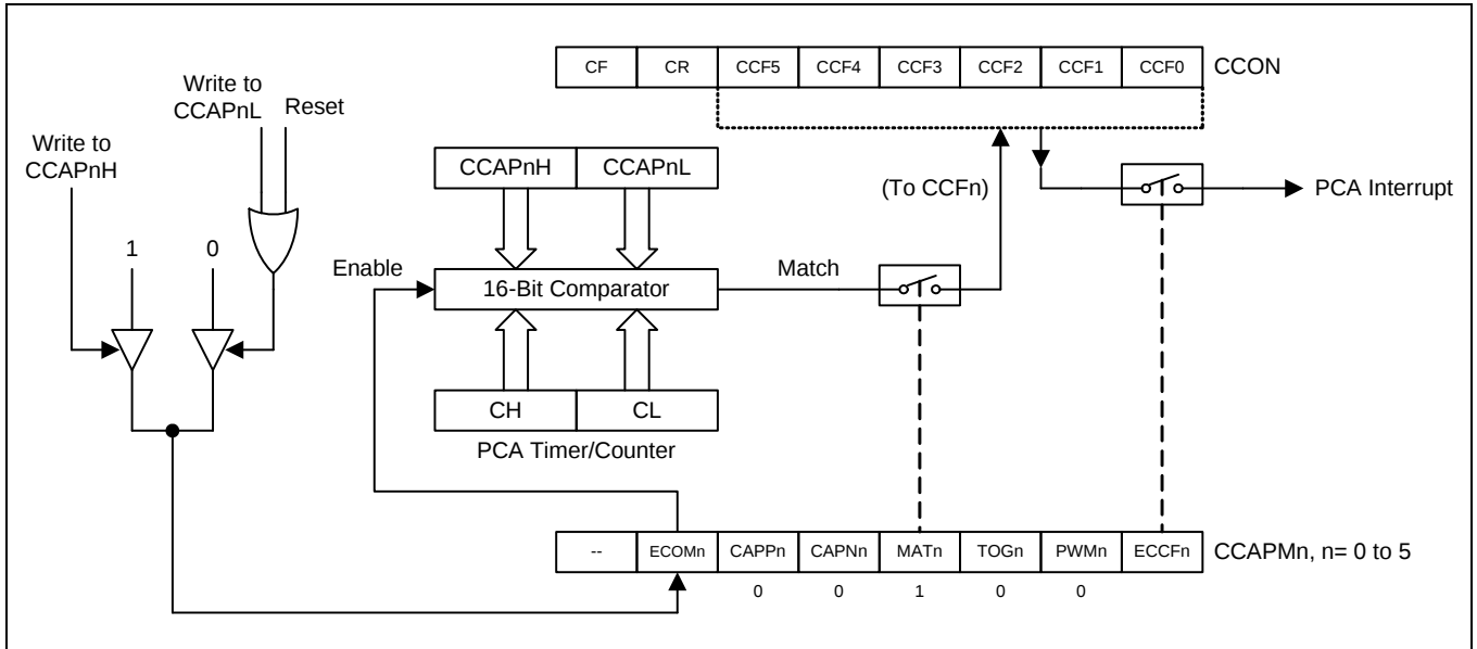
图 14-5. PCA 软件定时器模式
