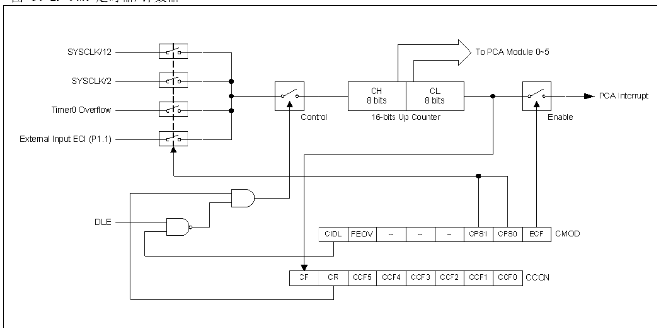
图 14-2. PCA 定时器/计数器
