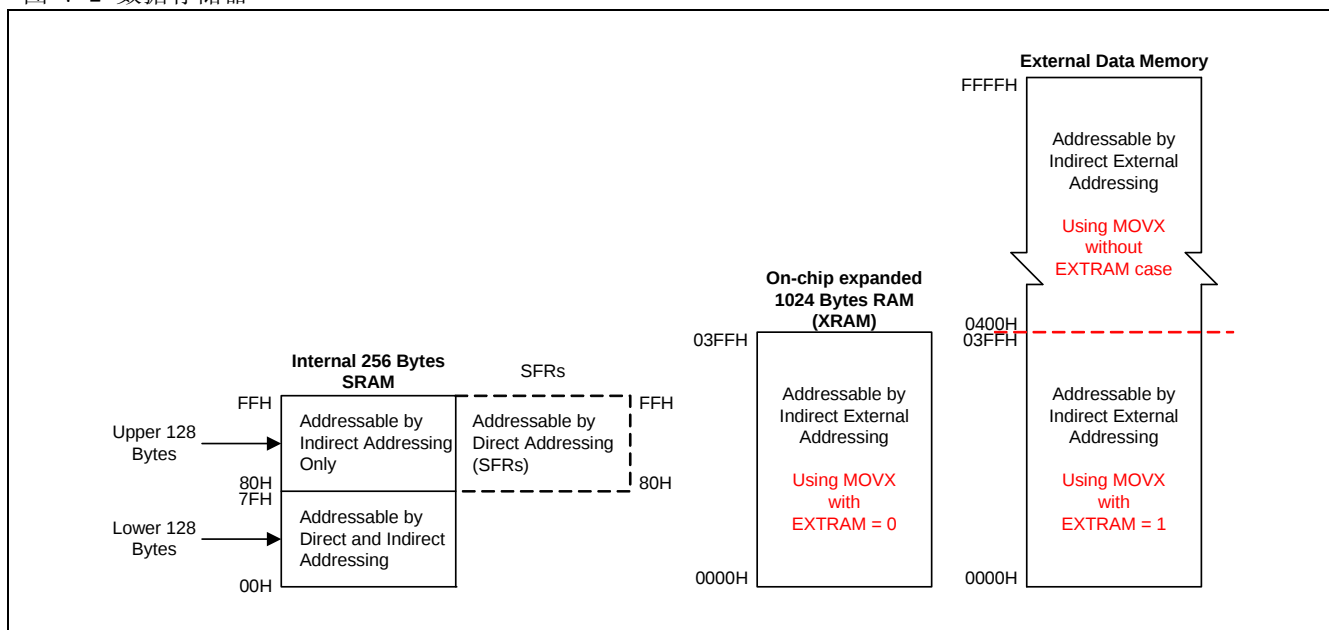
图 7-2 数据存储器
