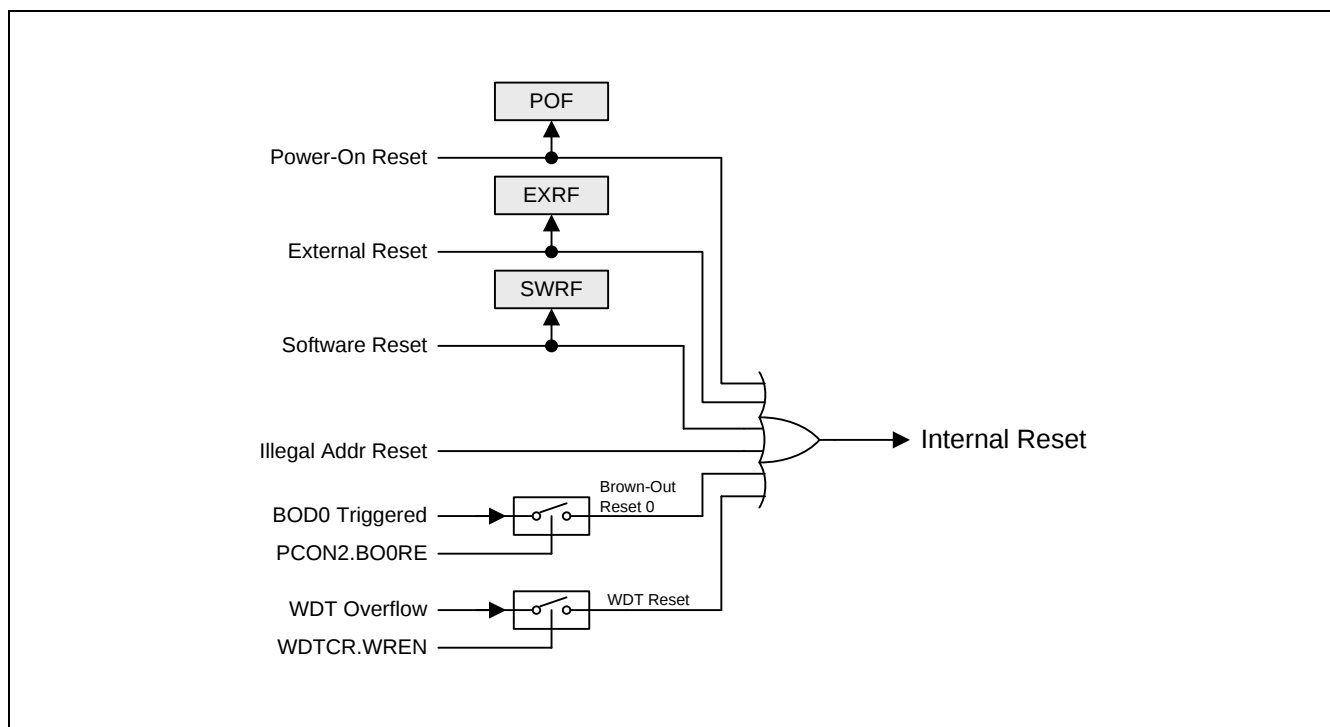
图 11-1. 系统复位源
