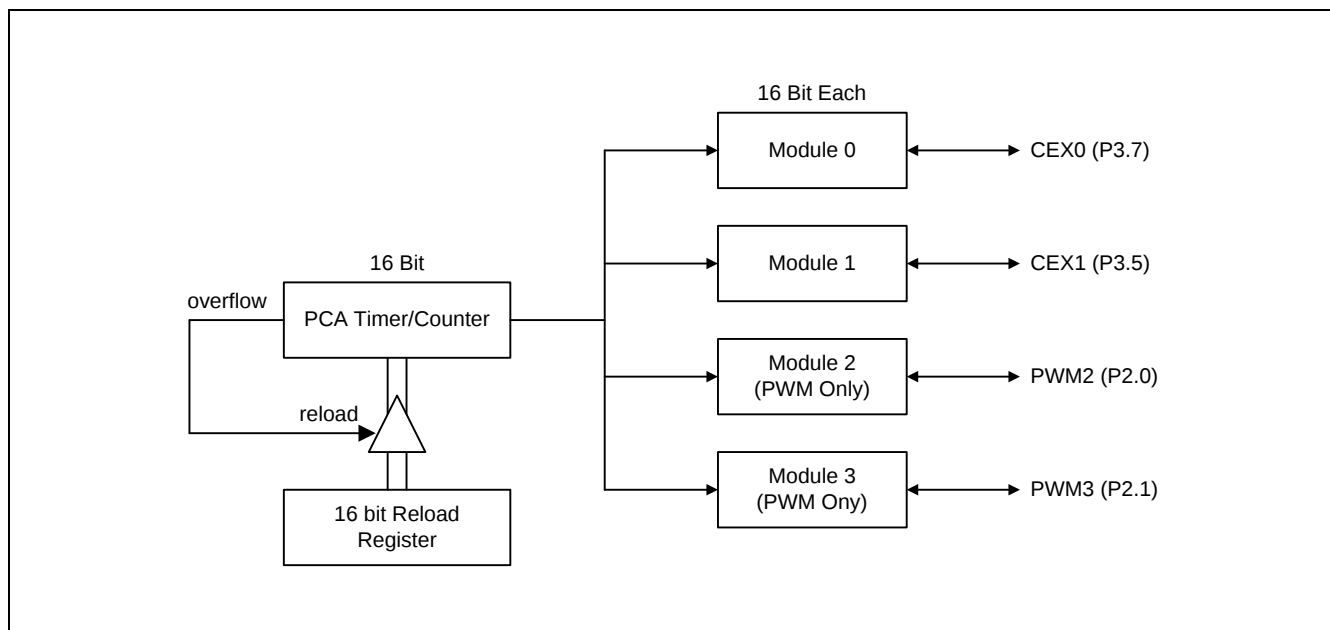
图 17-1. PCA 方框图
