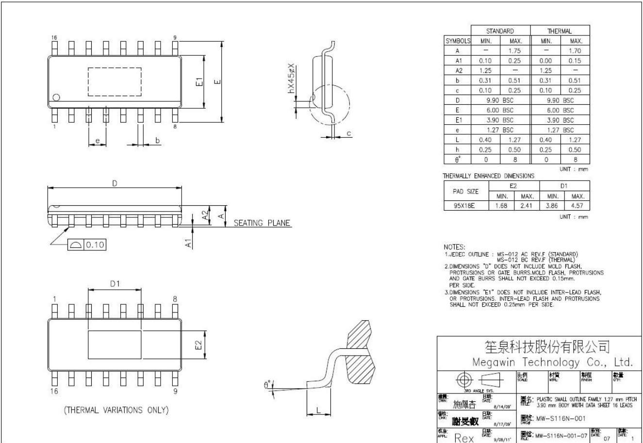
图 29-3. SOP-16
