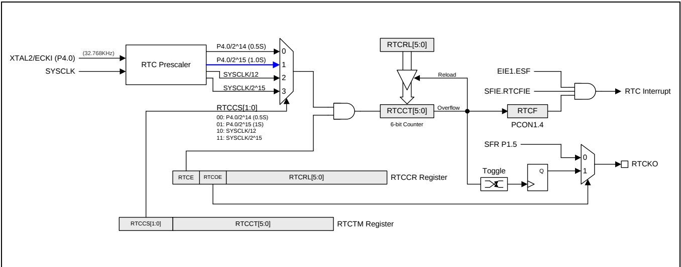
图 10–1. 实时时钟计数器
