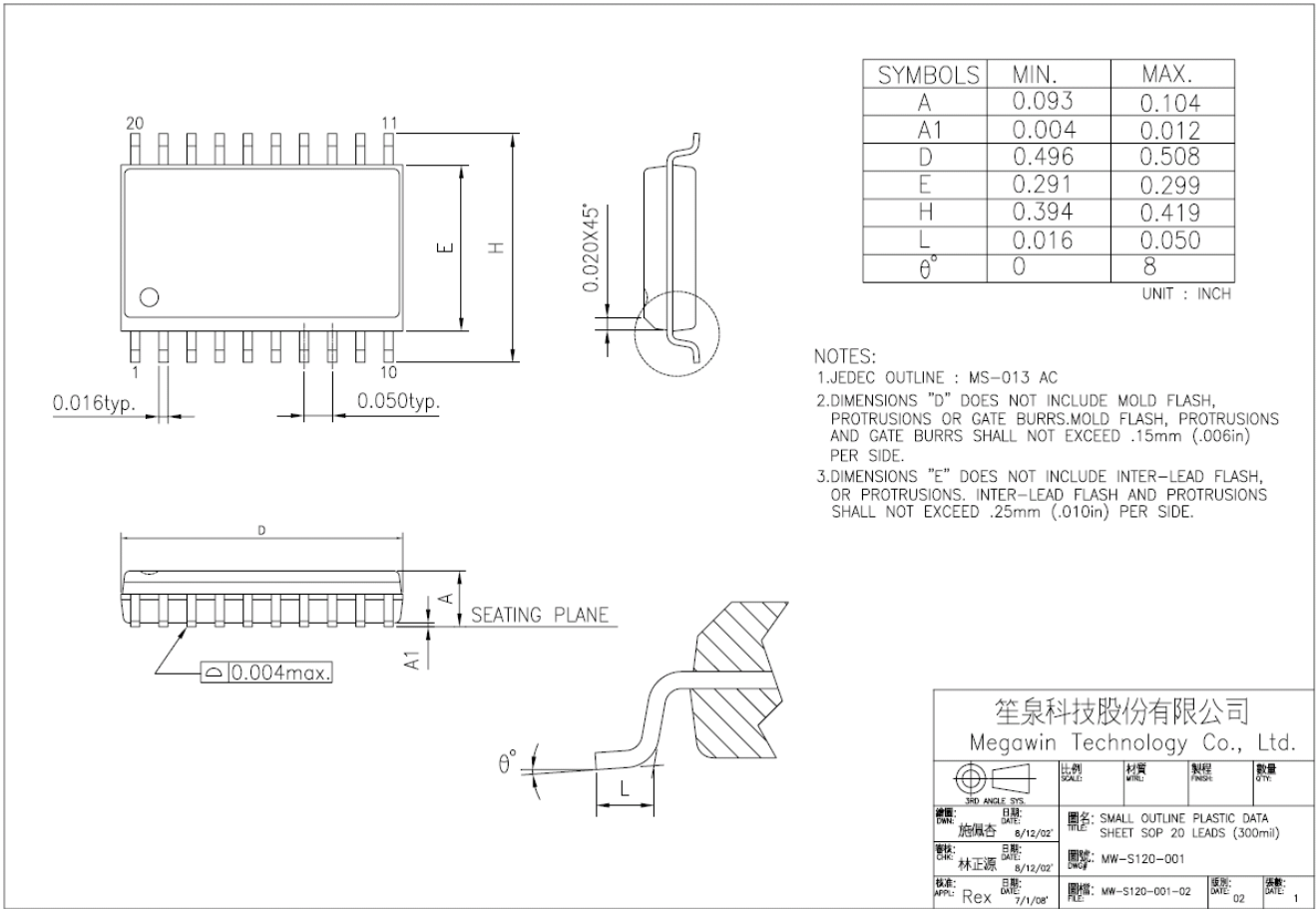
图 29-2. SOP-20
