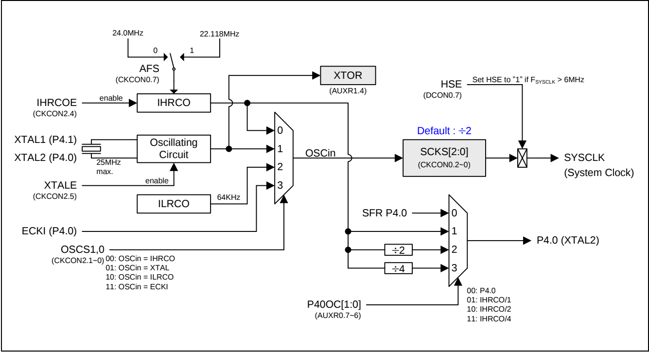
图 8-1. 系统时钟
