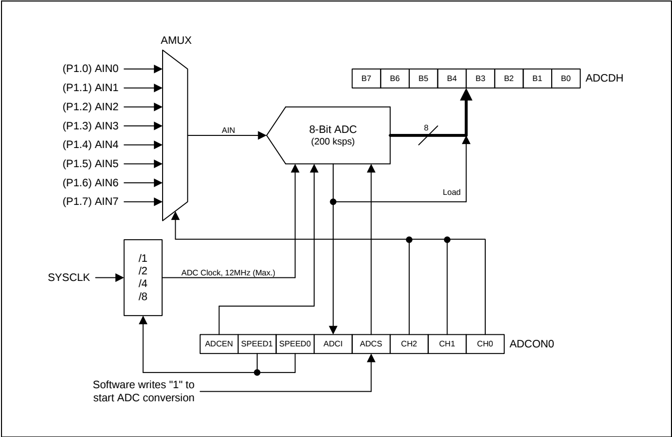
图 21-1. ADC 方框图
