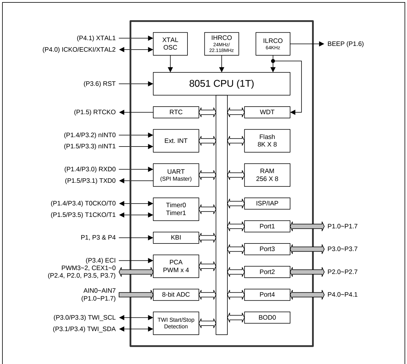
图 2-1. 方框图
