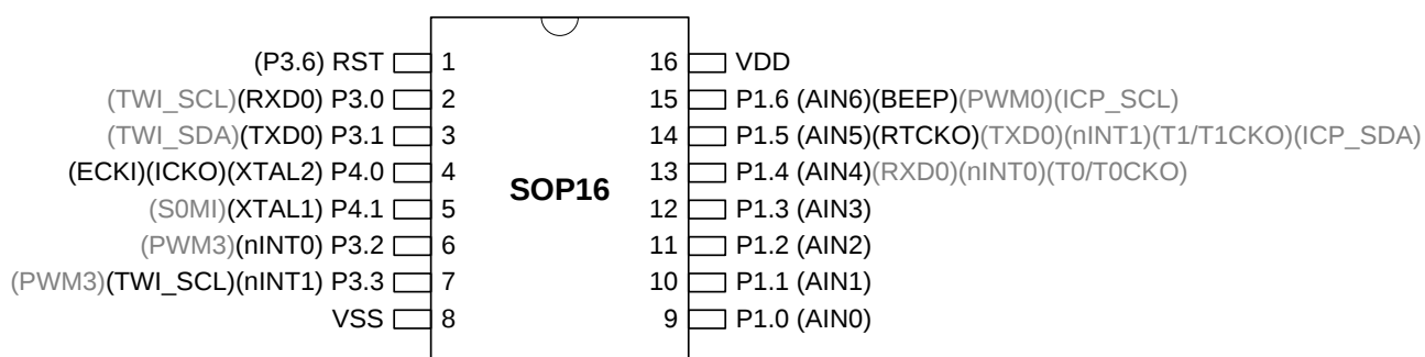
图 4-3. MA86E/L508AS16 顶视图
