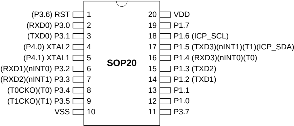
图 4-1. MA86E/L104AS20 顶视图
