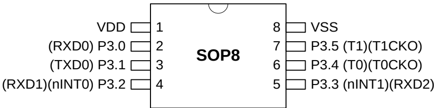
图 4-3. MA86E/L104AS8 顶视图
