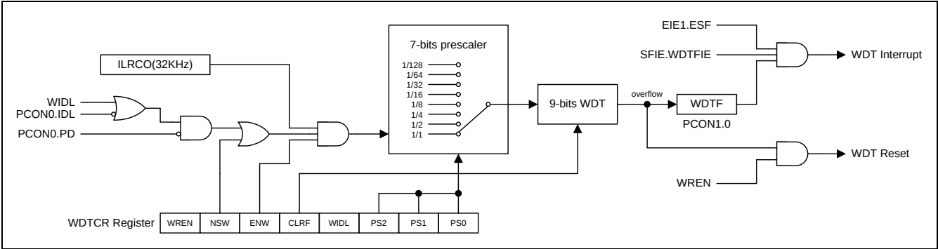
图 10-1 结构框图
