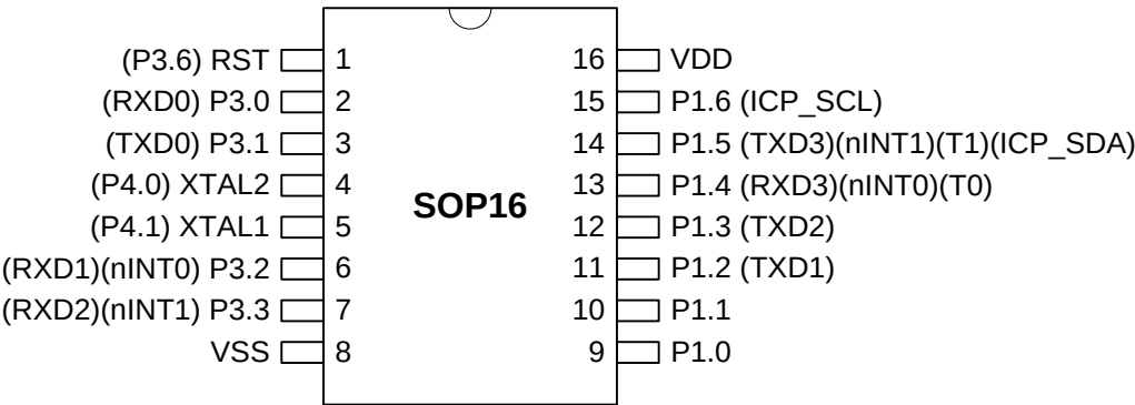
图 4-2. MA86E/L104AS16 顶视图
