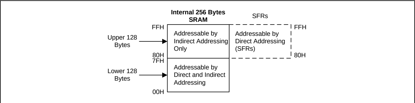
图 7-2 数据存储器
