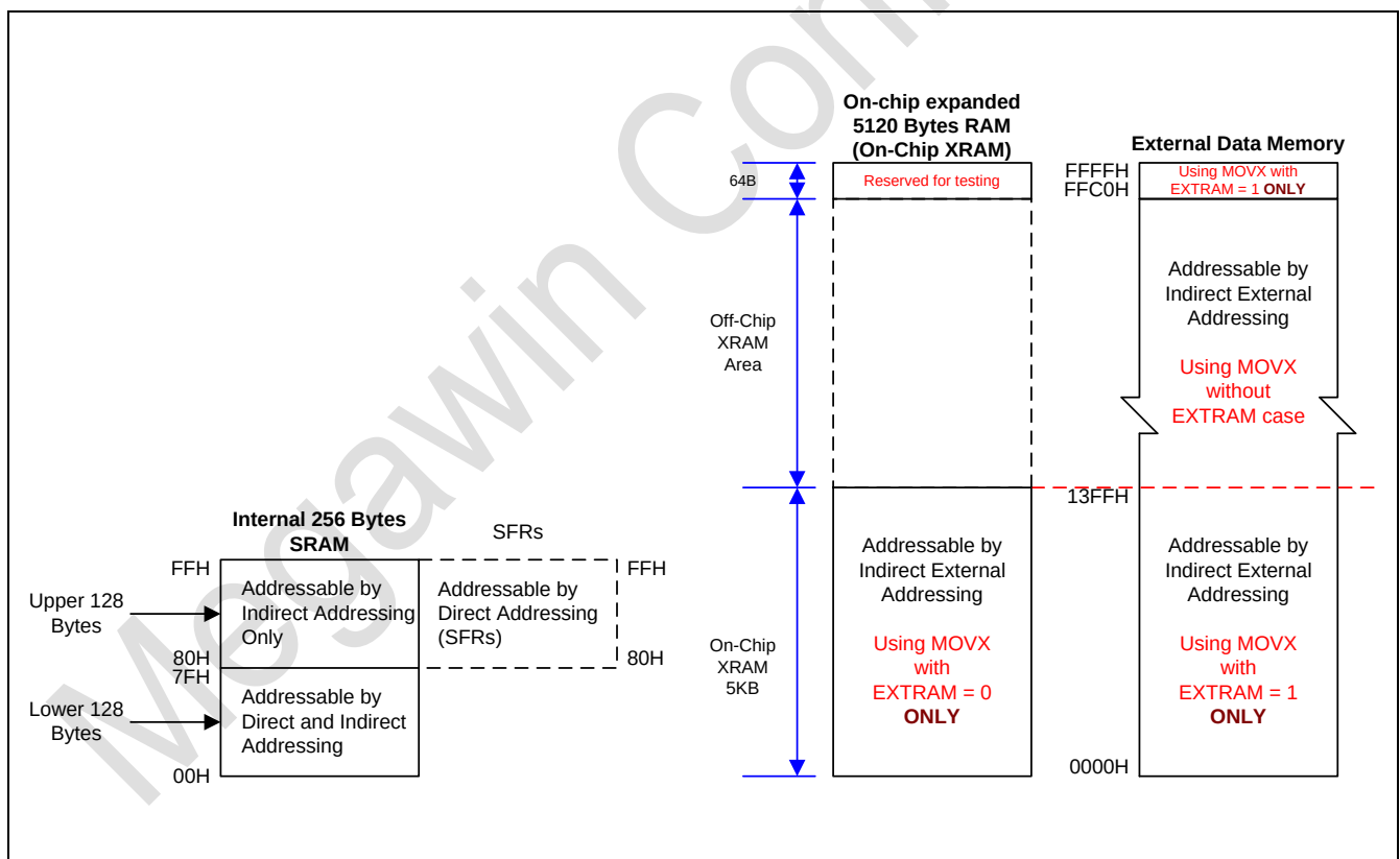
图 7-2 数据存储器
