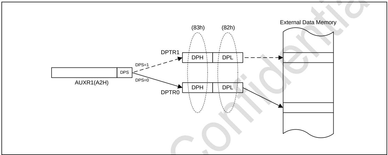
图 8-1 双 DPTR
