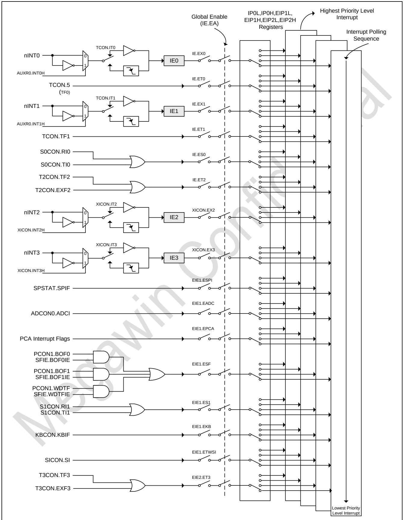
图 14-1. 中断系统
