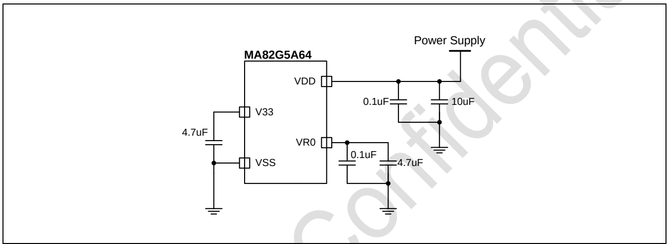
图 27-1. 电源电路
