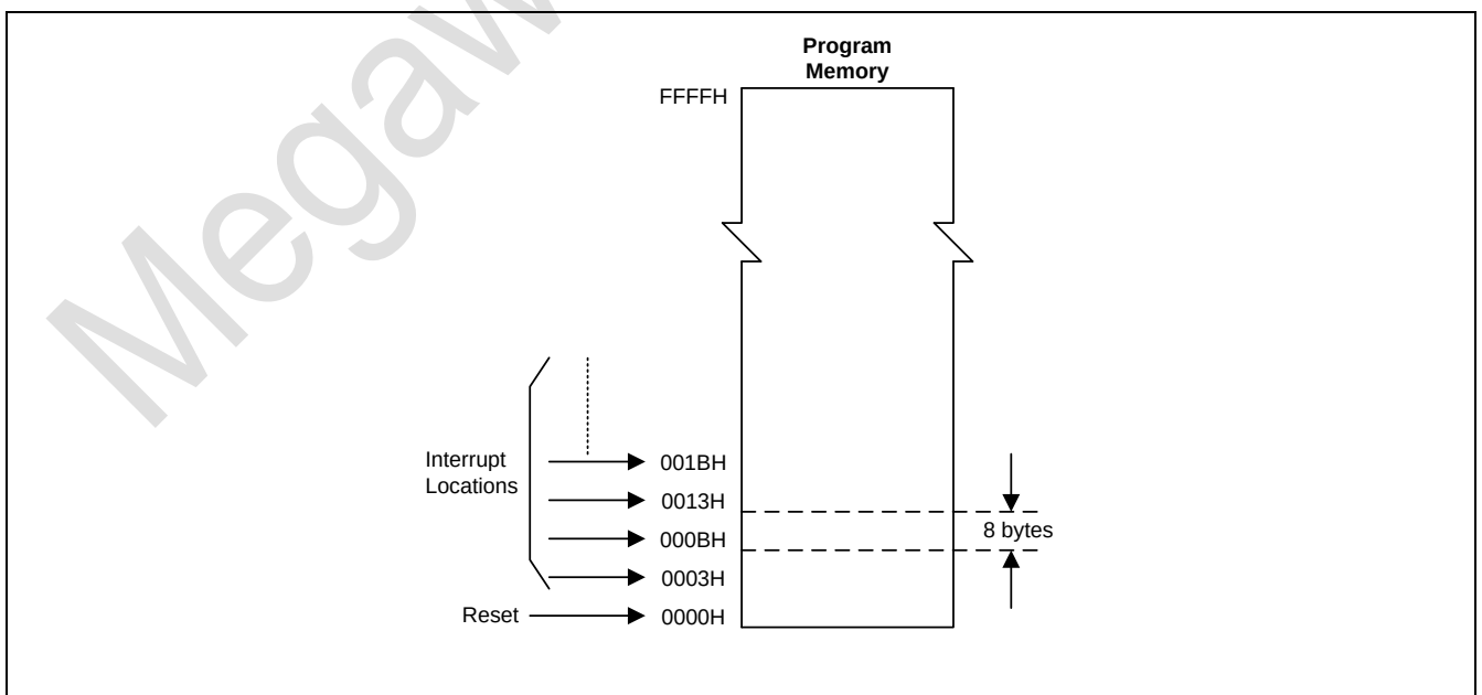
图 7-1 程序存储器
