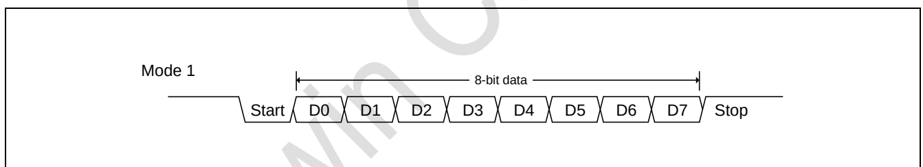
图 16-1. 模式 1 数据帧
