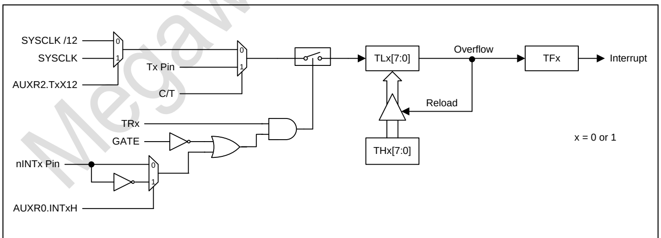
图 15-3. 定时器 0/1 模式 2 结构图
