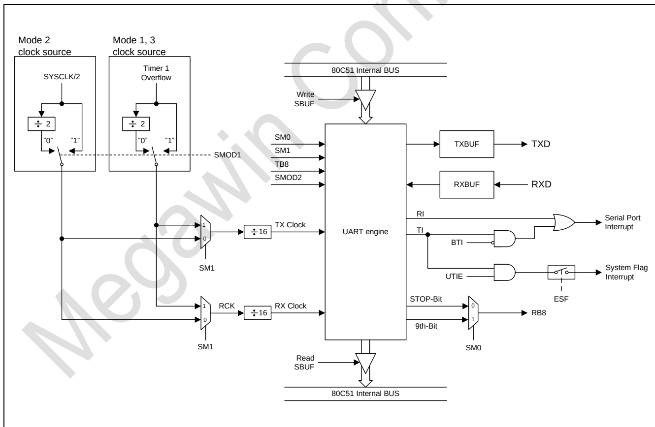
图 16-6. 串行口模式 1, 2, 3
