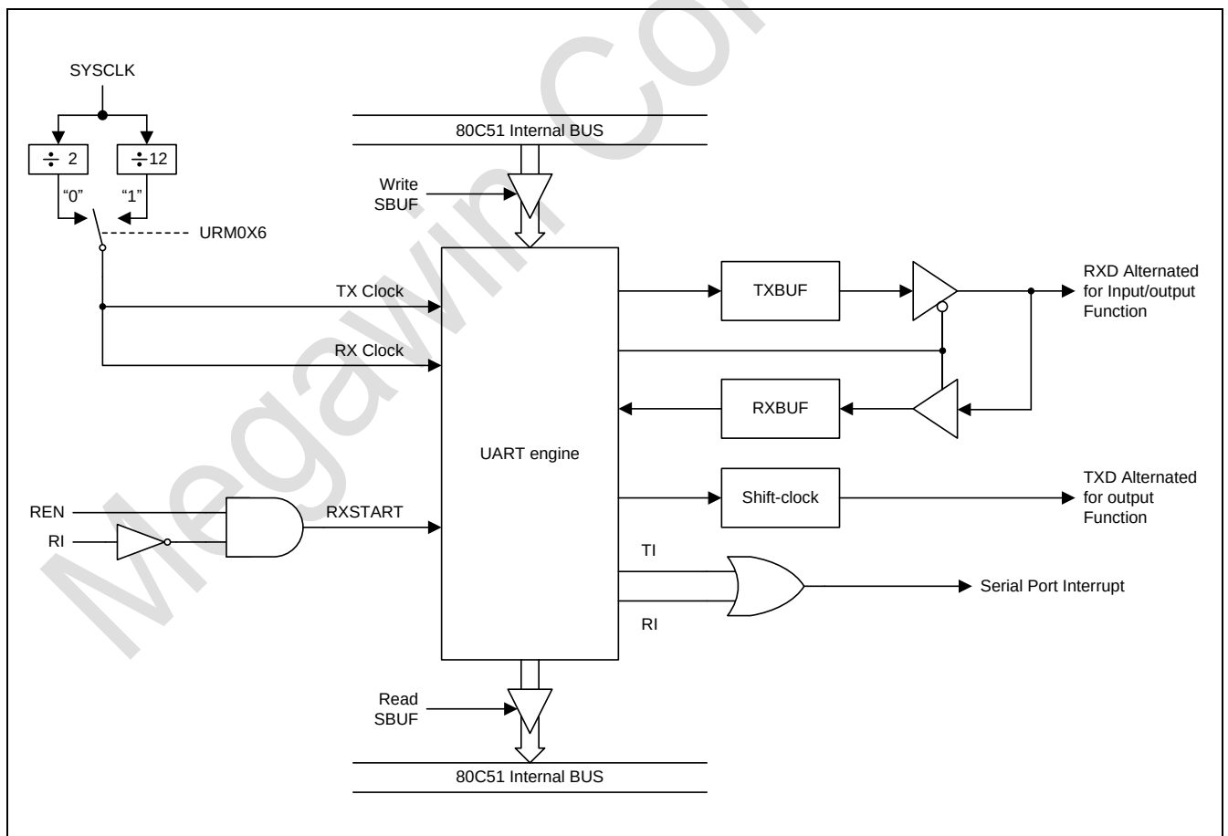
图 16-3. 串行口 0 模式 0
