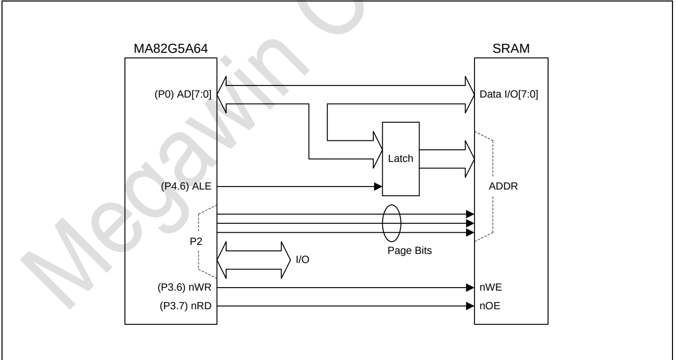
图 7-5 通过 8 位地址访问外部 RAM(使用'MOVX @ Ri' 和页位选择)
