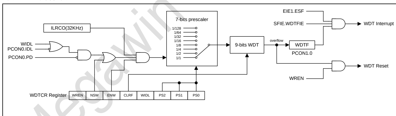
图 10-1 结构框图
