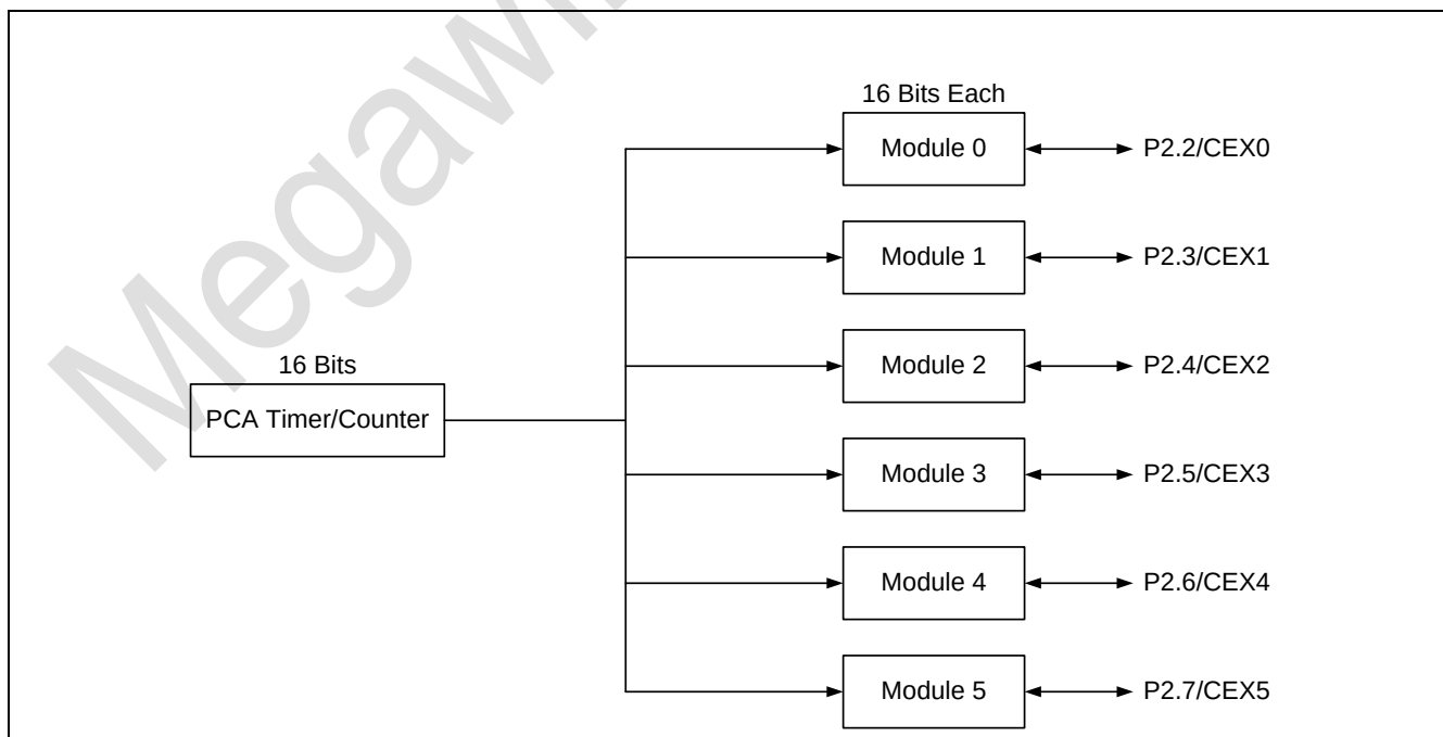
图 18-1. PCA 方框图
