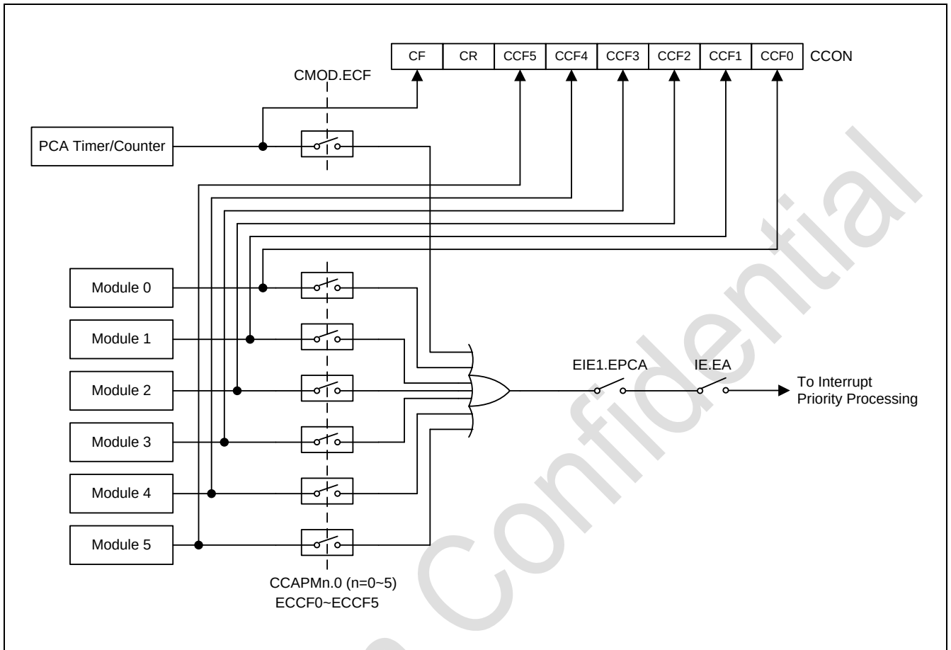
图 18-3. PCA 中断系统
