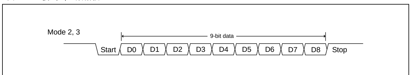
图 16-2. 模式 2, 3 数据帧
