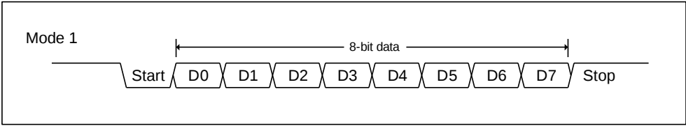
图 123-1 模式 1 数据帧
