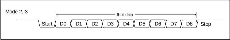
图 123-2 模式 2 数据帧
