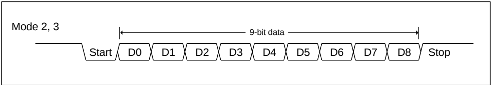
图 11-2 模式 2、3 数据帧
