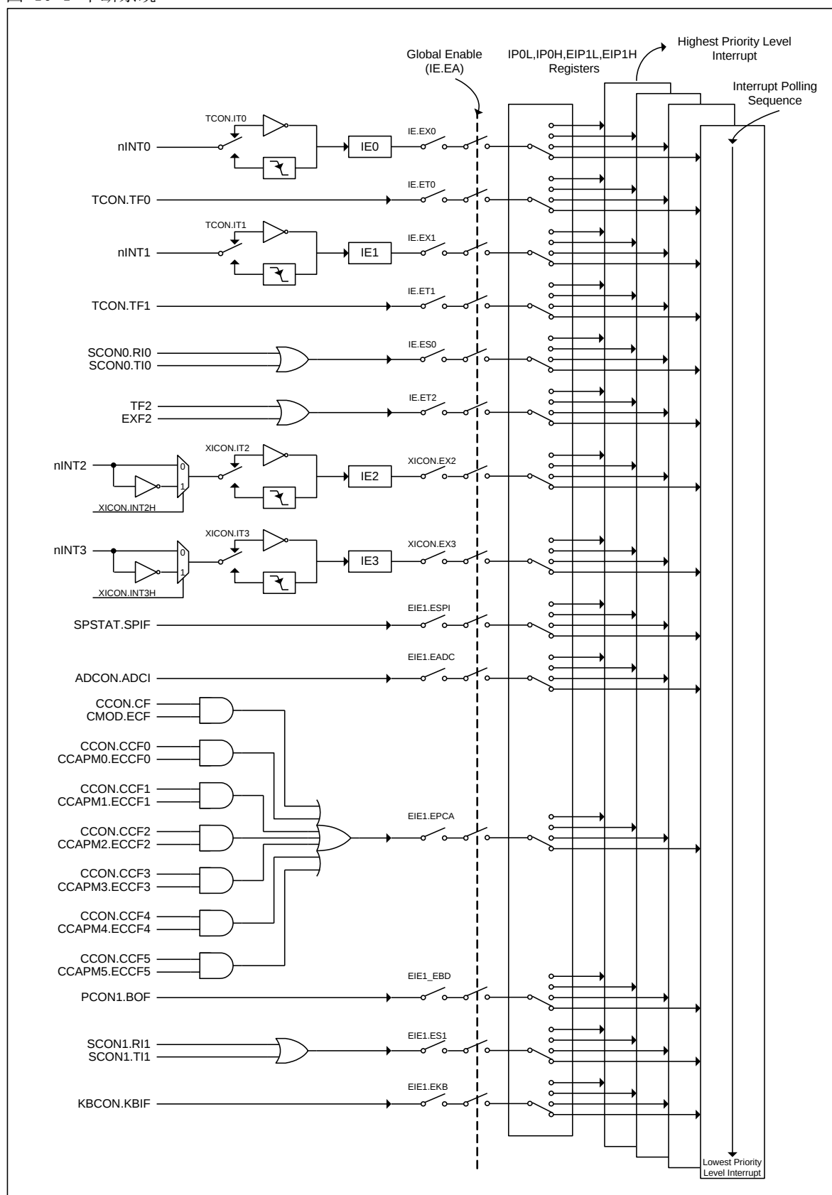
图 10-1 中断系统
