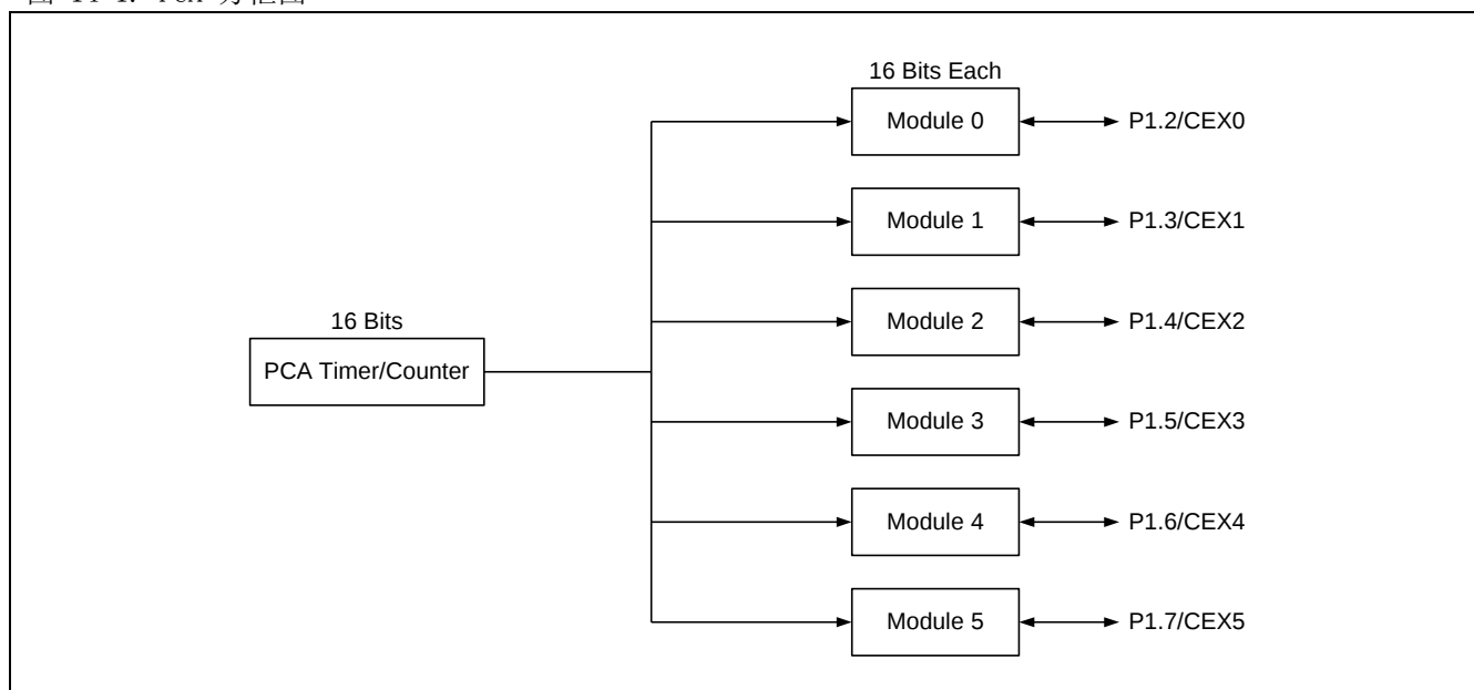
图 14-1. PCA 方框图
