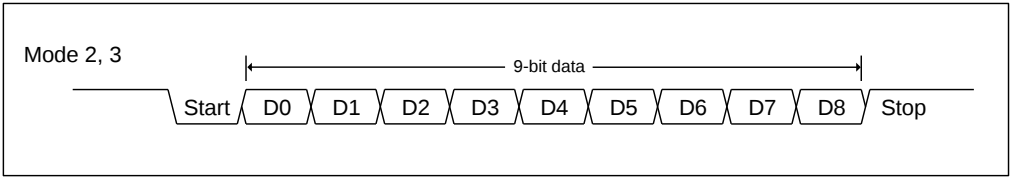
图 11-2 模式 2、3 数据帧
