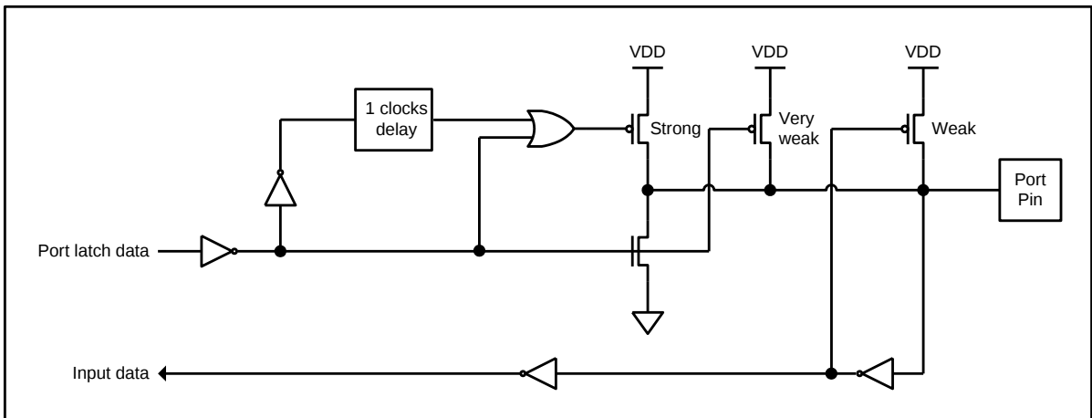
图 9-1 准双向 I/O
