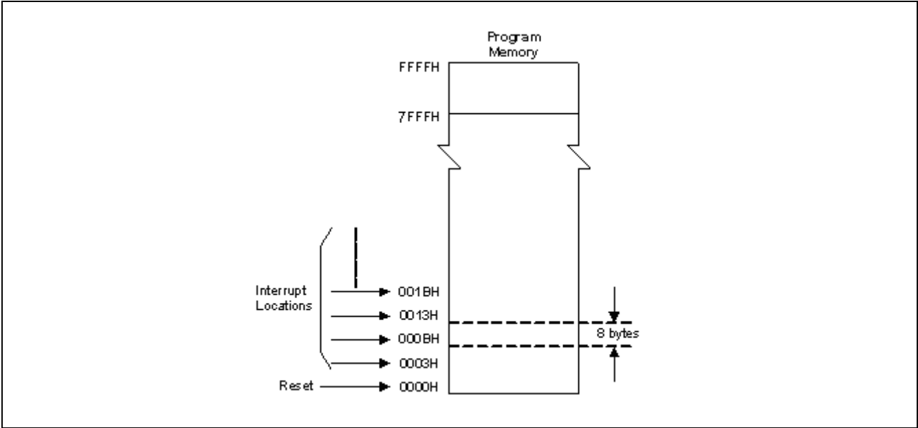
图 7-1 程序存储器
