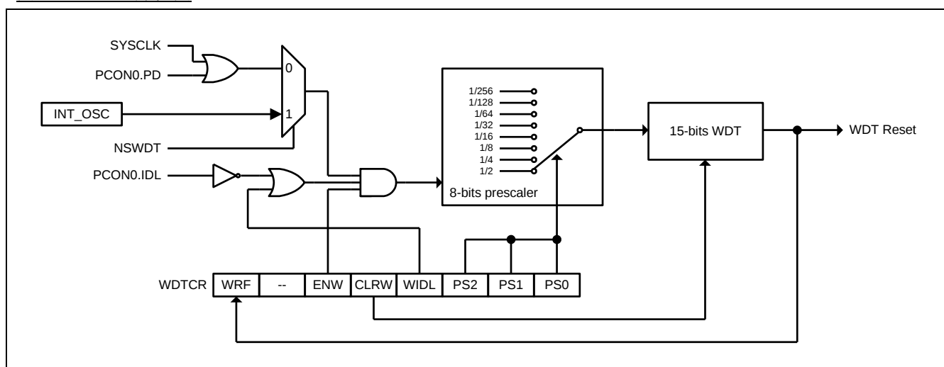
图 18-1. WDT 方框图
