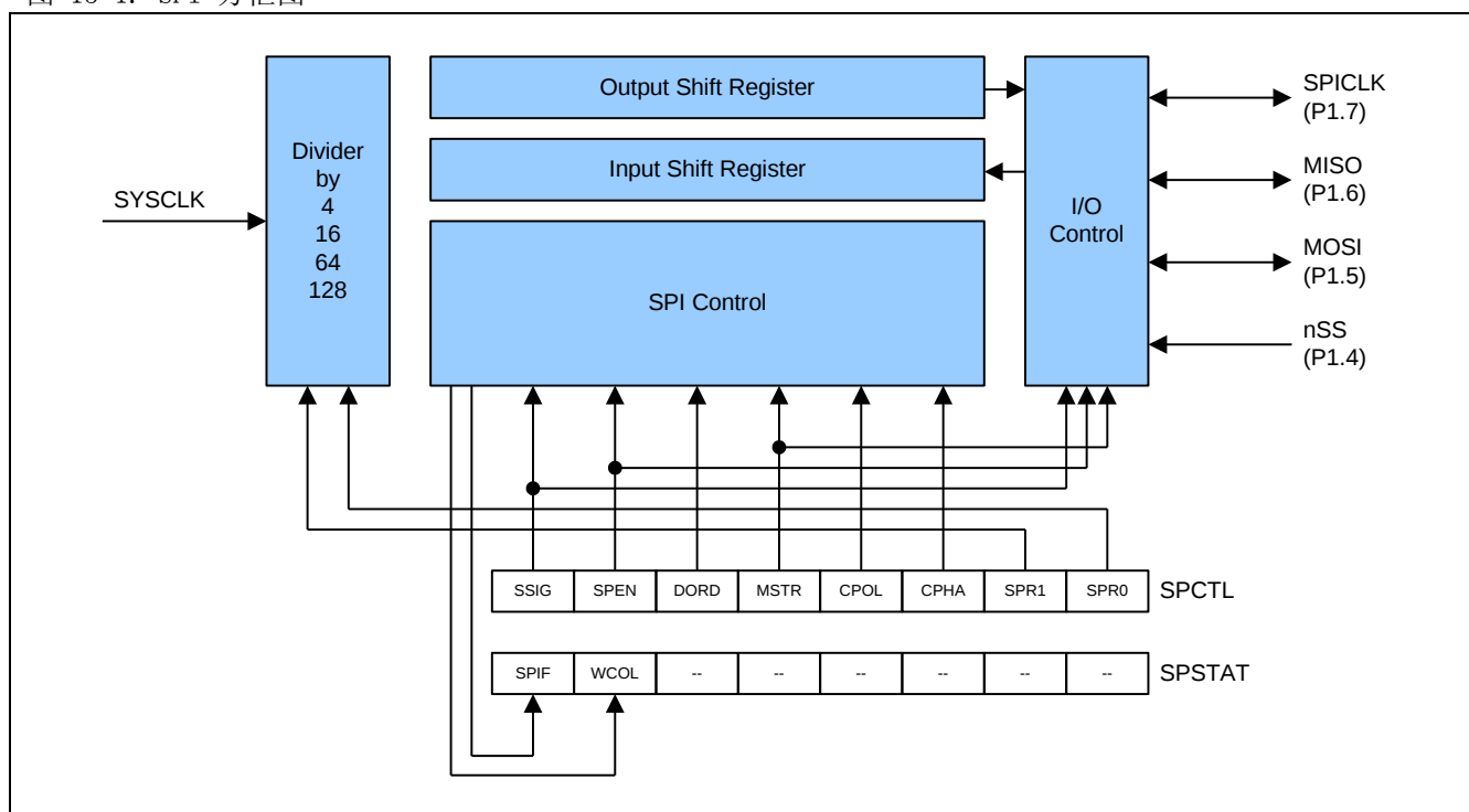
图 15-1. SPI 方框图
