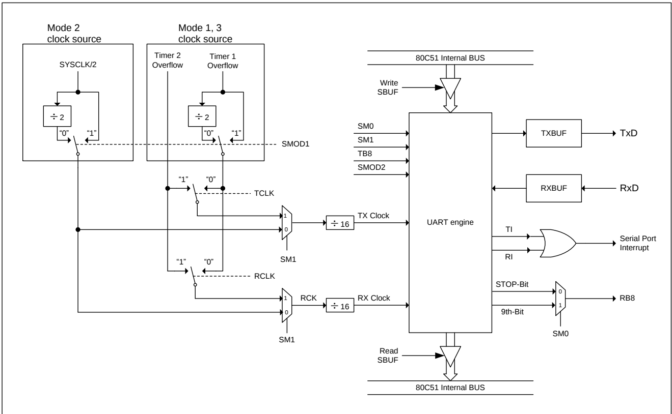
图 11-6 串行 0 模式 1、2、3
