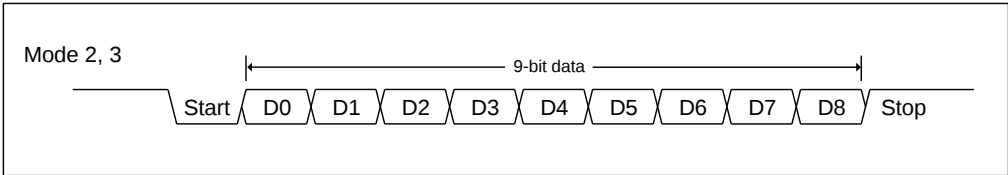
图 11-2 模式 2、3 数据帧
