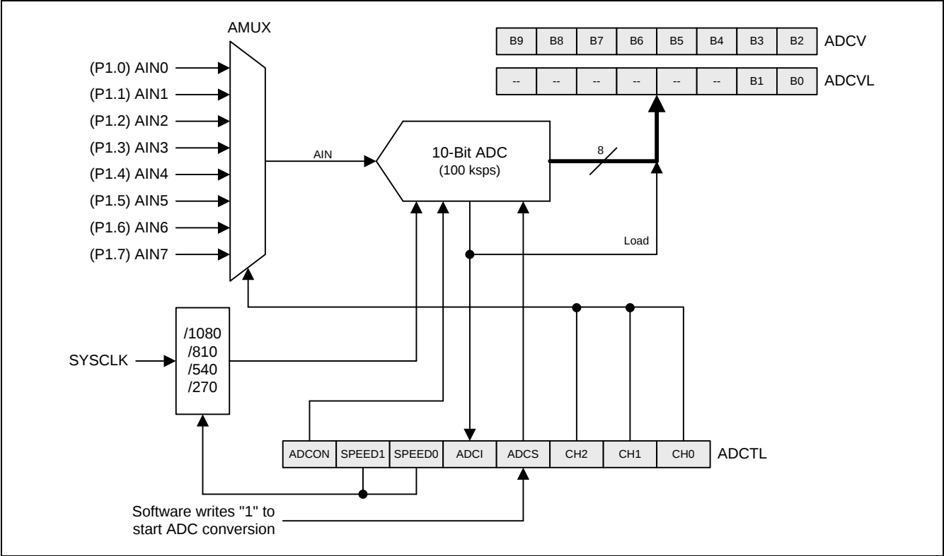
图 18-1. ADC 方框图
