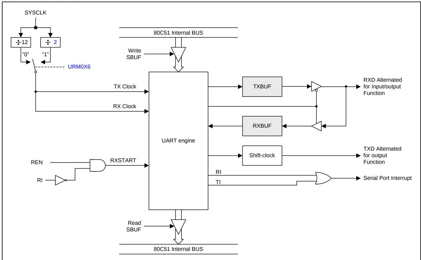
图 15-3. 串口模式 0
