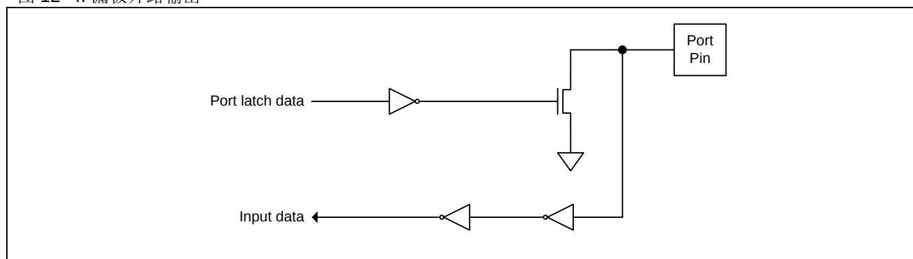
图 12-4. 漏极开路输出
