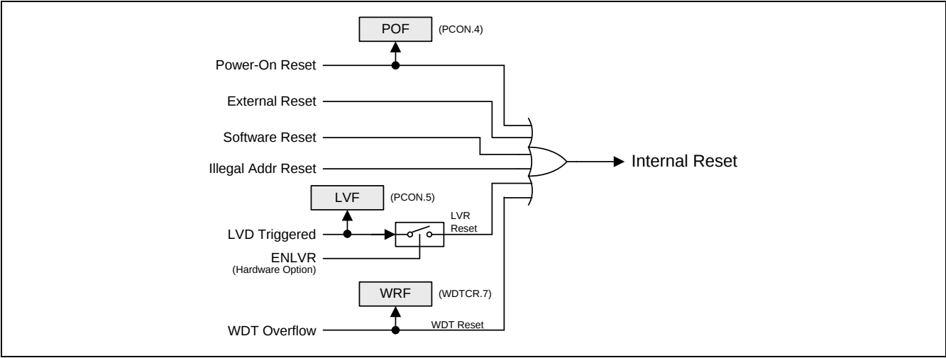
图 10-1. 系统复位源
