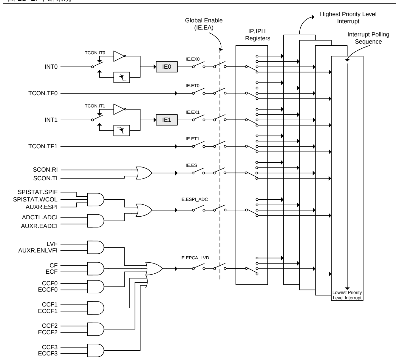
图 13-1. 中断系统
