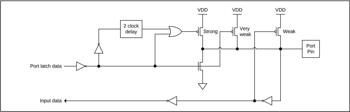
图 12-1. 准双向 I/O
