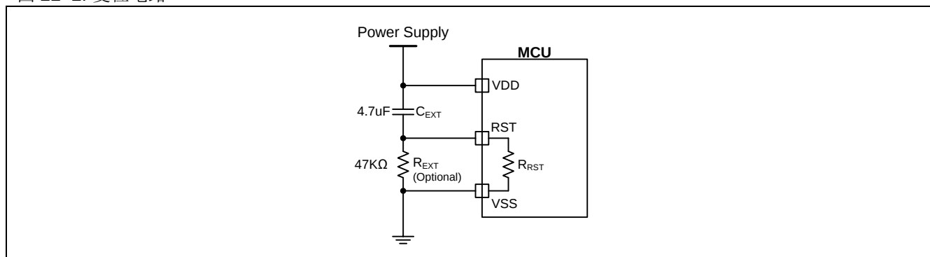
图 22-2. 复位电路
