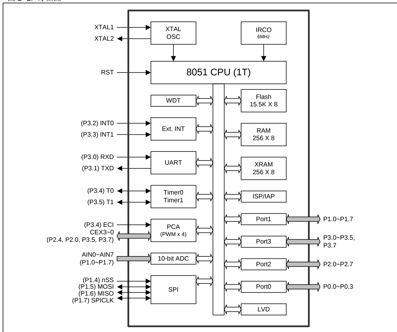
图 2-1. 方框图
