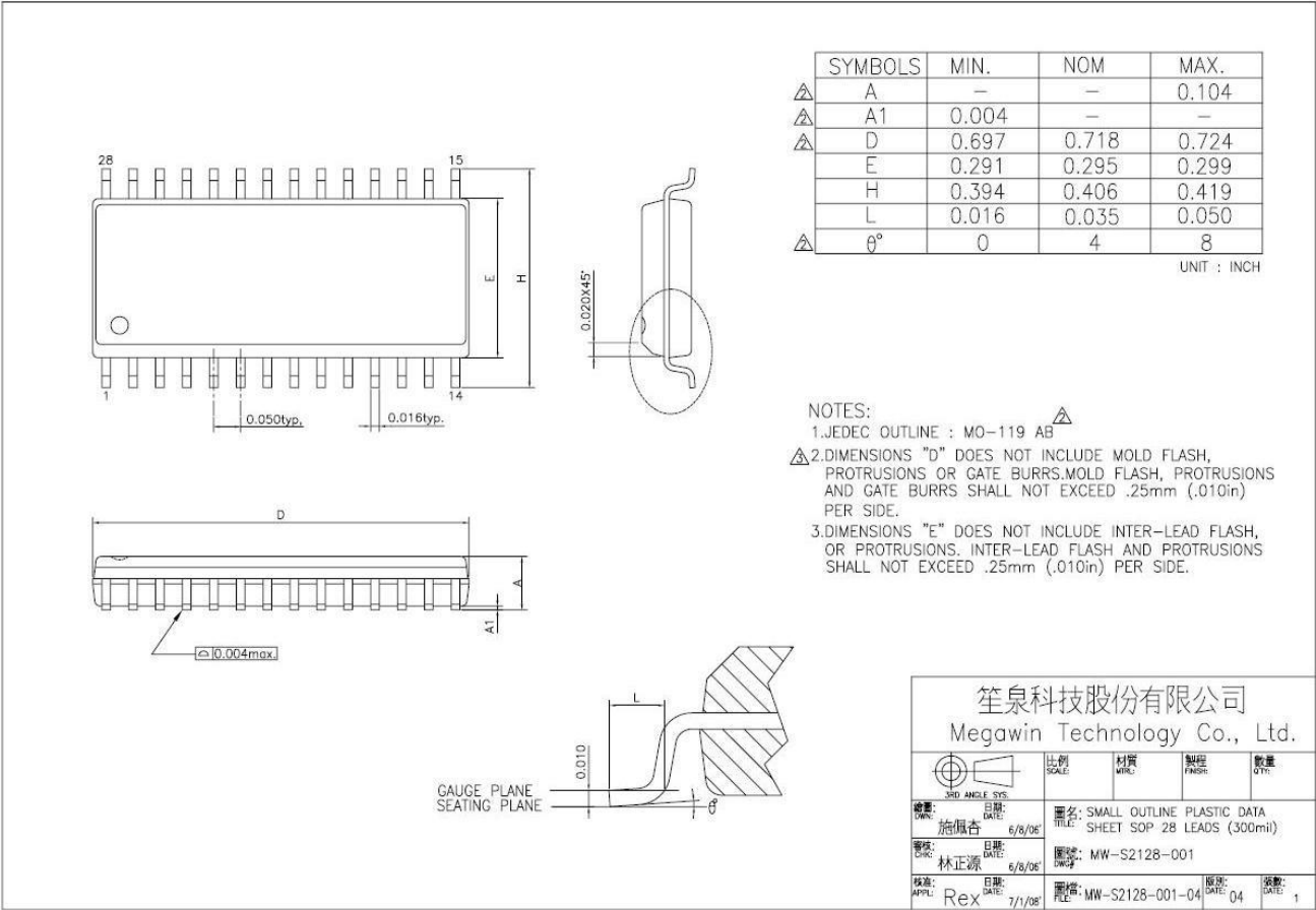
图 25-2. SOP-28
