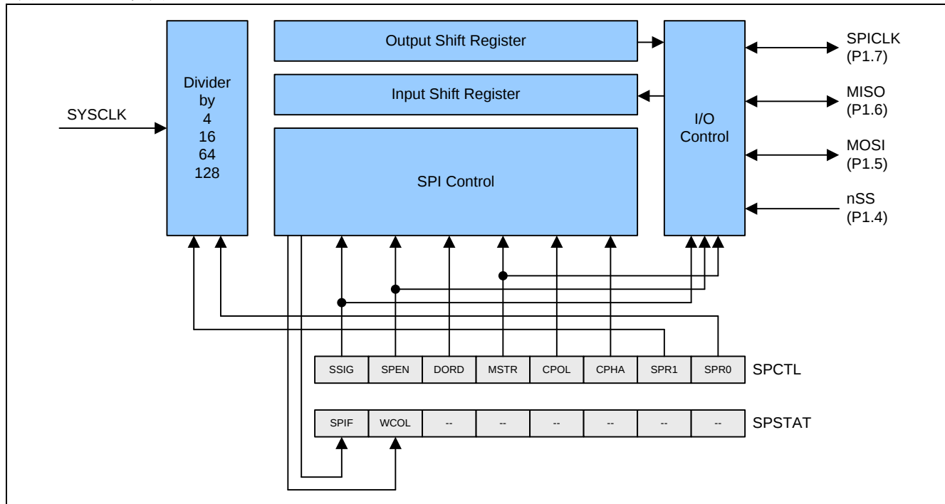
图 17-1. SPI 框图
