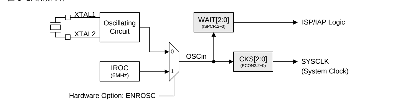
图 8-1. 系统时钟
