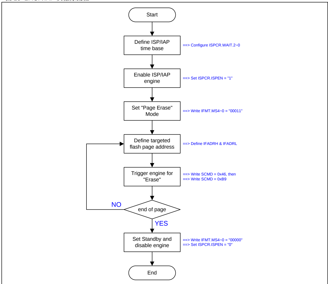
图 19-2. ISP/IAP 页擦除流程
