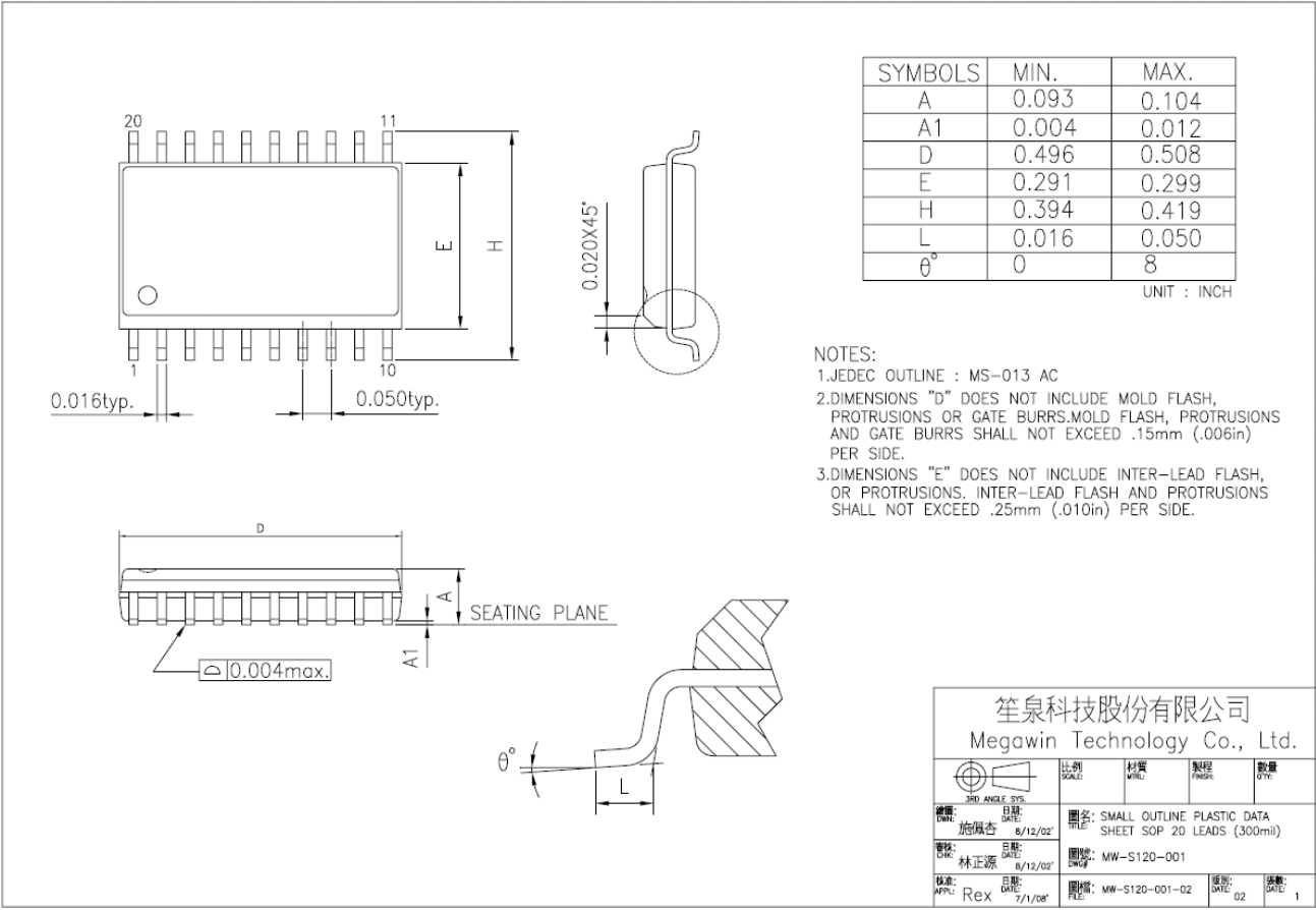
图 25-4. SOP-20
