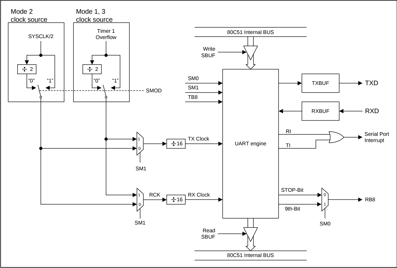
图 15-6. 串行口模式 1, 2, 3
