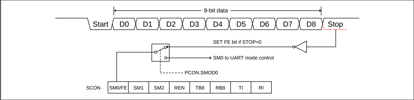
图 15-7. UART 帧错误检测
