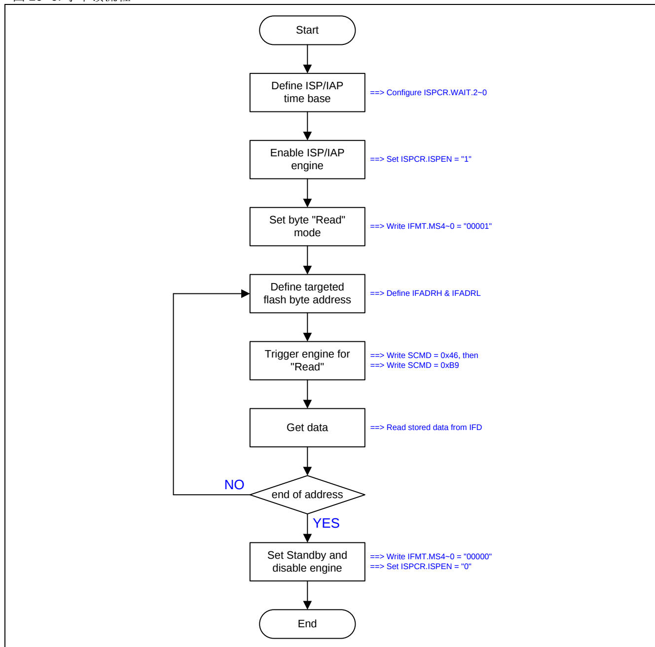
图 19-6. 字节读流程
