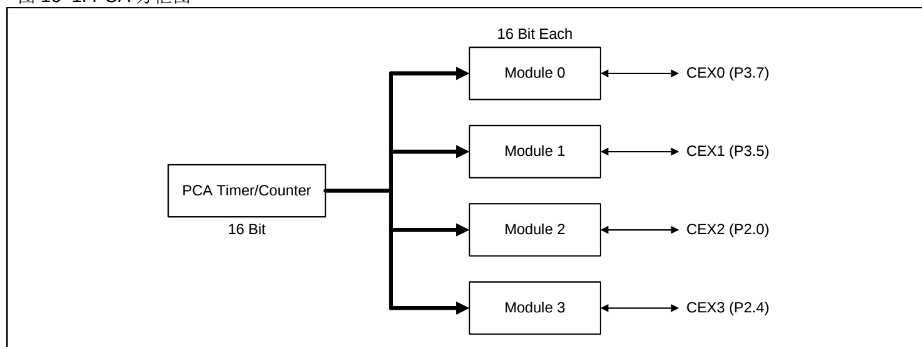
图 16-1. PCA 方框图
