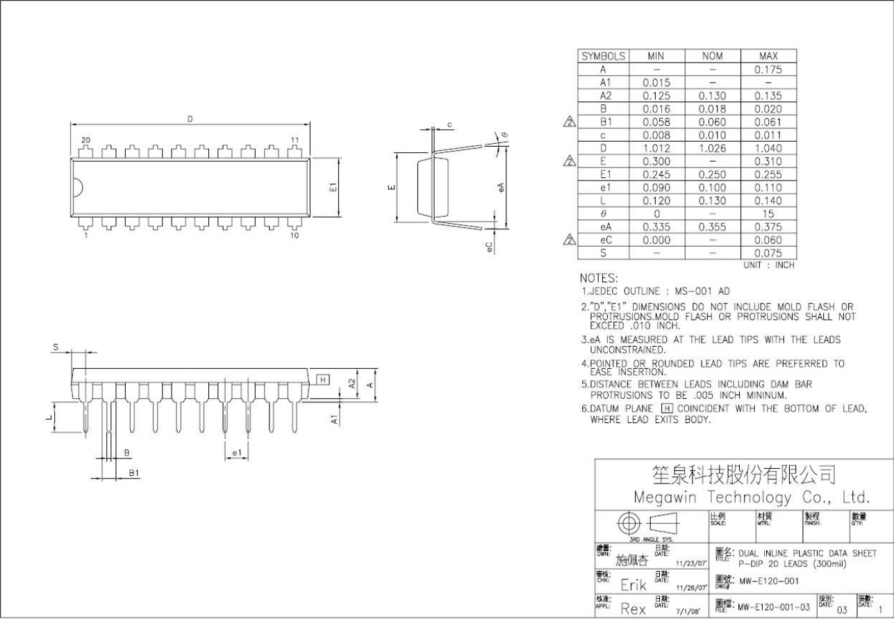
图 25-3. DIP-20
