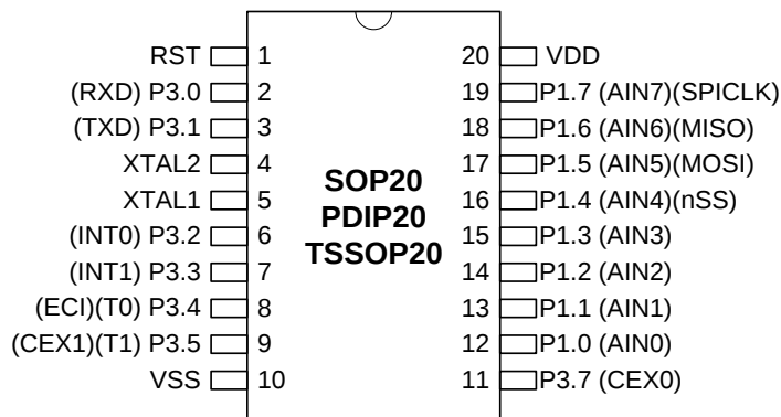
图 4-2. MA803_MA804 20-脚 顶视图
