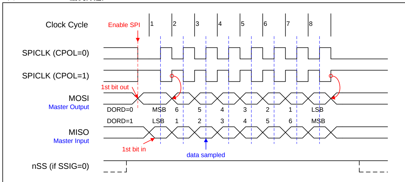
图 17-7. SPI 主机传送, CPHA=0
