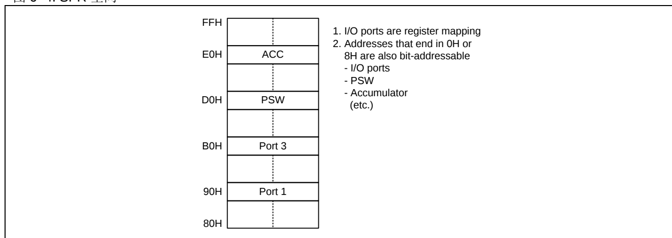
图 6-4. SFR 空间
