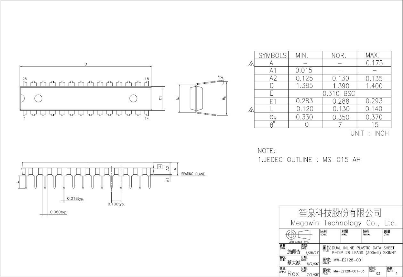
图 25–1. DIP-28
