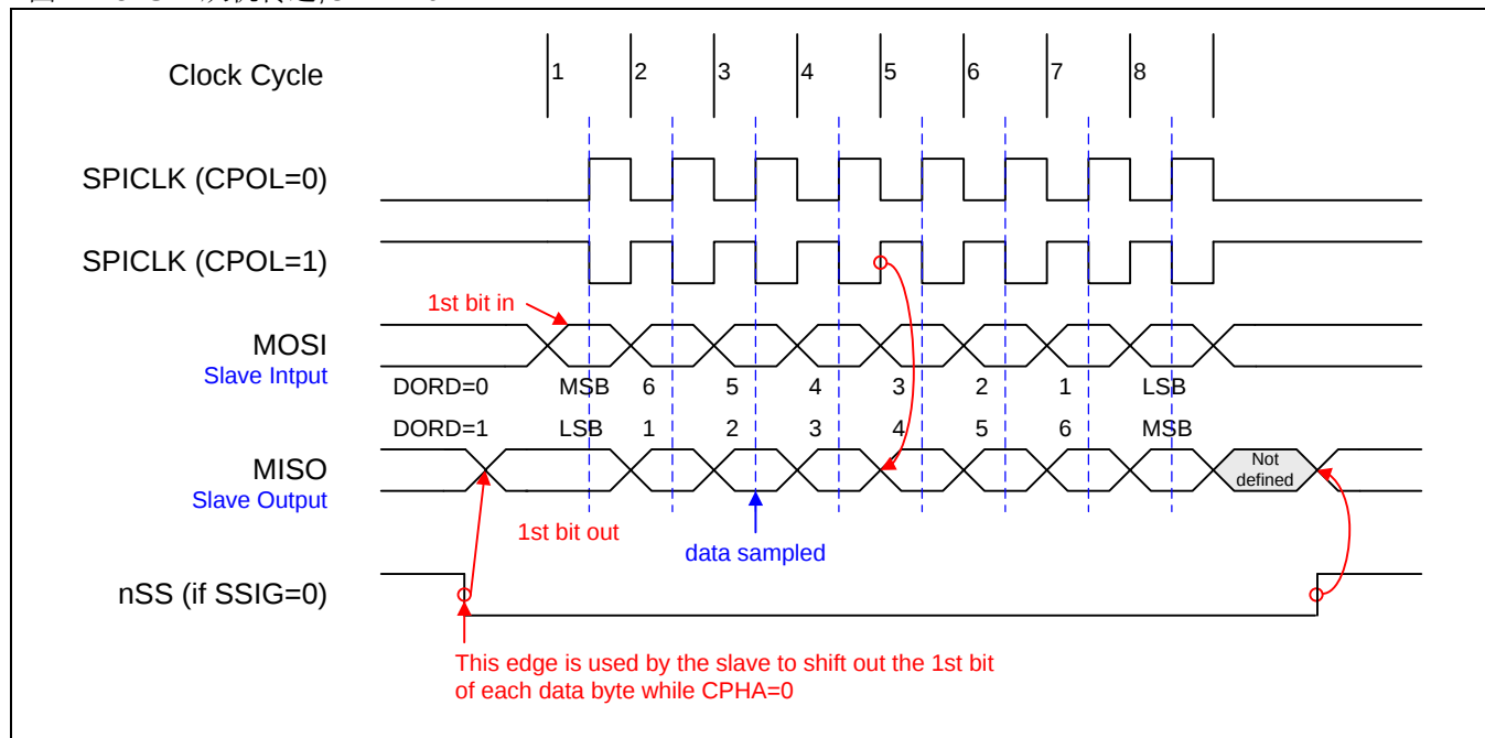
图 17-5. SPI 从机传送,CPHA=0
