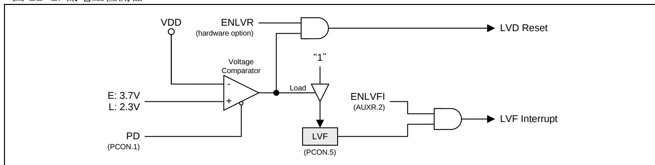
图 11-1. 低电压检测器
