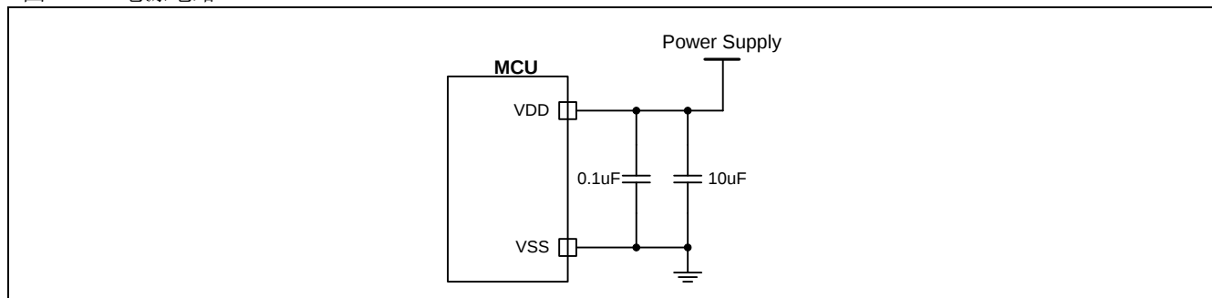
图 22-1. 电源电路
