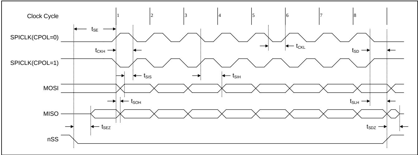
图 23-6. SPI 从机传送时间波形 CPHA=1
