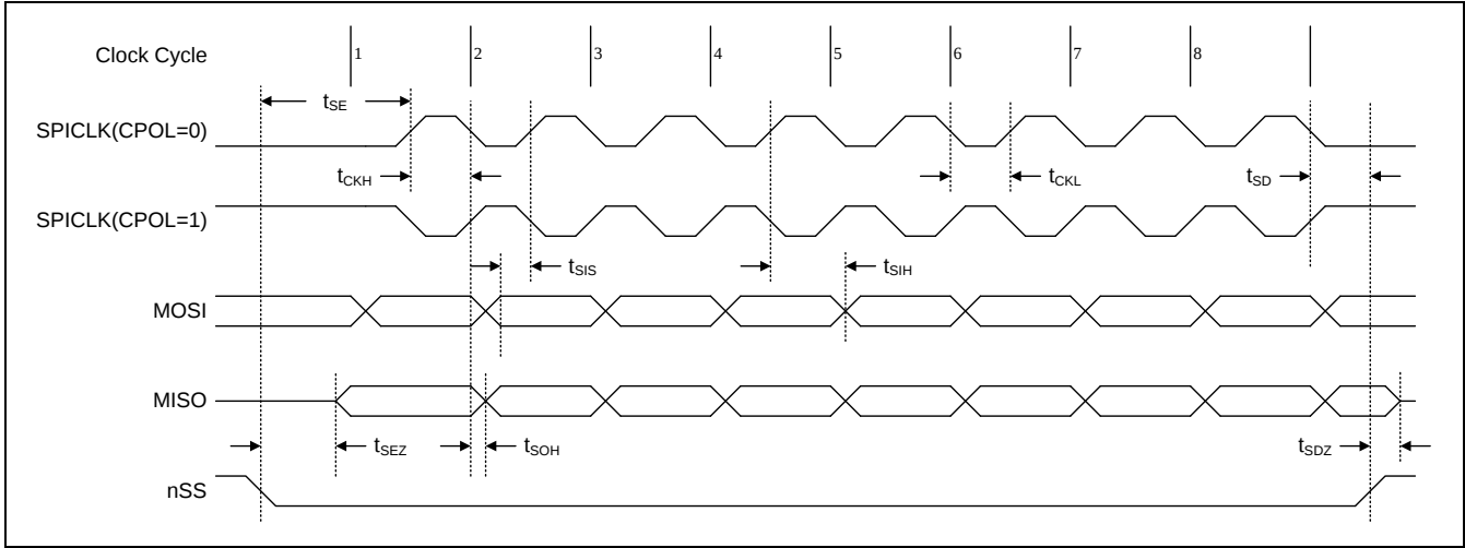
图 23-5. SPI 从机传送时间波形 CPHA=0
