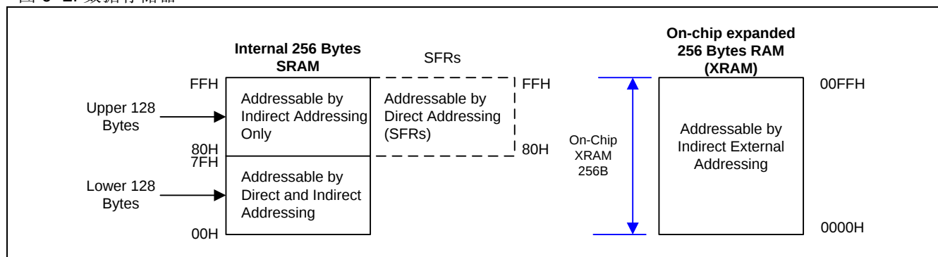
图 6-2. 数据存储器
