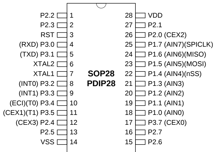
图 4-1. MA803_MA804 28-脚 顶视图
