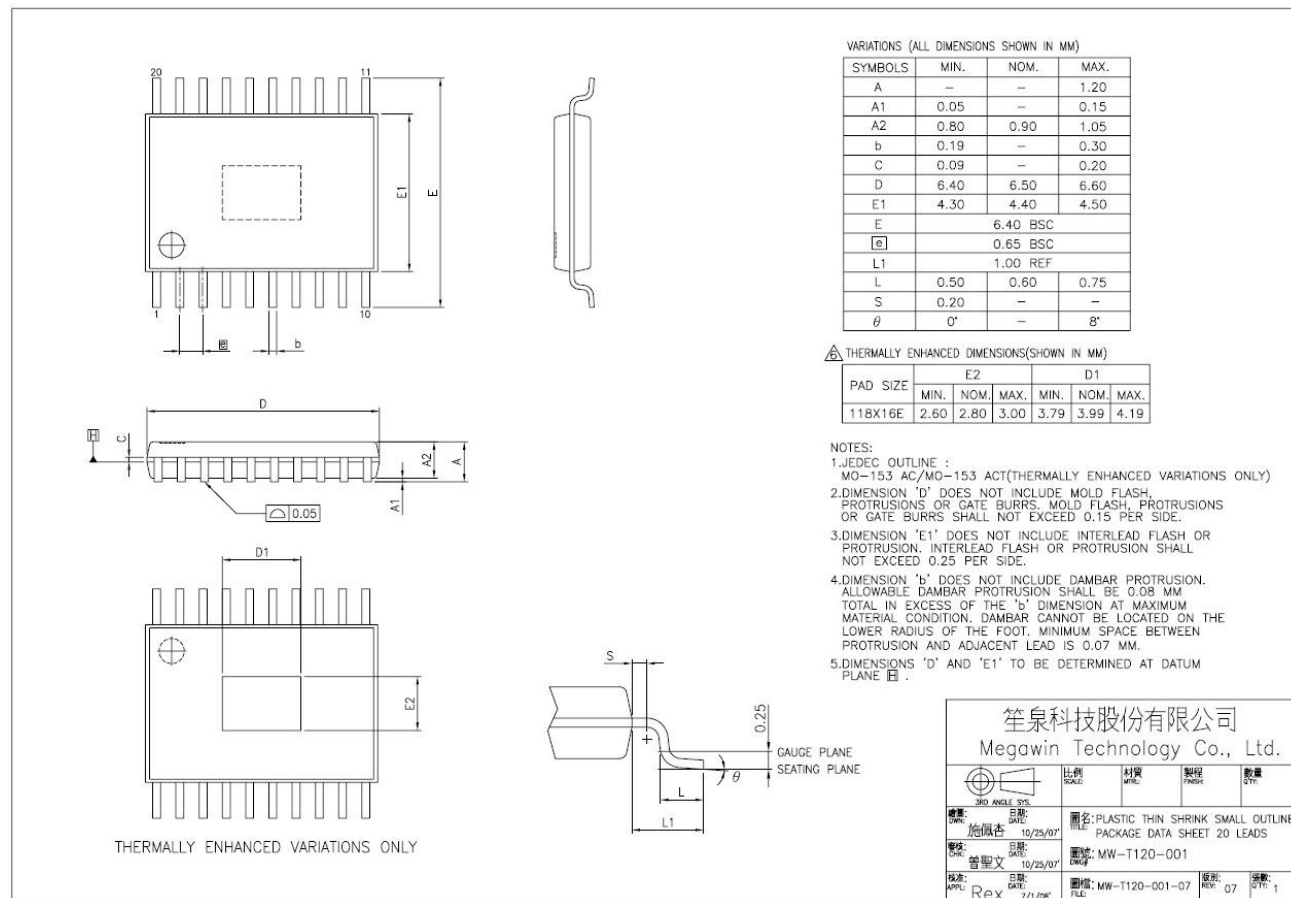
图 25-3. TSSOP-20
