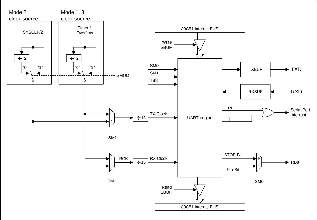
图 15-6. 串行口模式 1, 2, 3
