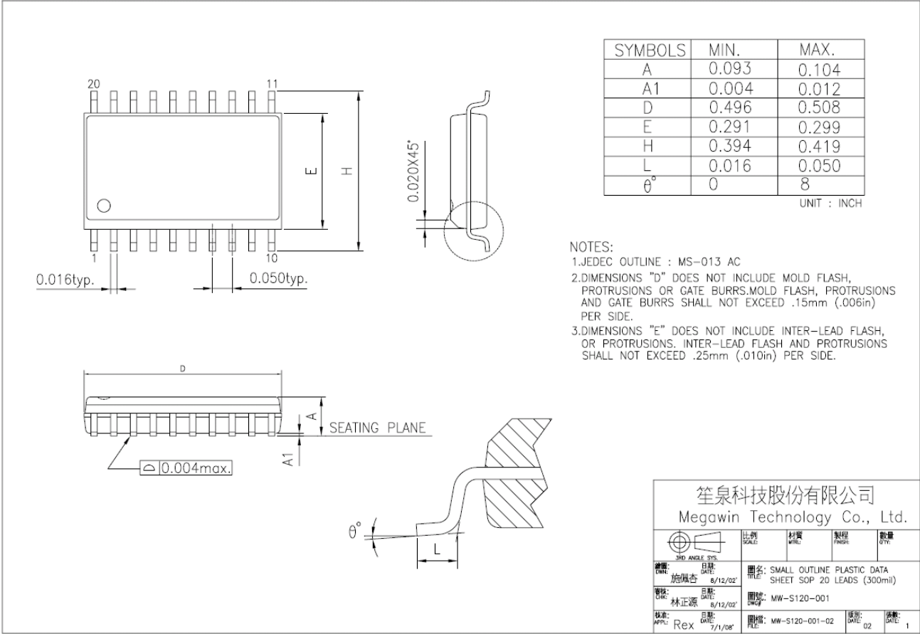
图 25-2. SOP-20
