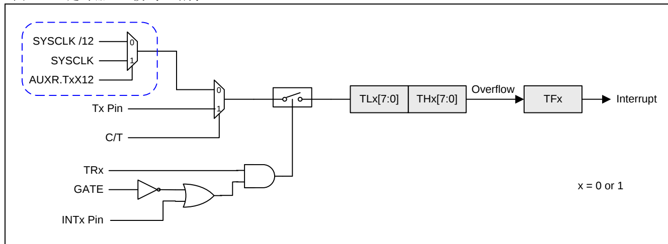
图 14-2. 定时器 0/1 模式 1 结构
