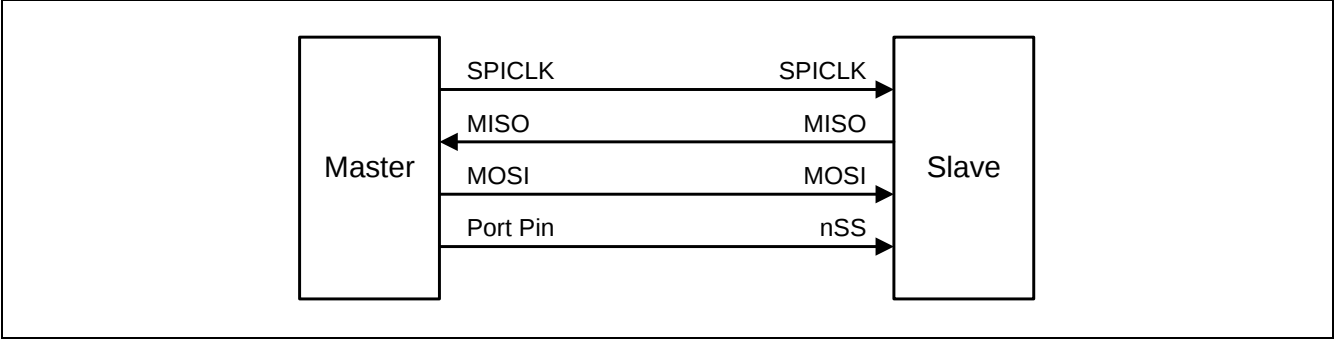
图 17-2. SPI 单主从机配置
