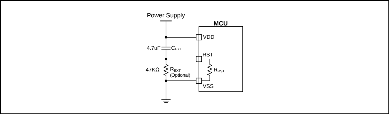
图 22-2. 复位电路
