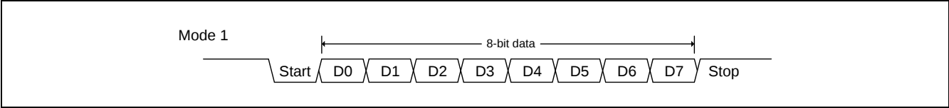
图 15-1. 模式 1 数据帧
