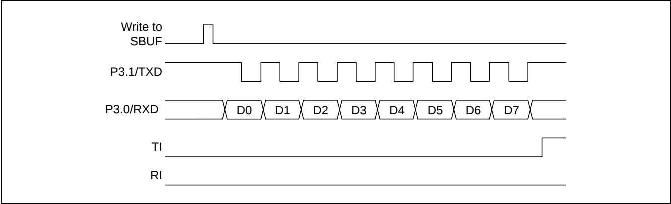
图 15-4. 模式 0 传送波形
