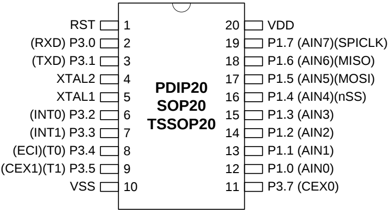
图 4–1. MA801_ MA802 20 脚 顶视图
