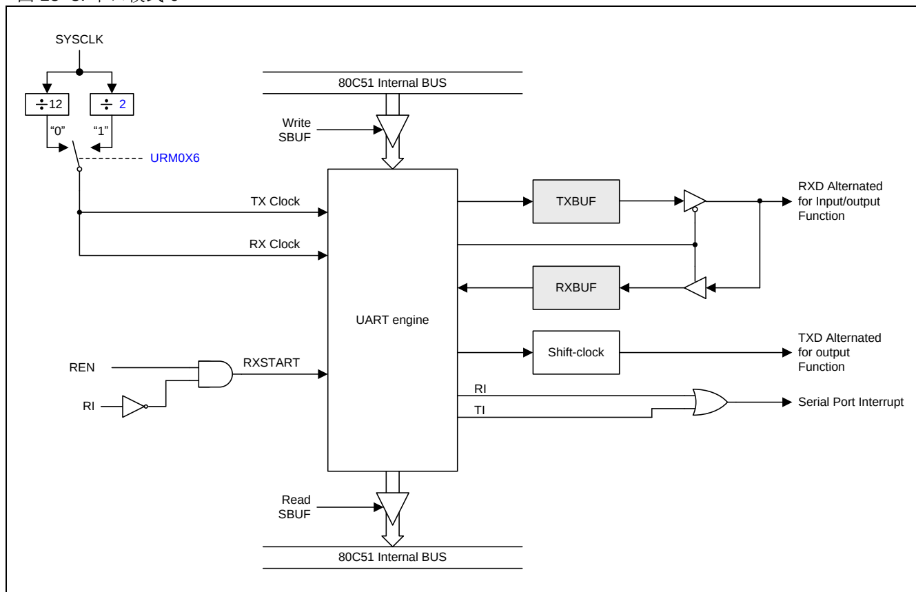
图 15-3. 串口模式 0
