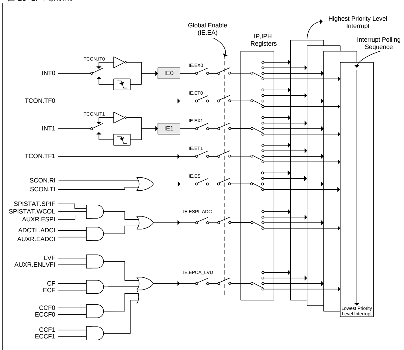
图 13-1. 中断系统
