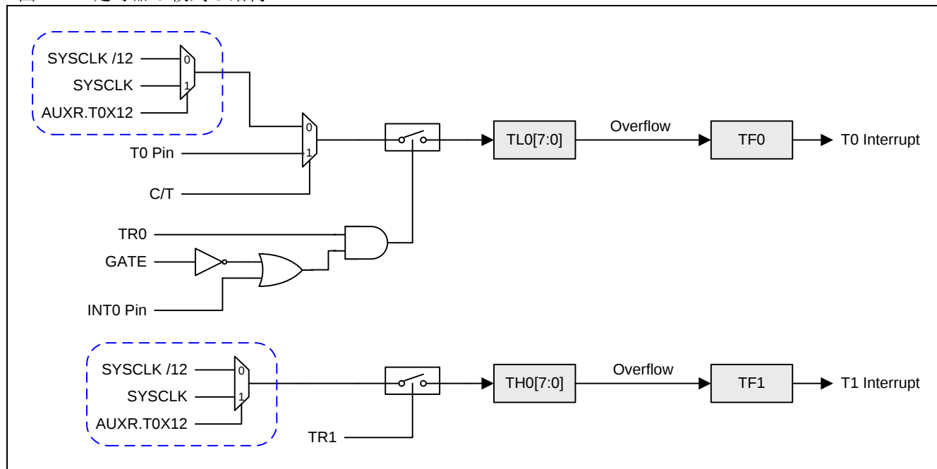
图 14-4. 定时器 0 模式 3 结构
