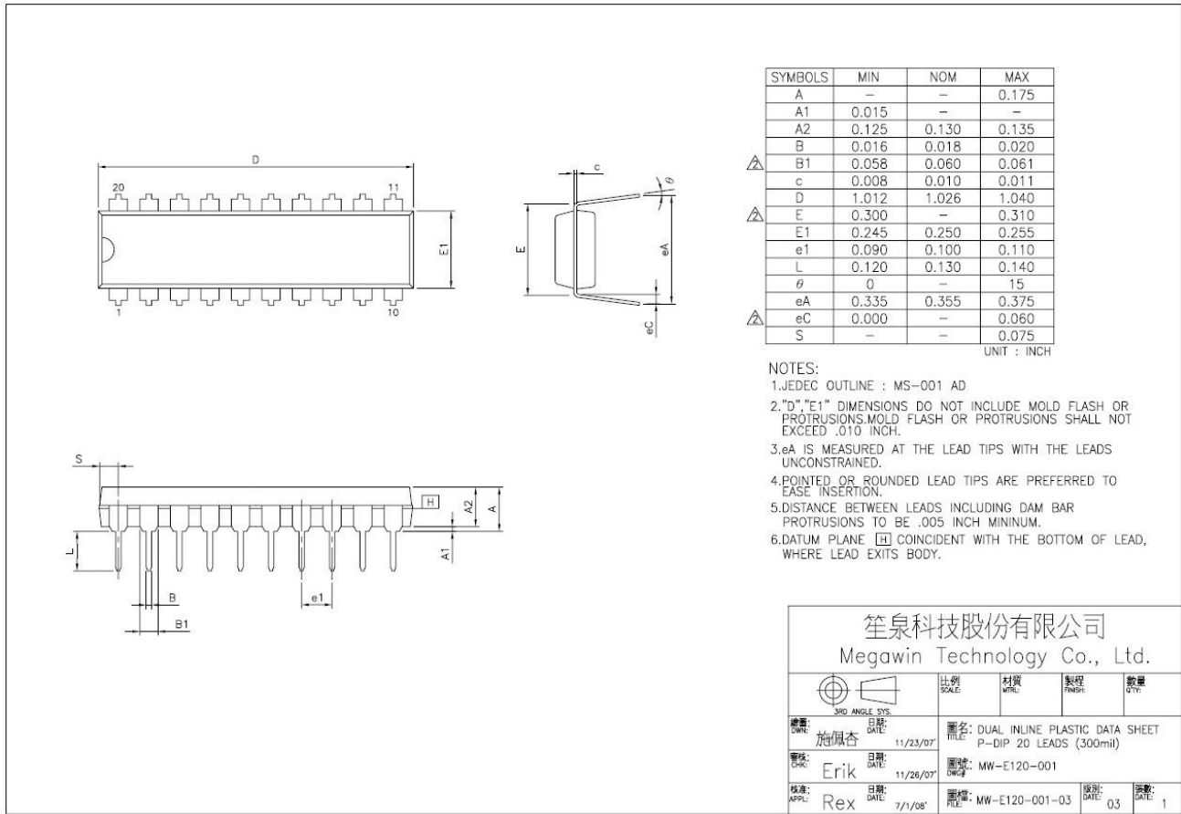
图 25-1. DIP-20
