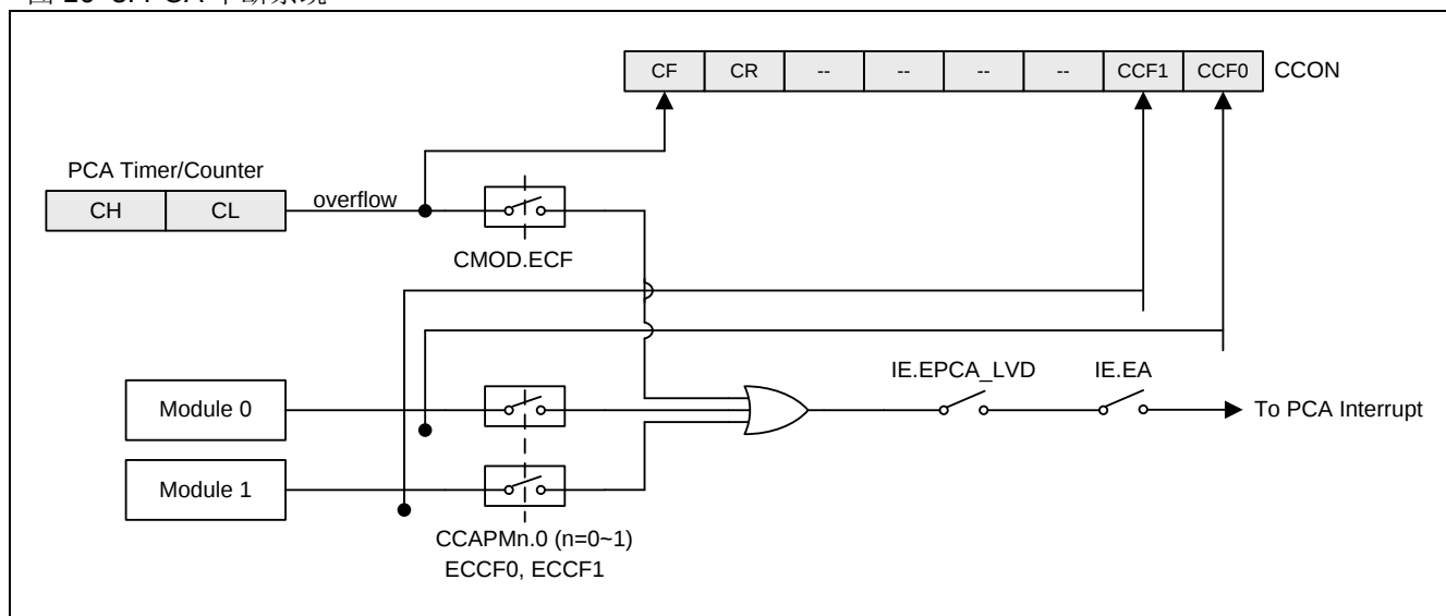
图 16-3. PCA 中断系统
