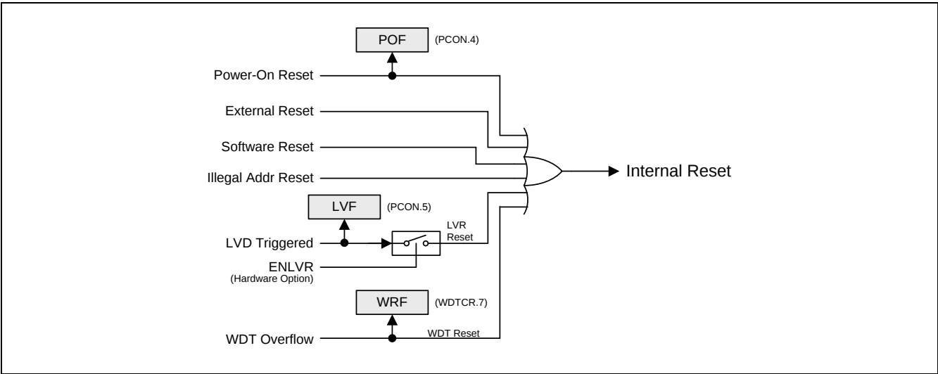
图 10-1. 系统复位源
