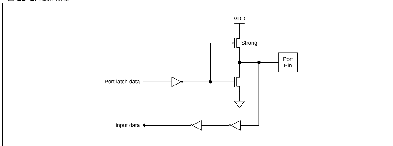
图 12-2. 推挽输出
