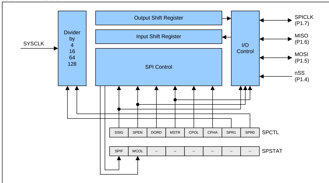
图 17-1. SPI 框图
