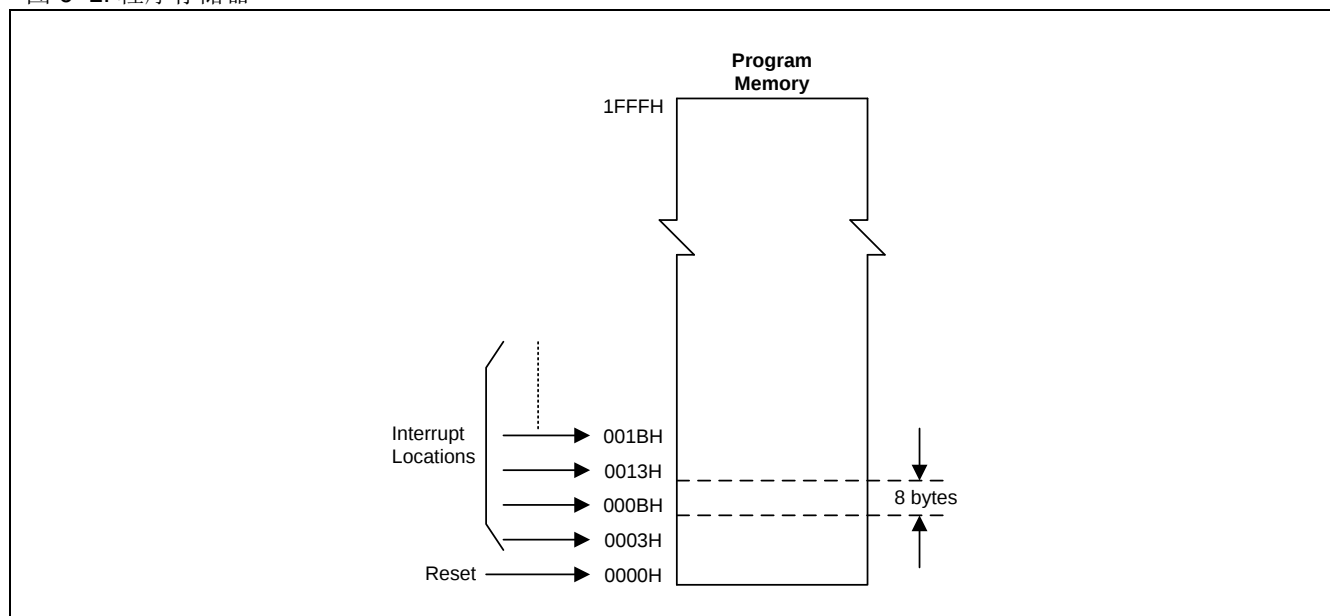
图 6-1. 程序存储器
