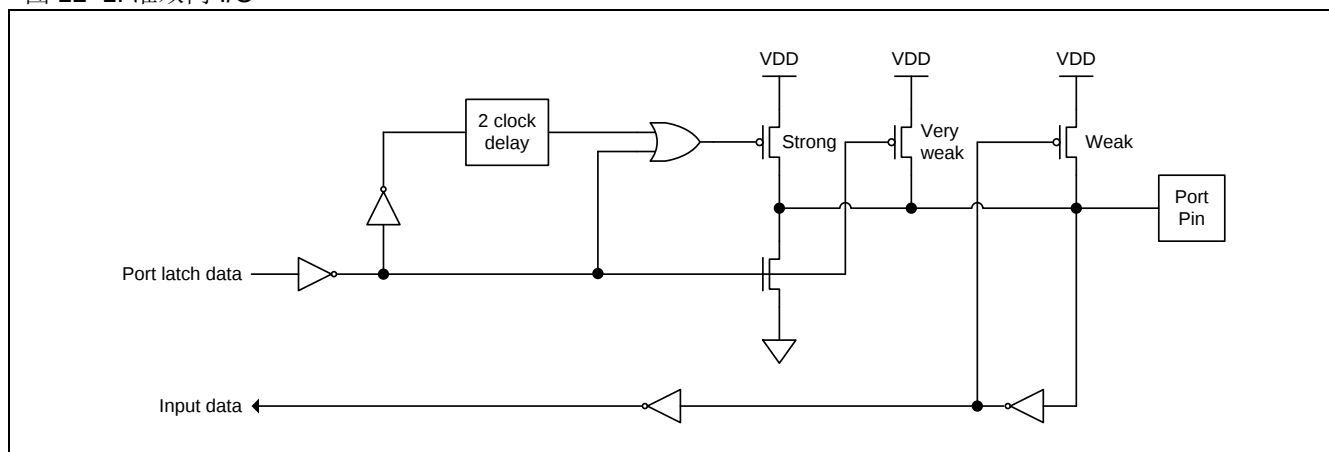
图 12-1. 准双向 I/O
