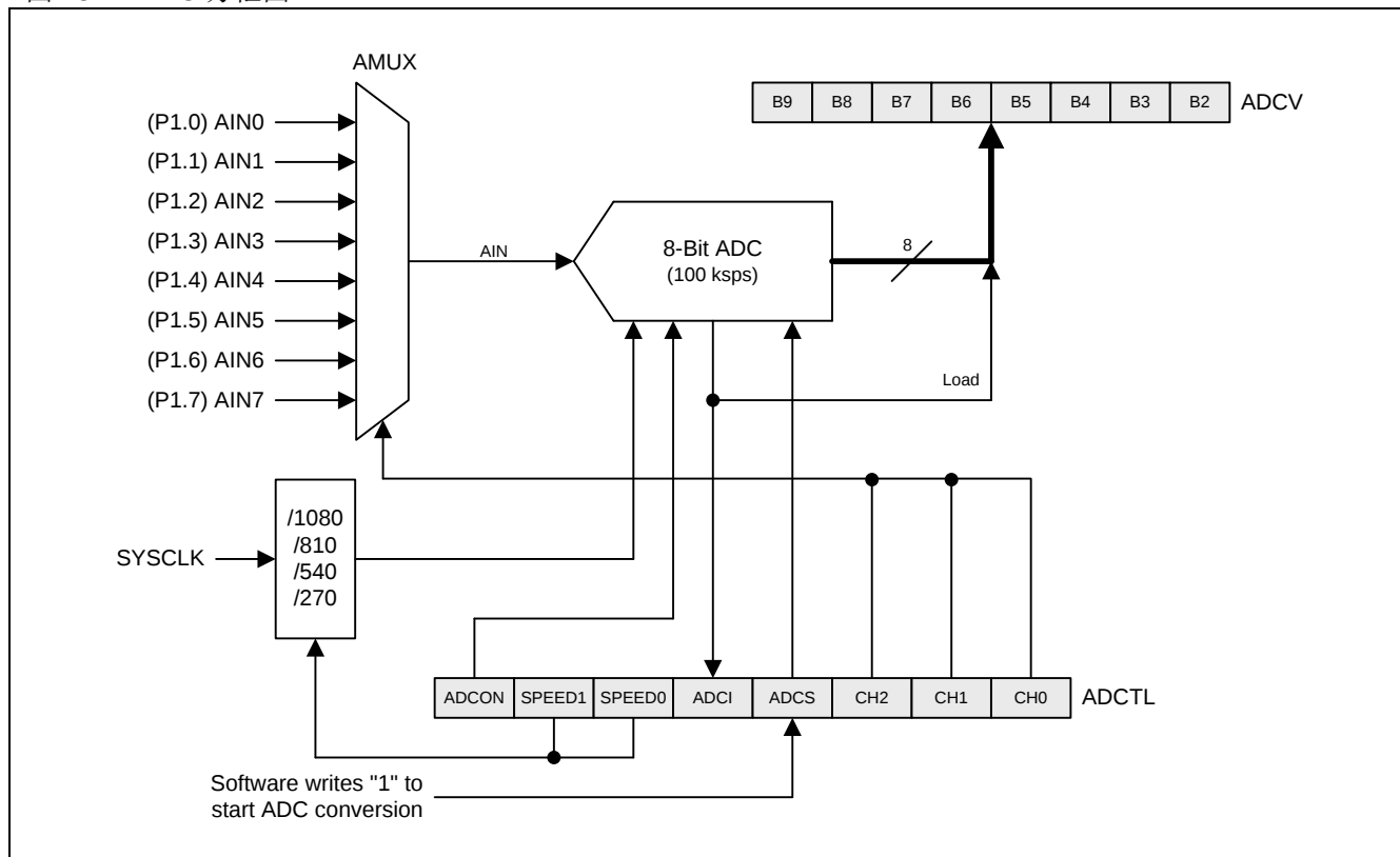
图 18-1. ADC 方框图
