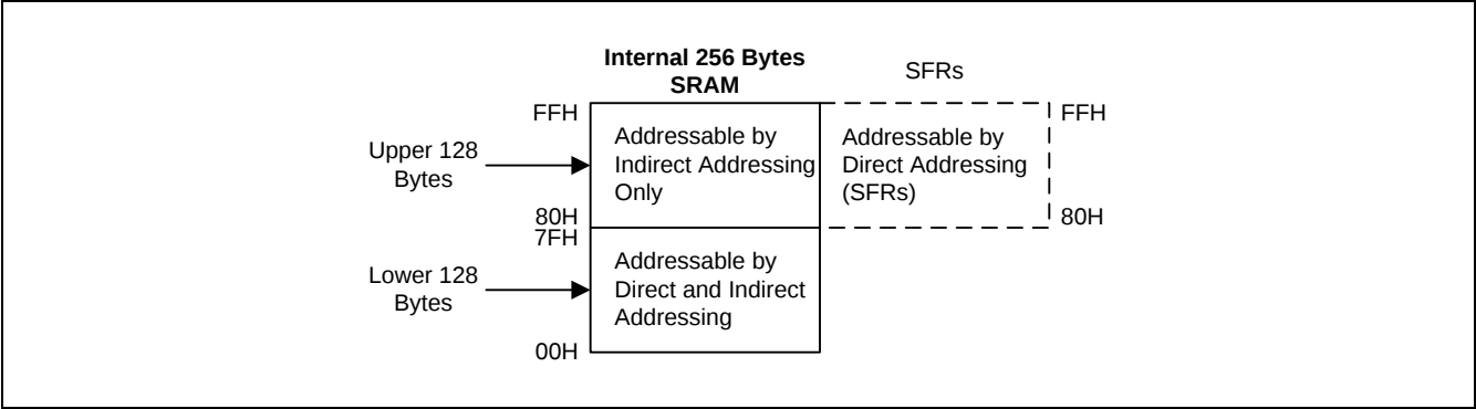
图 6-2. 数据存储器
