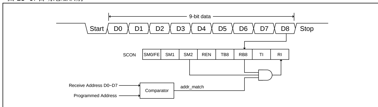
图 15-9. 自动地址识别
